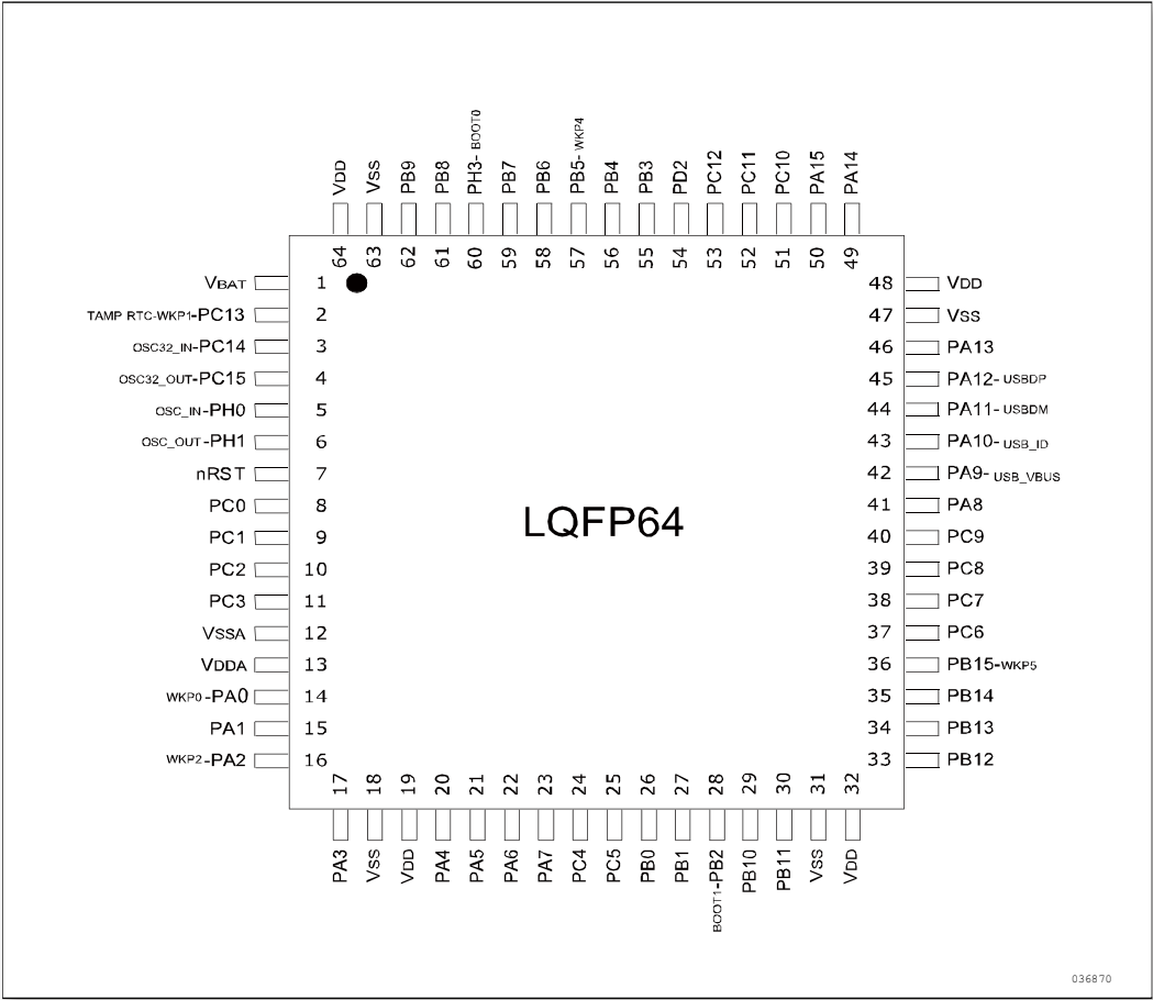
图 3-3 LQFP64 引脚分布
