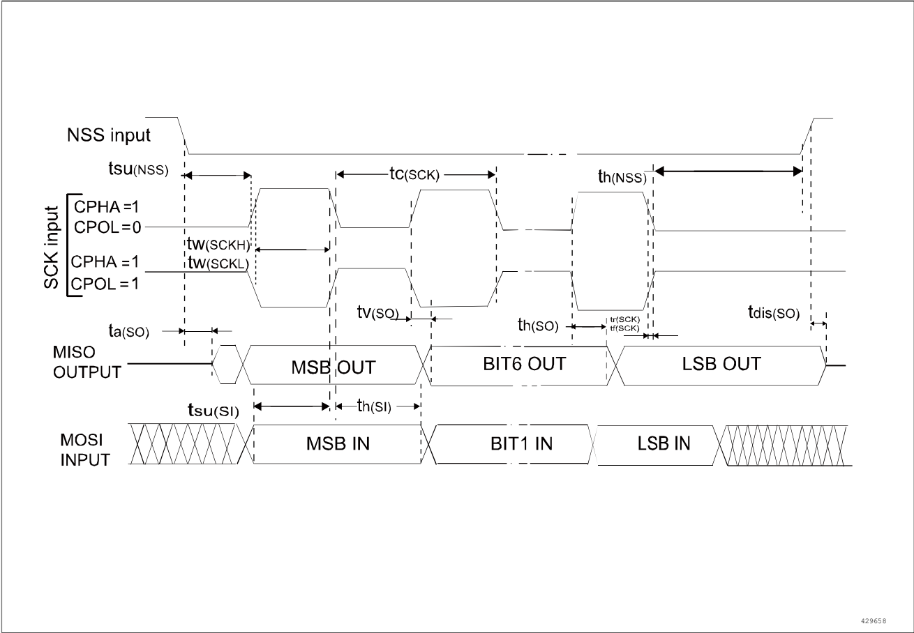
图 4-16 SPI 时序图-从模式和 CPHA = 1，CPHASEL = 1 (1)
