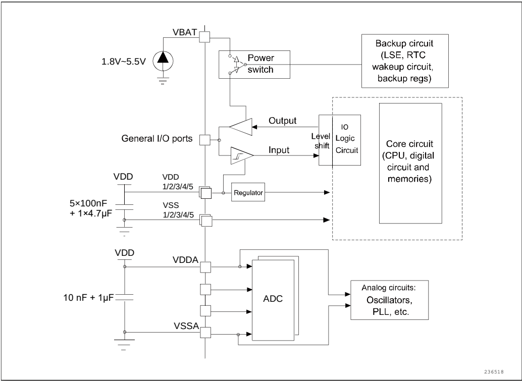
图 4-3 供电方案
