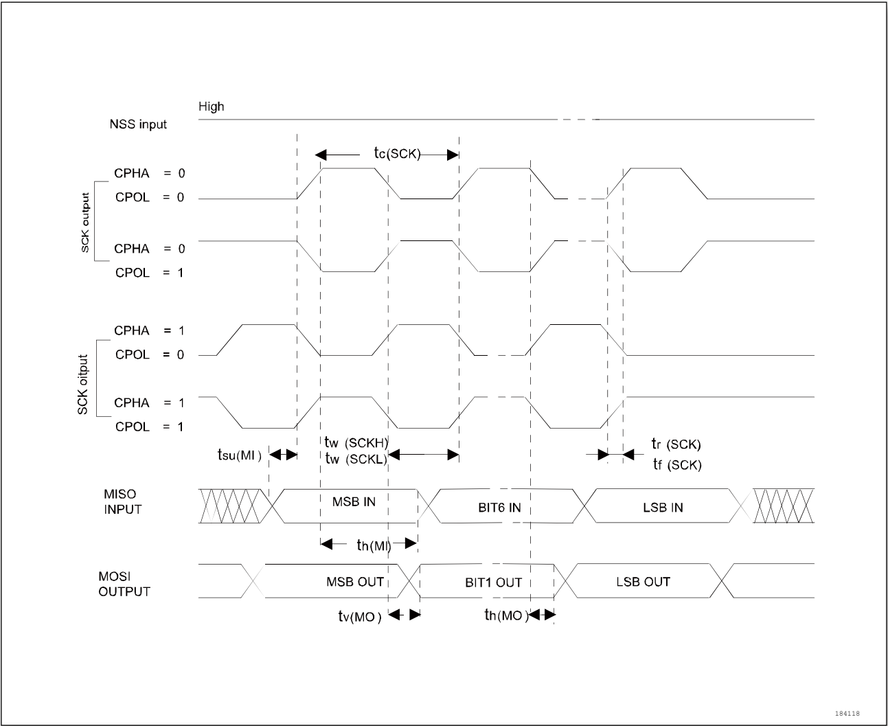
图 4-17 SPI 时序图-主模式，CPHASEL = 1 (1)
