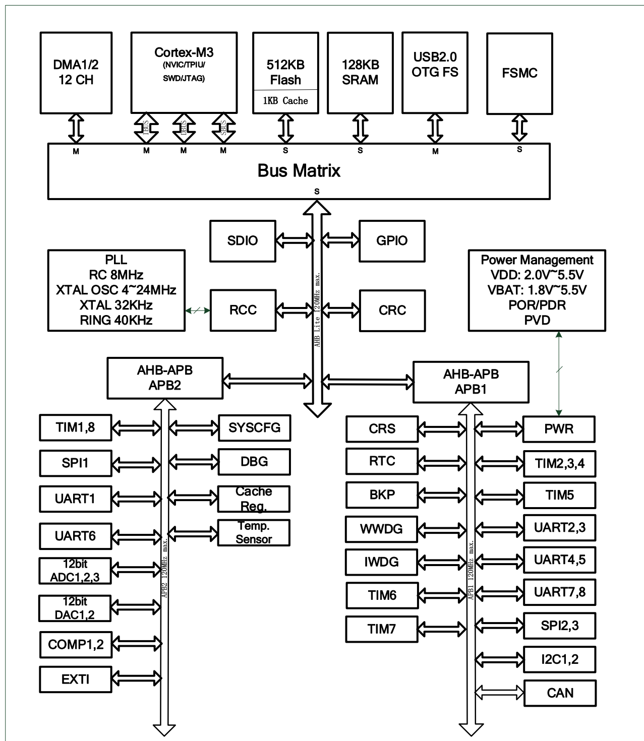
图 2-2 模块框图
