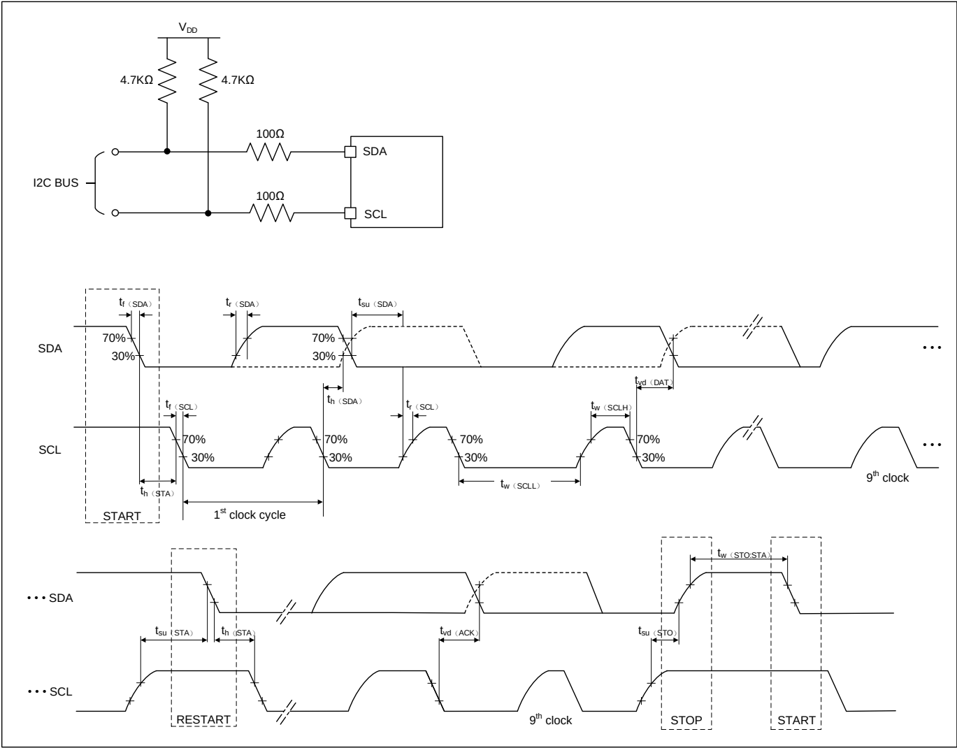
图 4-14 I2C 总线交流波形和测量电路 (1)
