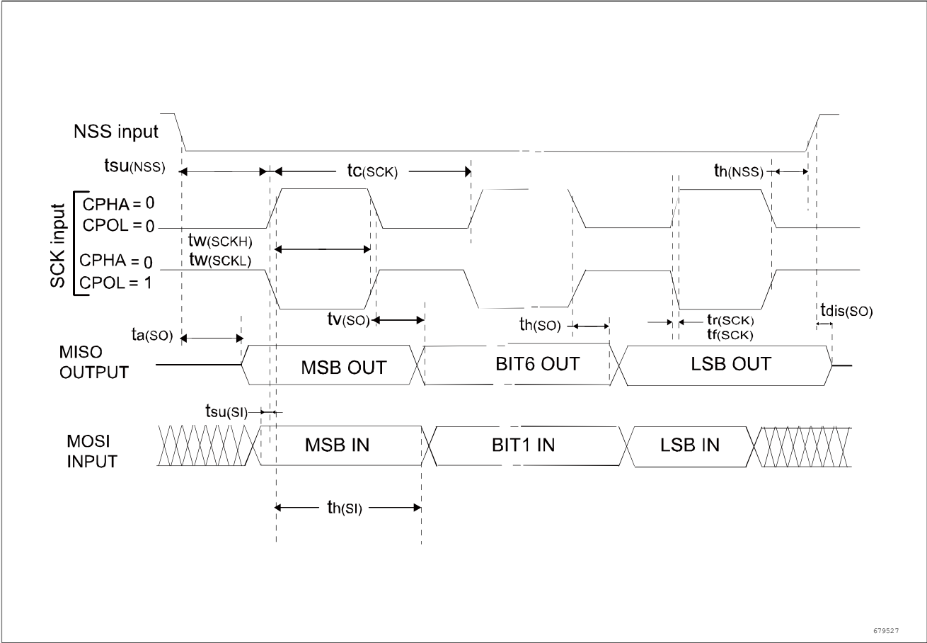
图 4-15 SPI 时序图-从模式和 CPHA = 0, CPOL = 1
