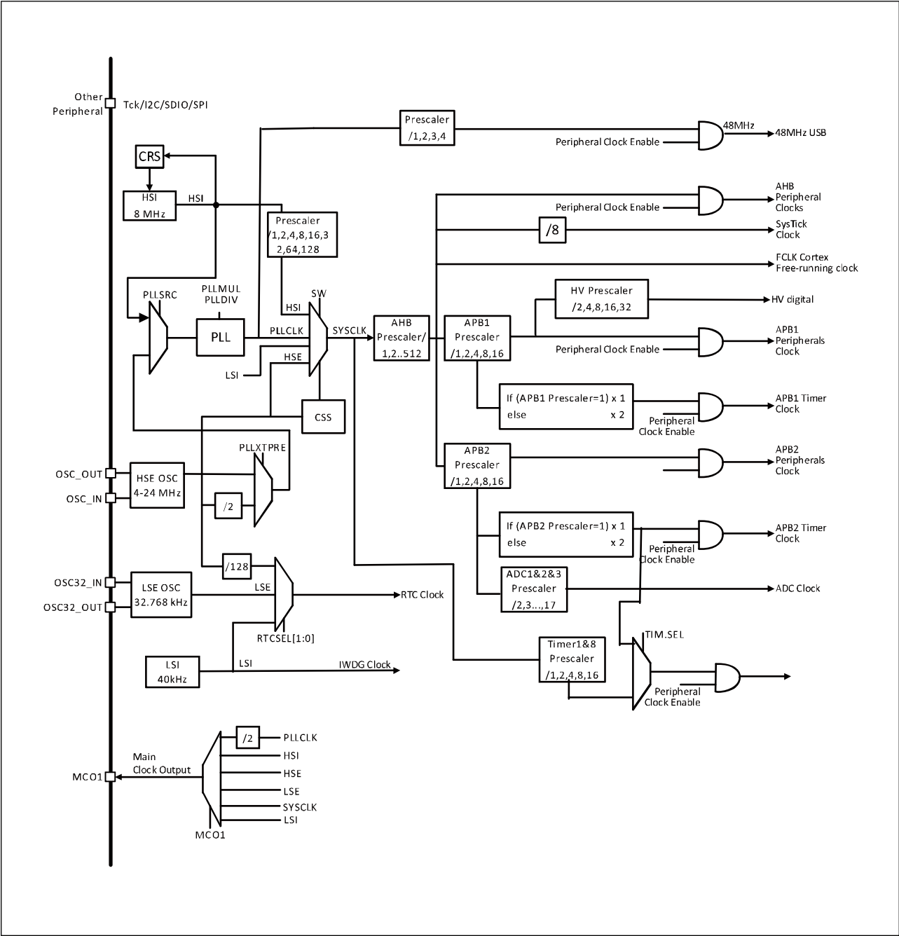
图 2-3 时钟树
