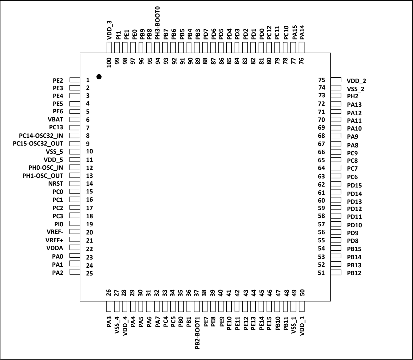
图 4-2 LQFP100 引脚分布
