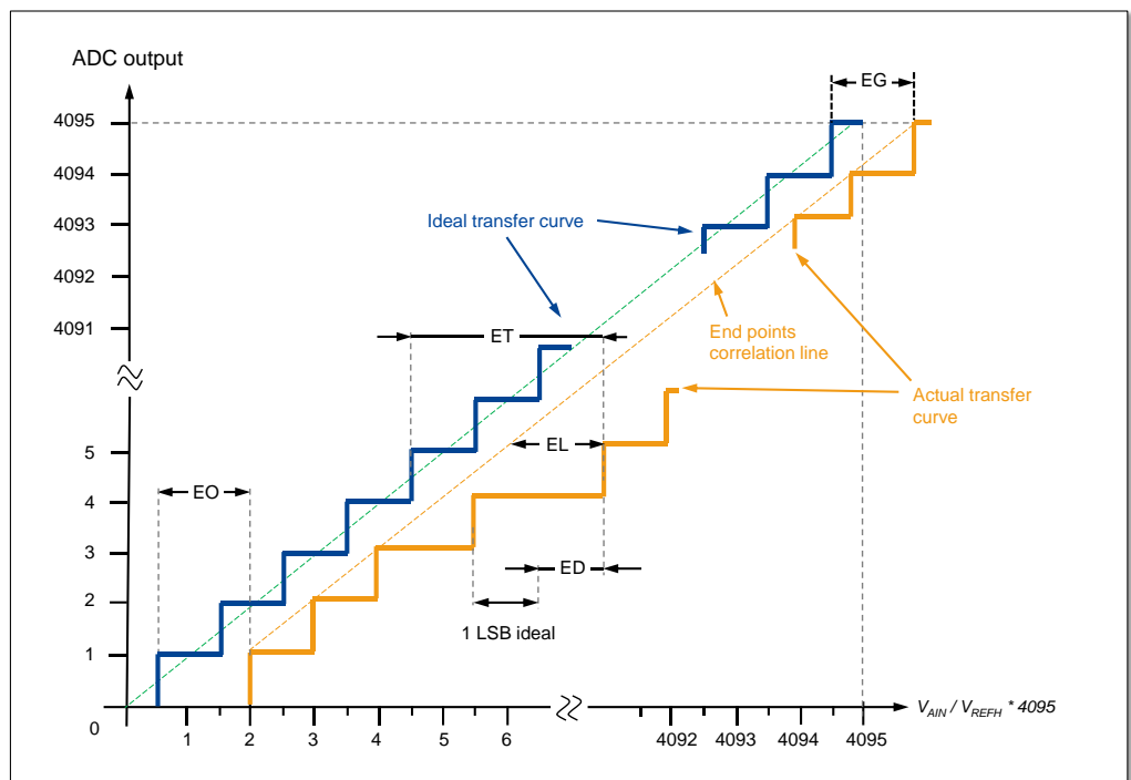
图 5-12 ADC 静态参数示意图
