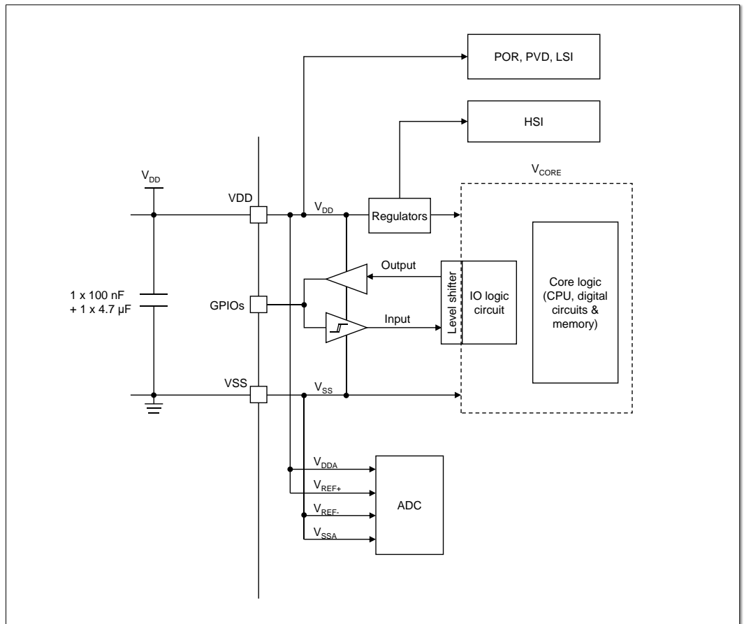
图 5-3 供电方案
