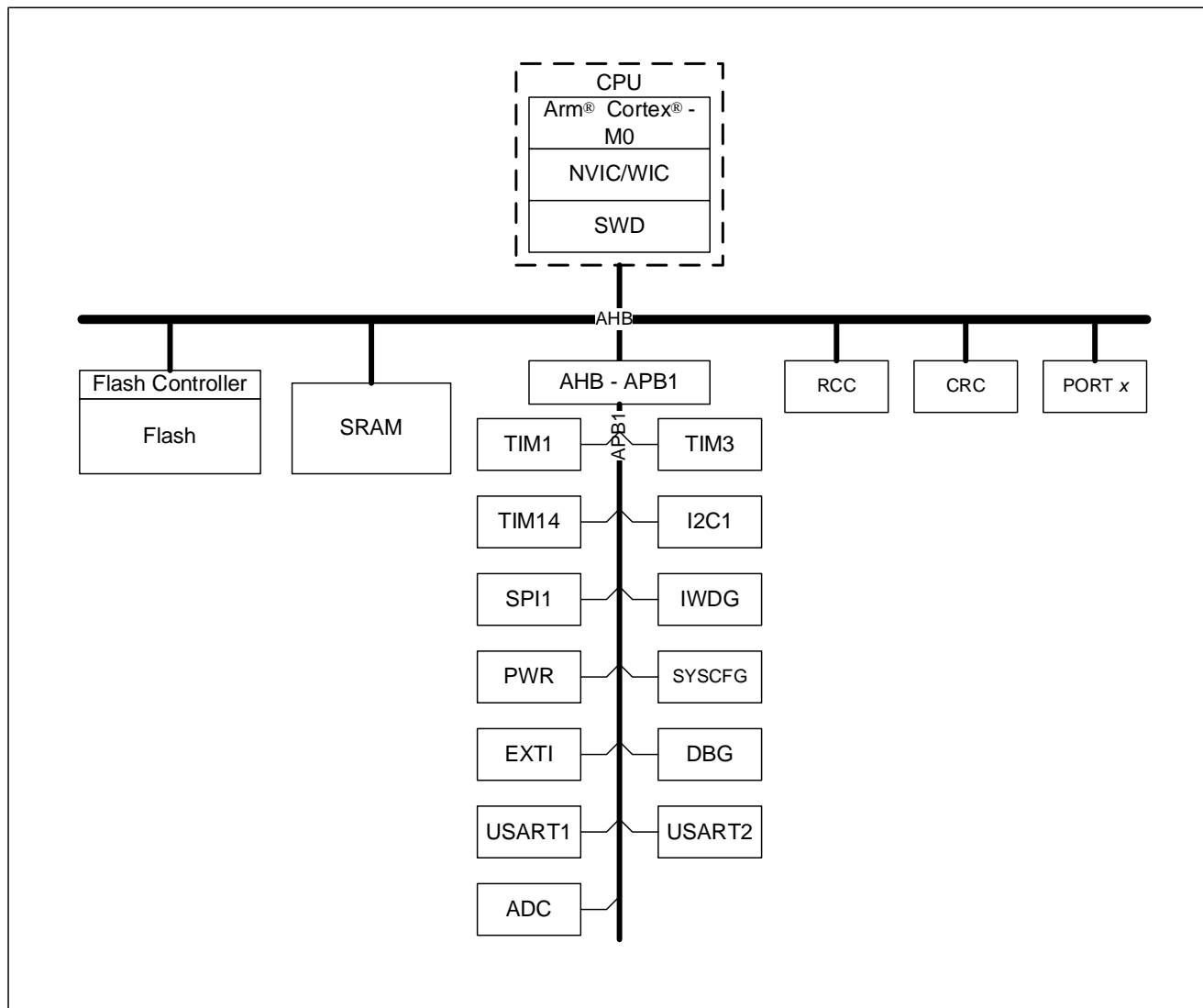
图 3-1 系统框图
