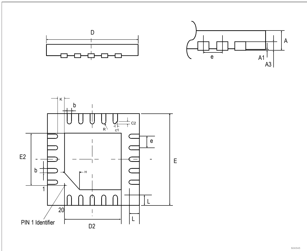
图 6-1 QFN20 封装尺寸
