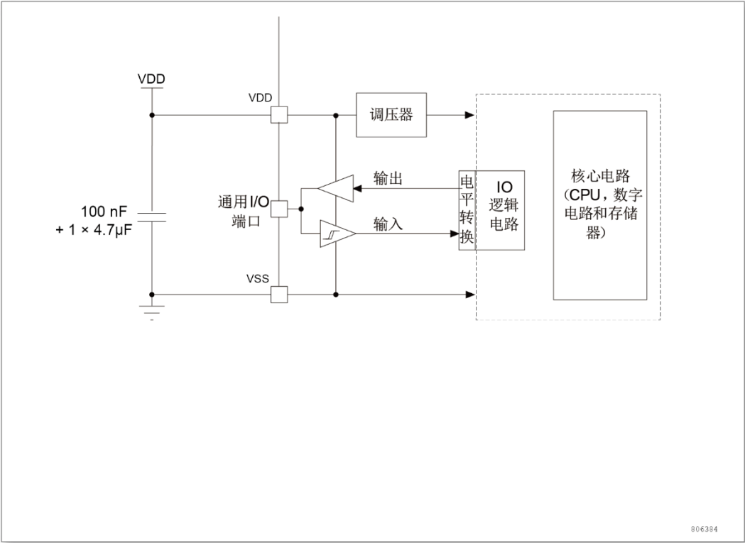
图 10 供电方案
