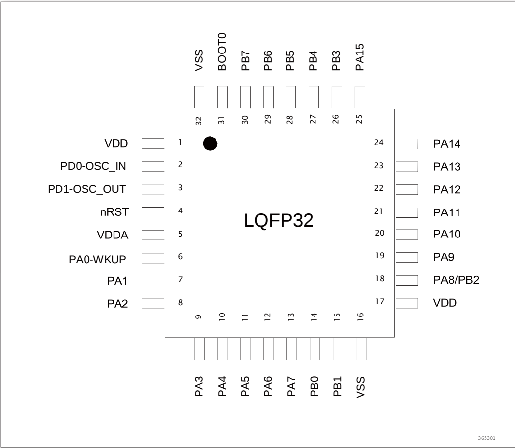
图 7. LQFP32 引脚分布
