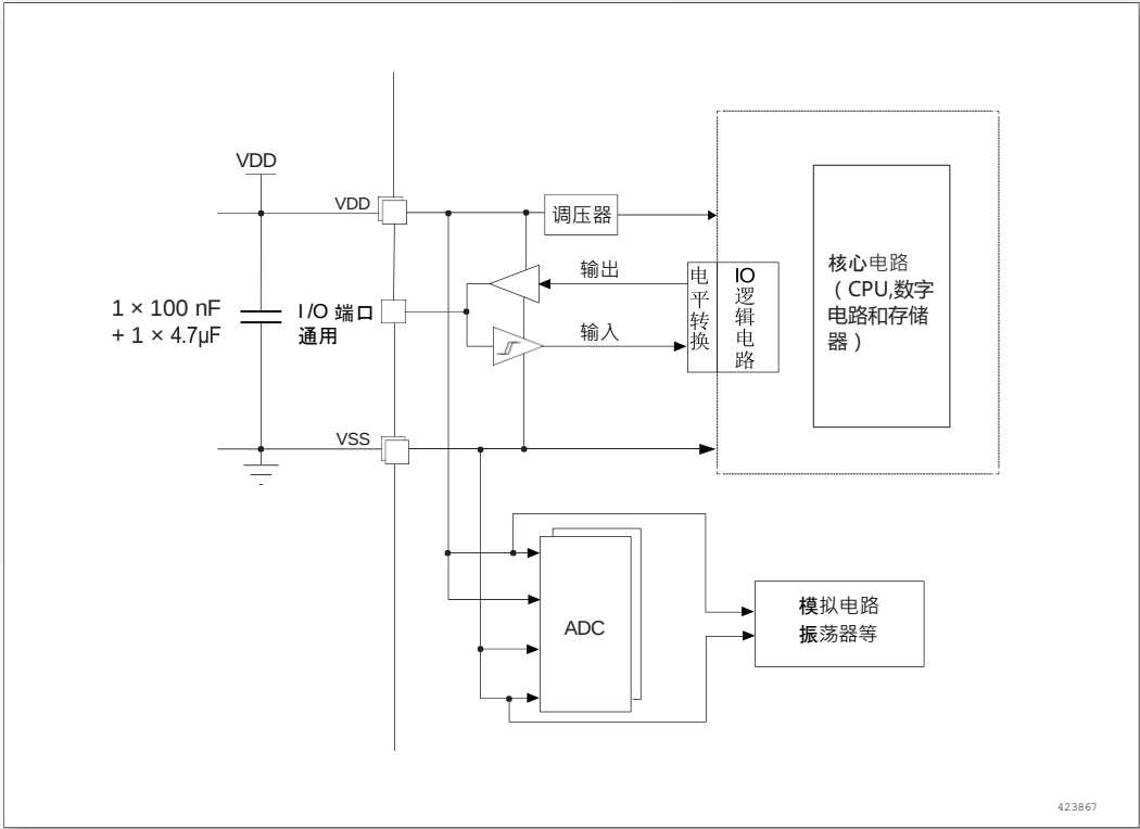
图 12. 供电方案
