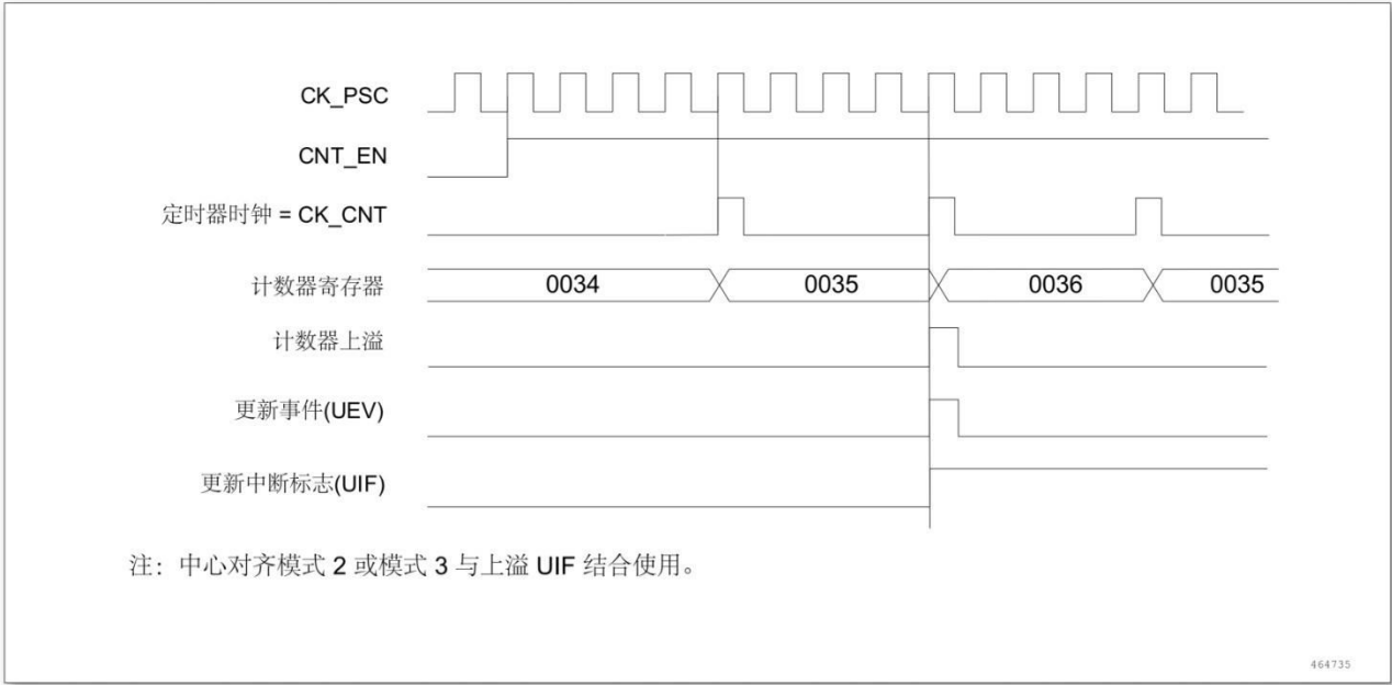
图 12-17 计数器时序图，内部时钟分频因子为 4，TIMx_ARR = 0x03
