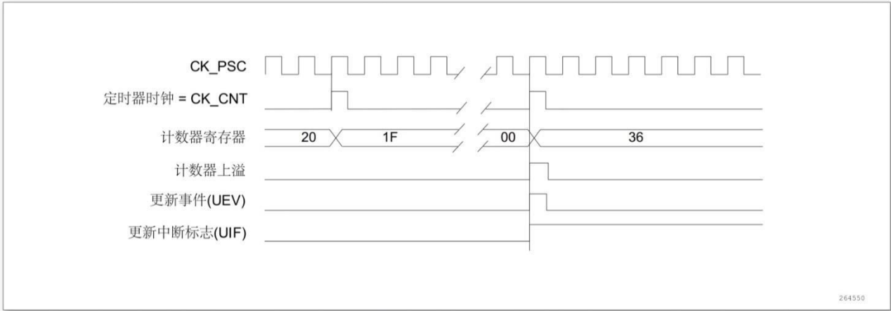
图 12-13 计数器时序图，内部时钟分频因子为 N
