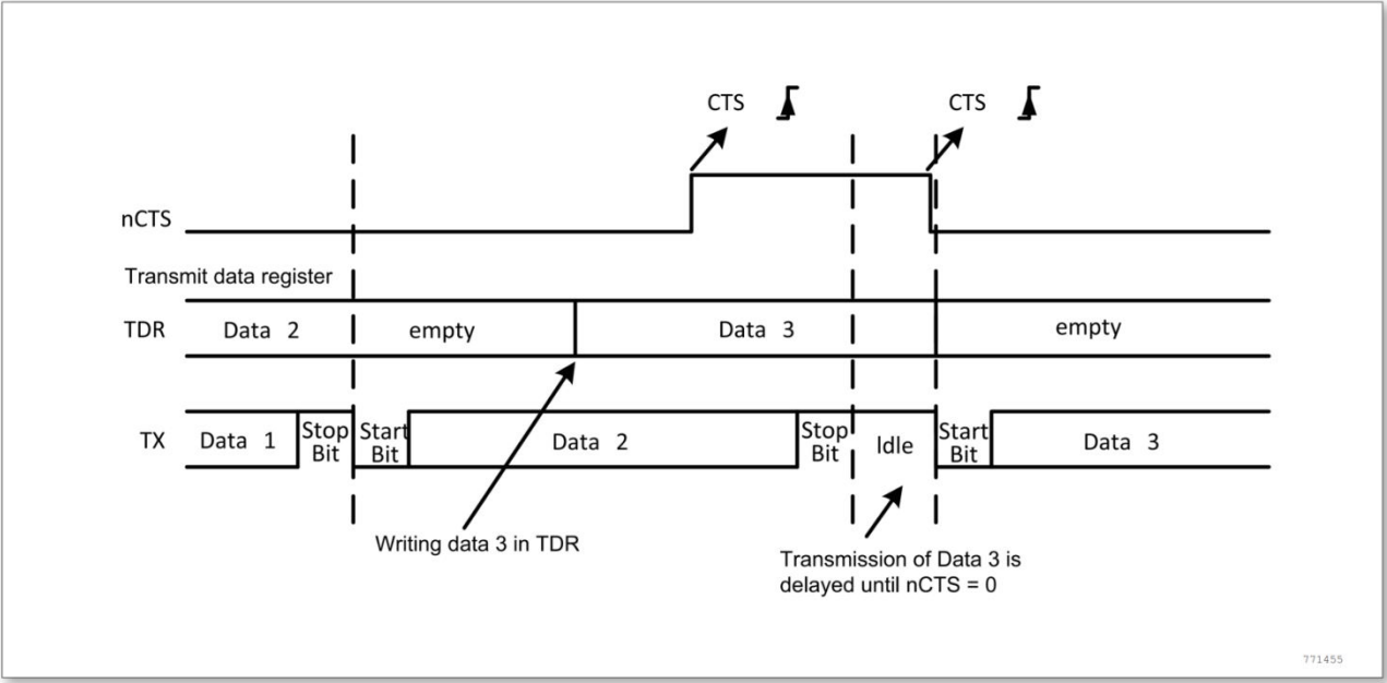
图 20-9 CTS 流控制
