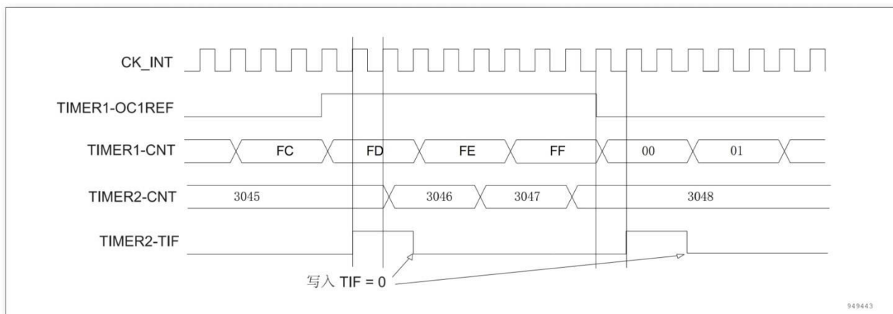
图 12-42 定时器 1 的 OC1REF 控制定时器 3
