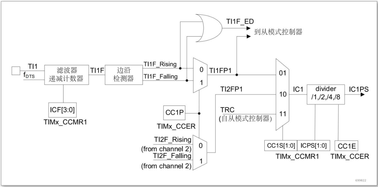
图 15-12 捕获/比较通道：（通道 1 输入部分）
