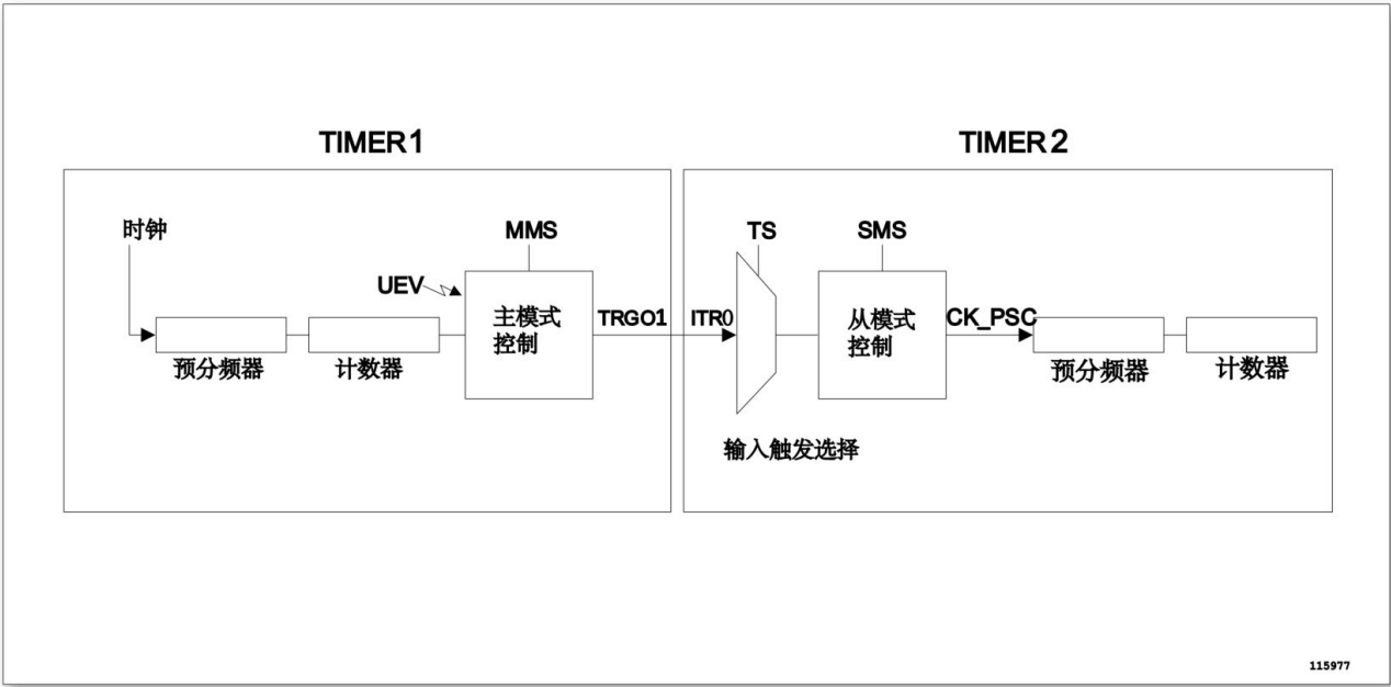
图 13-41 主/从定时器的例子
