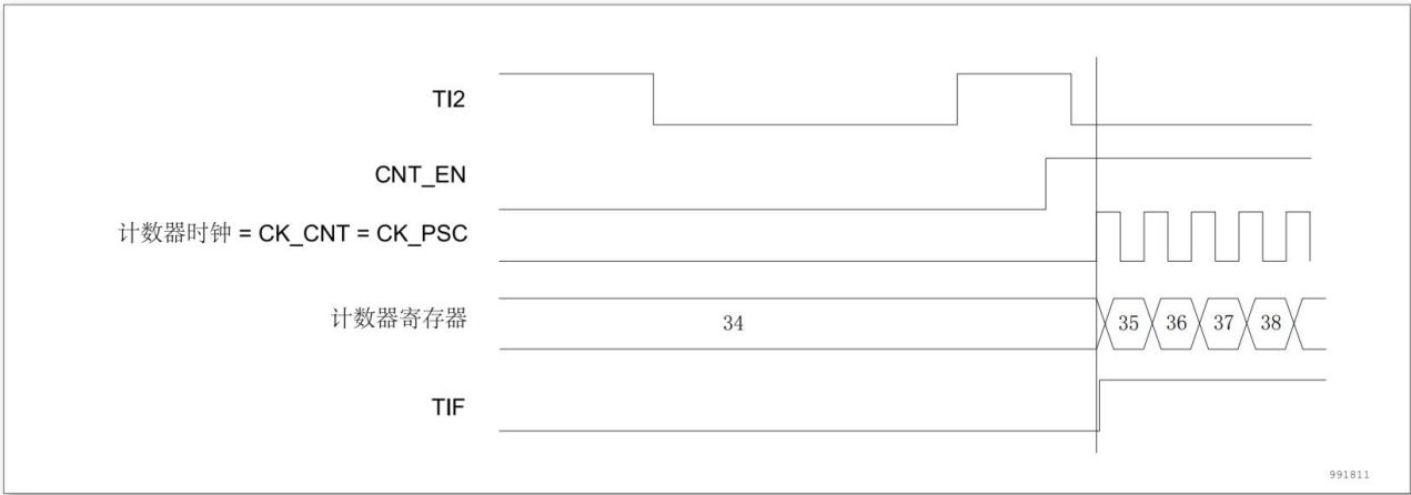
图 13-39 触发模式下的控制电路
