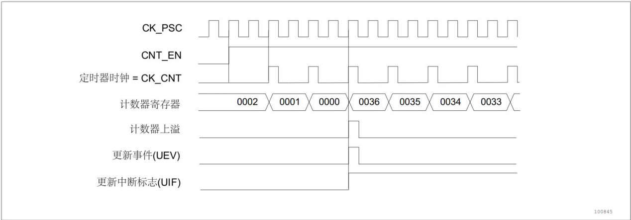
图 11-11 计数器时序图，内部时钟分频因子为 2
