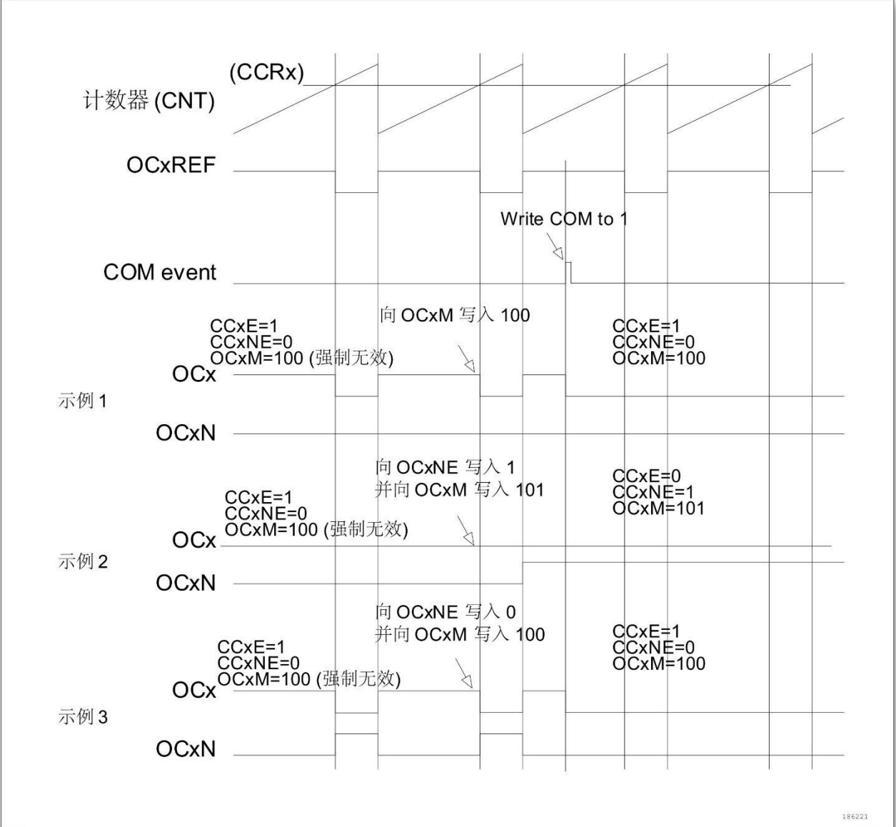
图 11-41 产生六步 PWM，使用 COM 的例子 (OSSR = 1)
