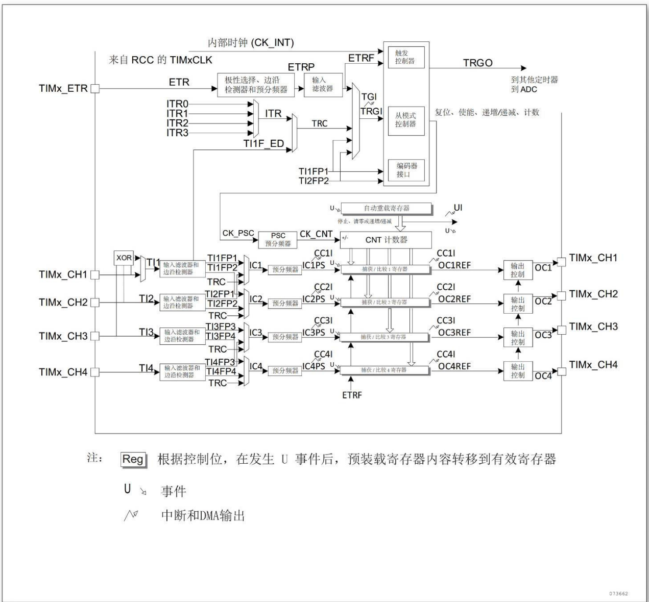
图 12-1 通用定时器框图
