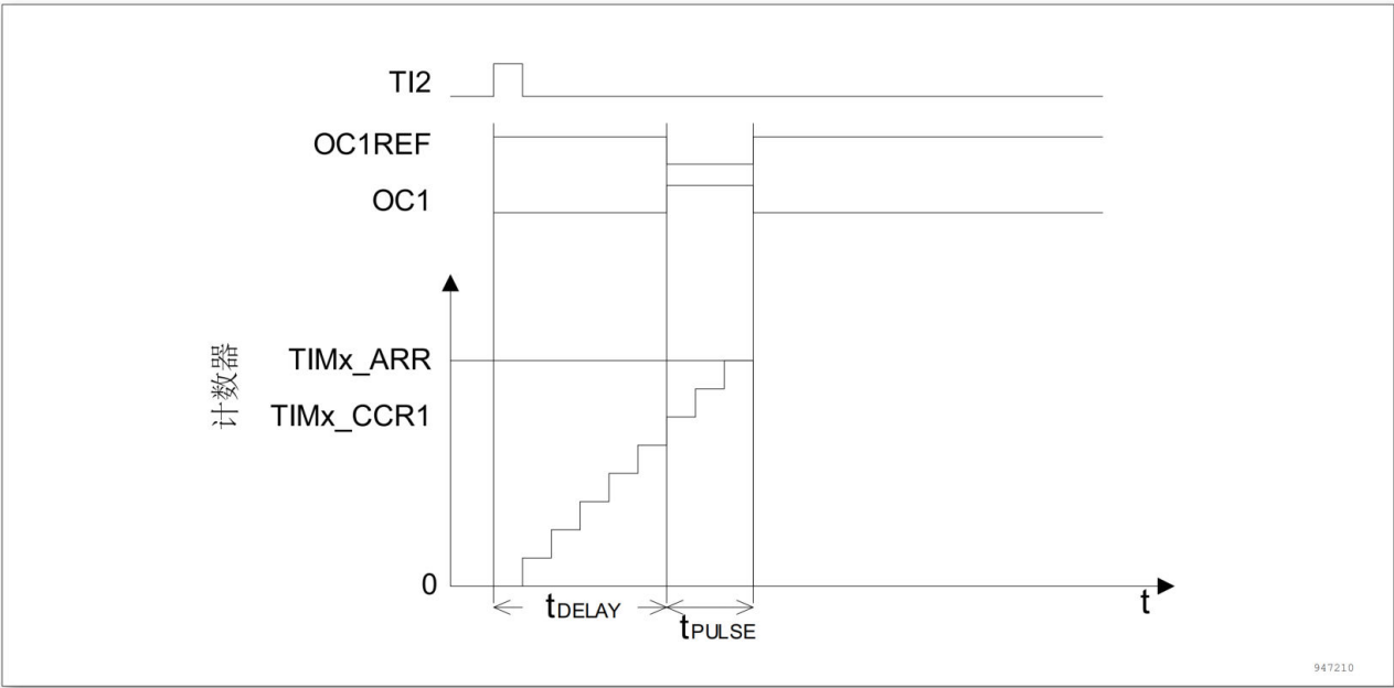
图 11-42 单脉冲模式的例子
