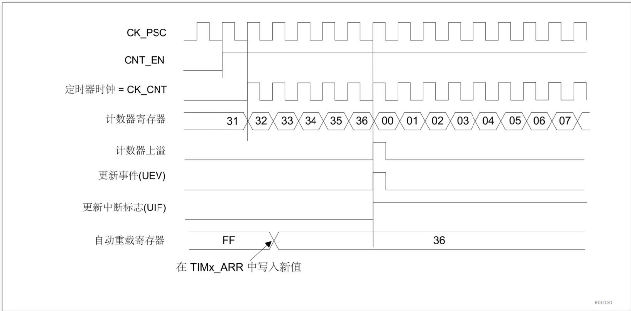
图 11-8 计数器时序图，当 ARPE = 0 时的更新事件 (TIMx_ARR 没有预装入)
