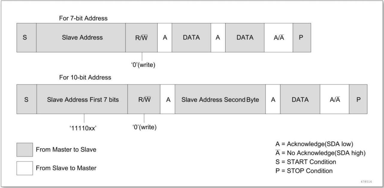
图 19-4 主发送协议
