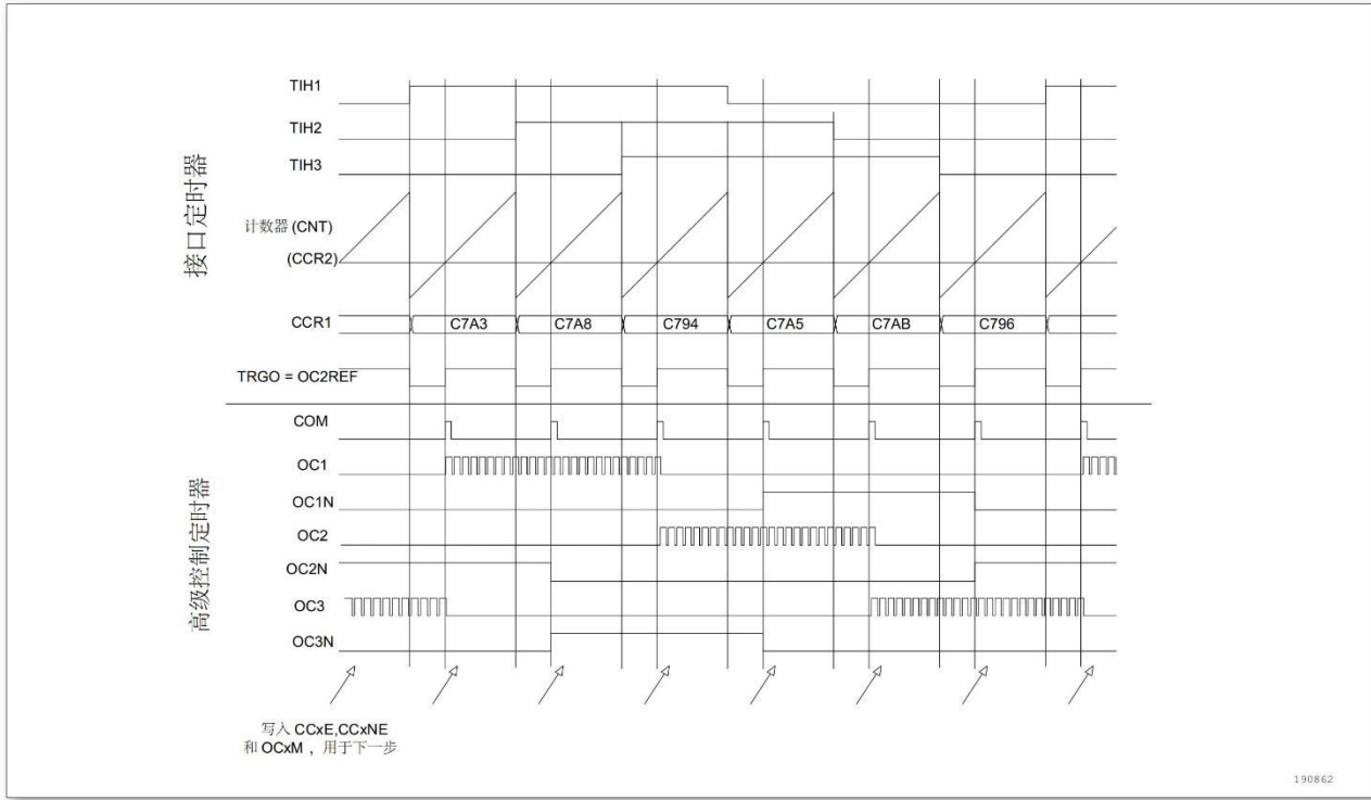
图 11-45 霍尔传感器接口的实例
