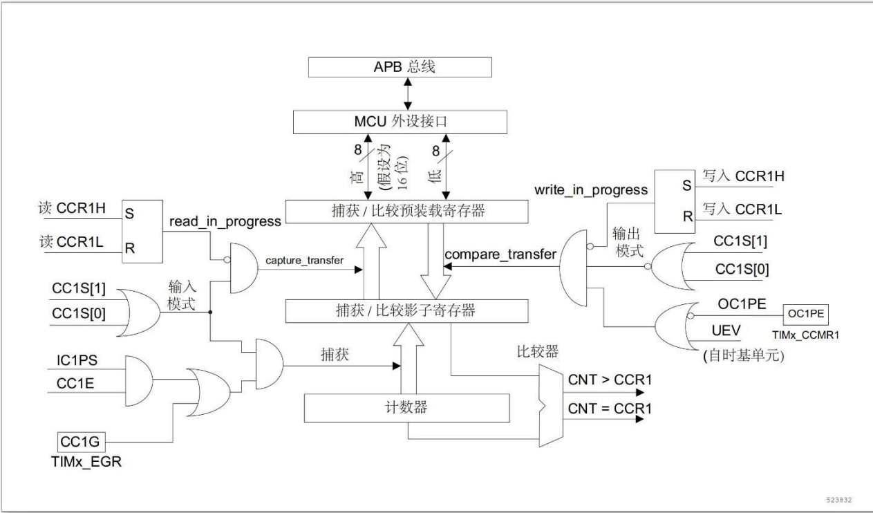
图 11-28 捕获/比较通道 1 的主电路
