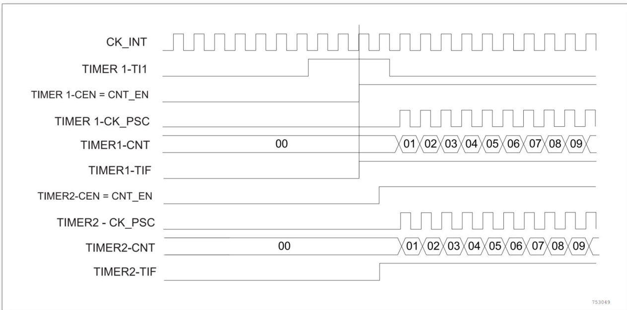
图 12-46 使用定时器 1 的 TI1 输入触发定时器 1 和定时器 3
