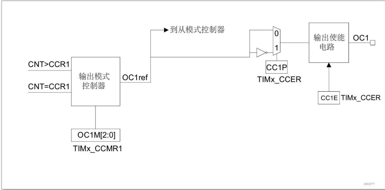
图 14-14 捕获/比较通道的输出部分 (通道 1)
