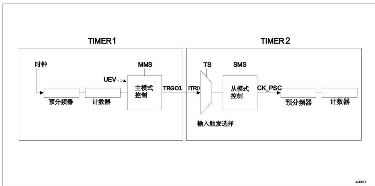
图 12-41 主/从定时器的例子
