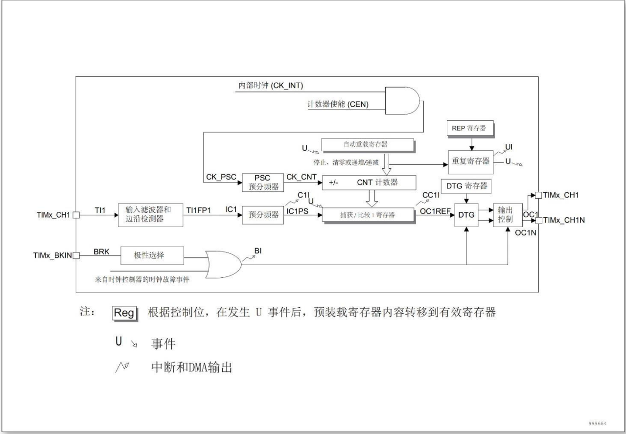
图 15-1 基本定时器 TIM16 和 TIM17 框图
