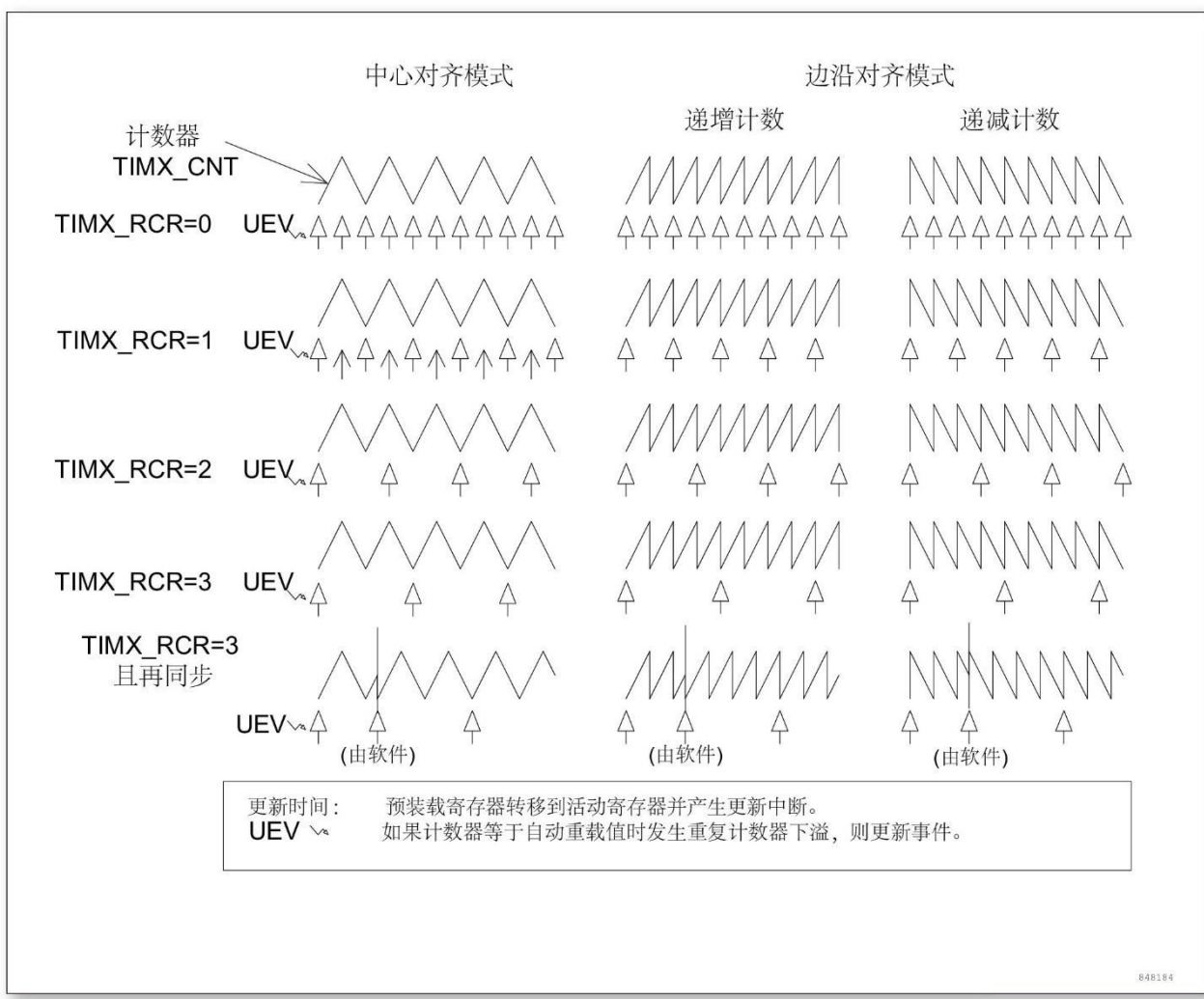
图 11-21 不同模式下更新速率的例子，及 TIMx_RCR 的寄存器设置
