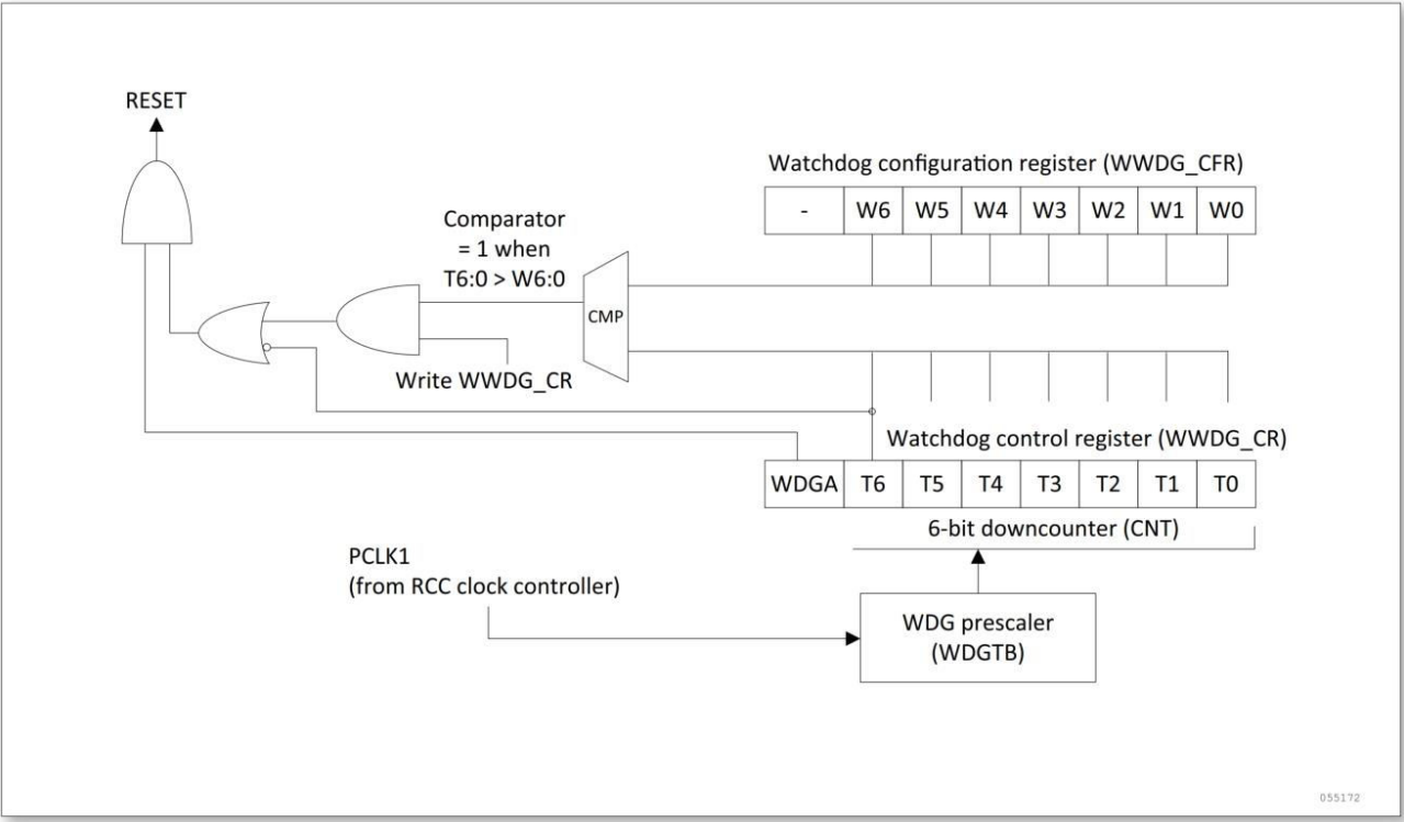
图 17-1 看门狗框图
