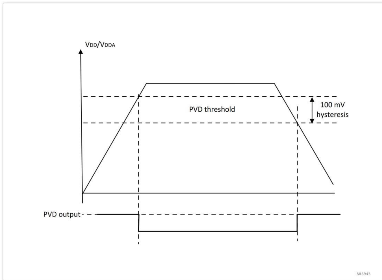
图 4-3 PVD 阈值
