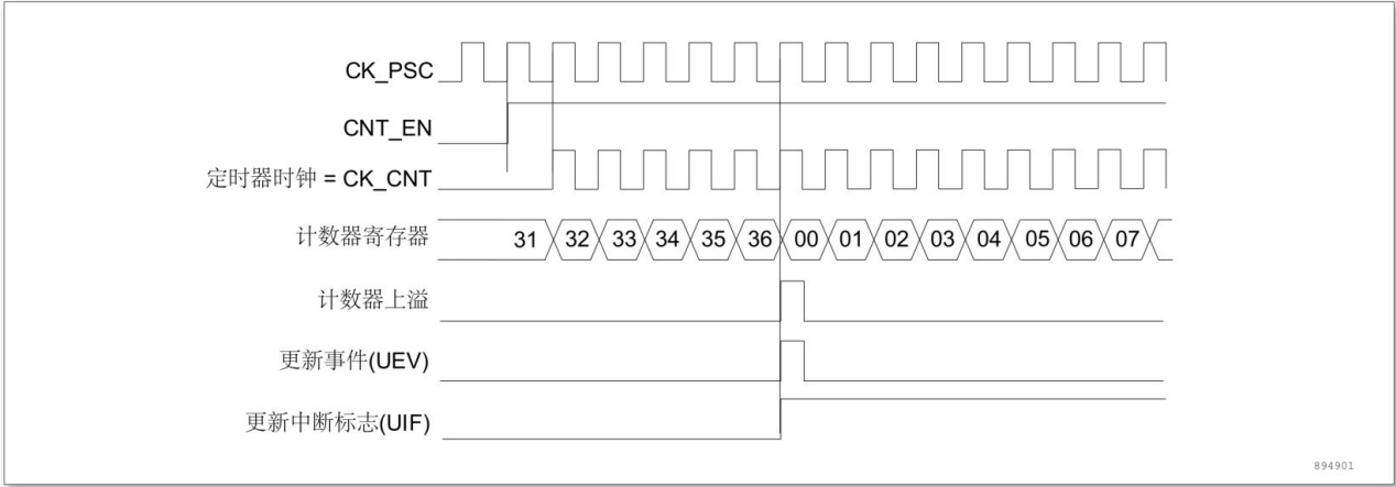
图 14-4 计数器时序图，内部时钟分频因子为 1
