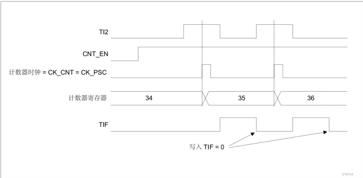
图 11-24 外部时钟模式 1 下的控制电路
