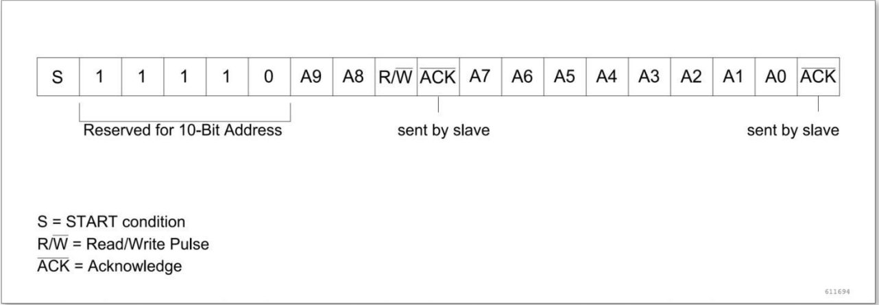
图 19-3 10 位的地址格式
