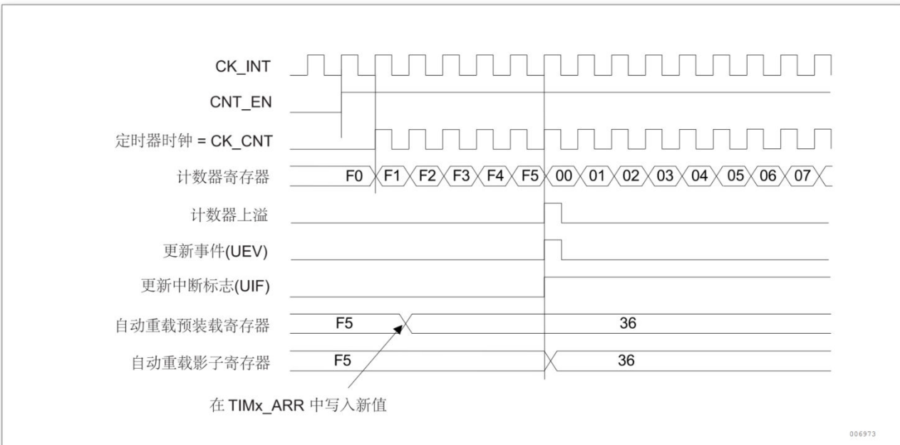
图 15-9 计数器时序图，当 ARPE=1 时的更新事件(TIMX ARR 预装载)
