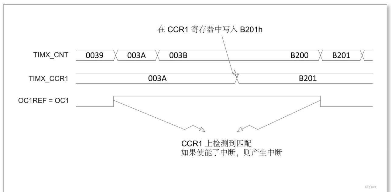
图 13-30 输出比较模式, 翻转 OC1
