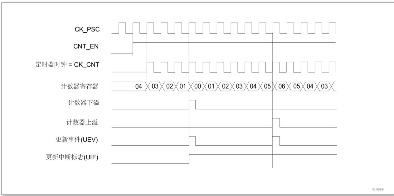
图 11-15 计数器时序图，内部时钟分频因子为 1，TIMx_ARR = 0x06
