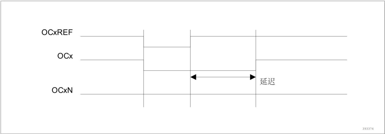
图 11-37 死区波形延迟大于负脉冲
