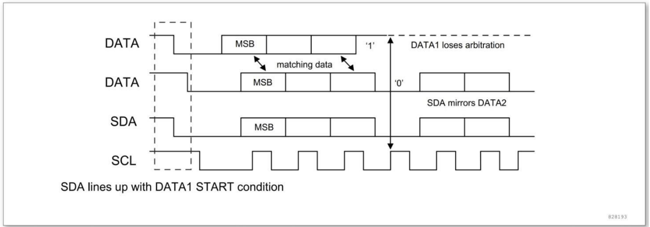
图 19-10 多个主机仲裁
