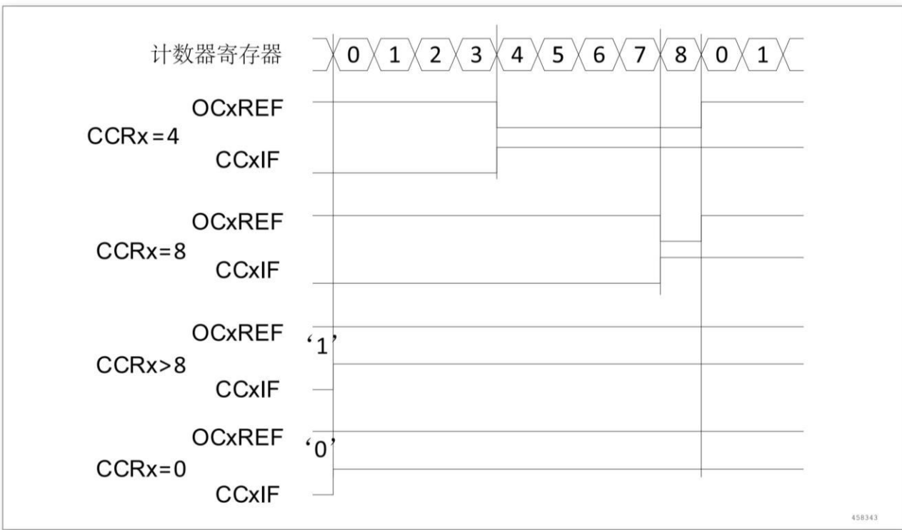
图 13-31 边沿对齐的 PWM 波形 (ARR = 8)
