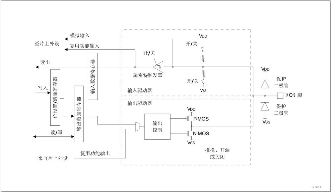
图 6-1 I/O 端口位的基本结构
