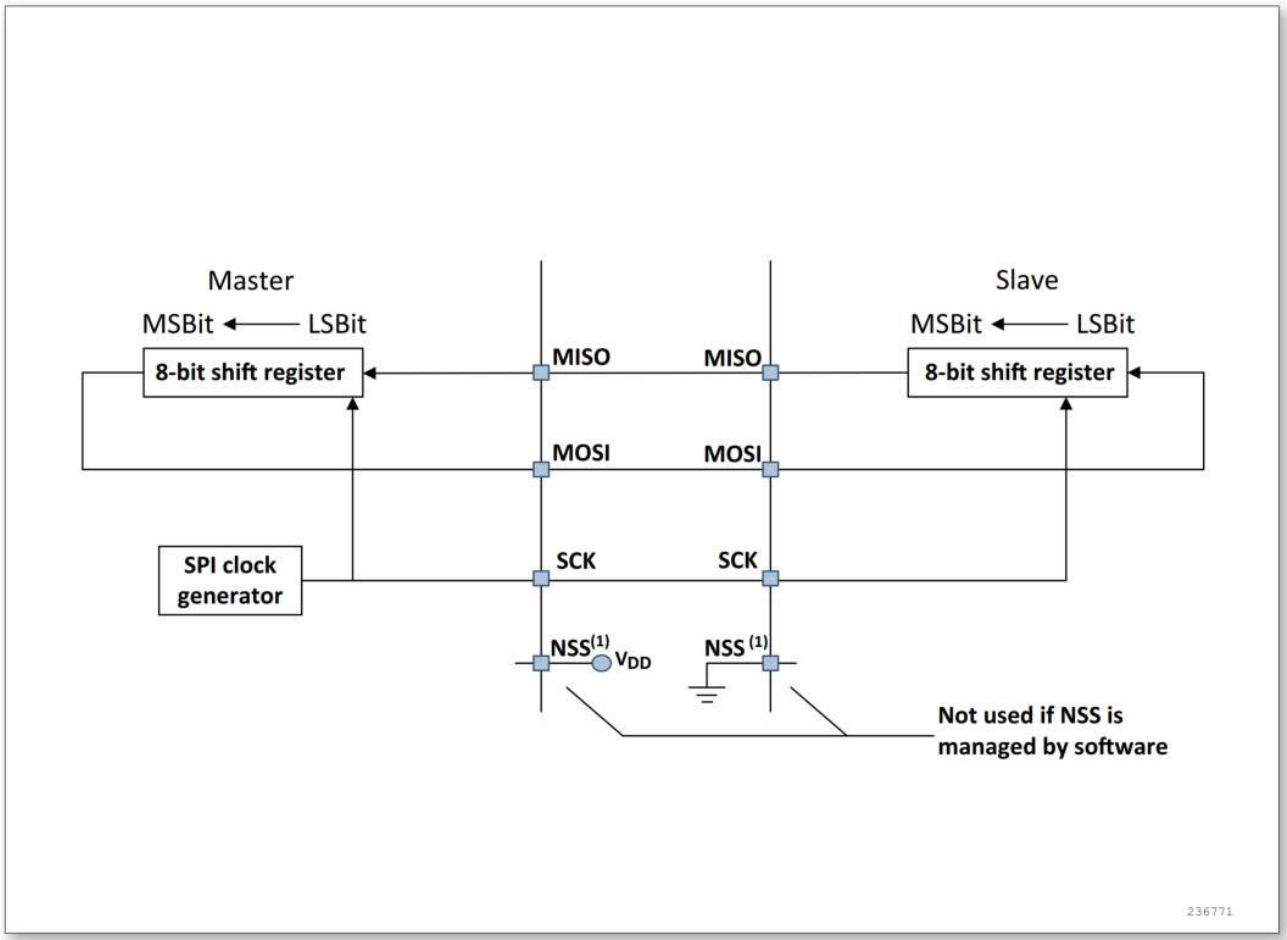
图 18-2 单主和单从应用
