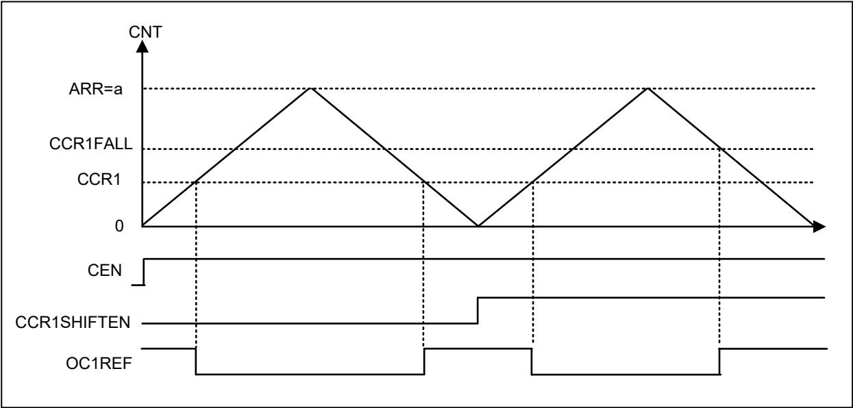
图 11-35 移相功能示意图
