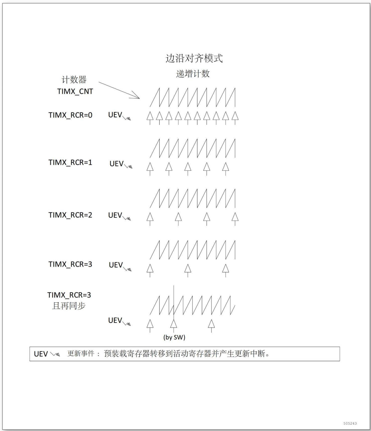
图 15-10 不同模式及不同 TIMX RCR 寄存器设置下更新速率的例子
