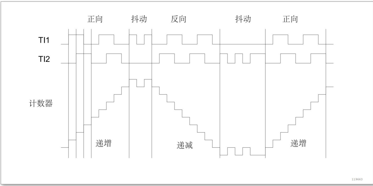
图 13-35 编码器模式下的计数器操作实例
