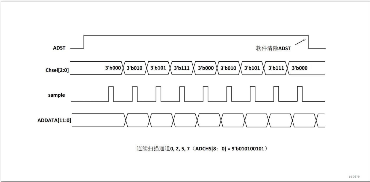
图 9-5 连续扫描模式使能通道转换时序图（通道方向从低到高）
