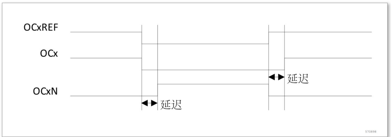
图 15-17 带死区插入的互补输出
