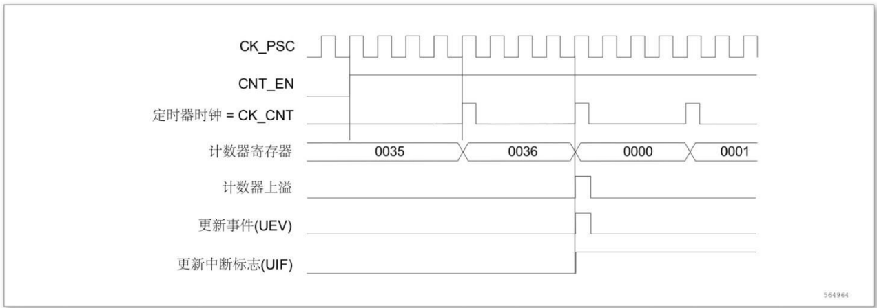
图 12-6 计数器时序图，内部时钟分频因子为 4
