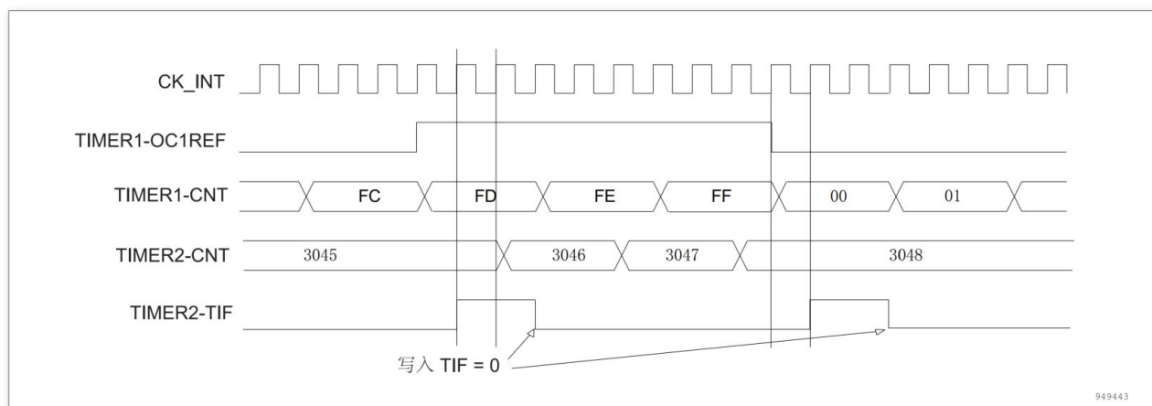
图 13-42 定时器 1 的 OC1REF 控制定时器 2
