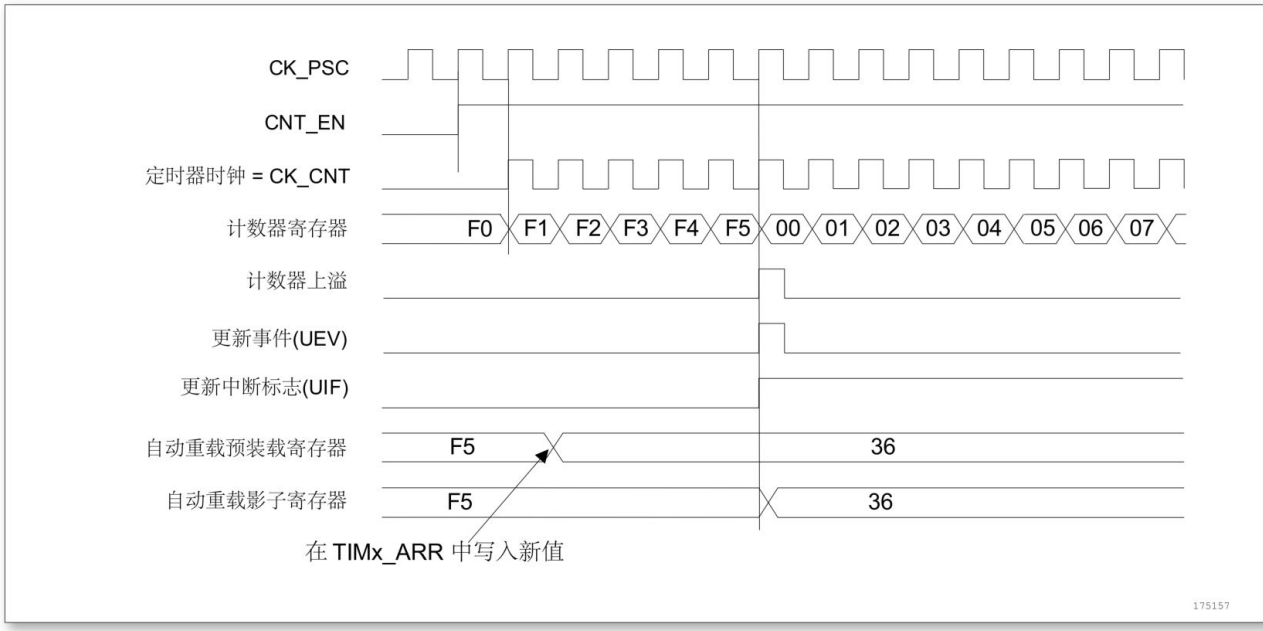
图 11-9 计数器时序图，当 ARPE = 1 时的更新事件 (预装入了 TIMx_ARR)
