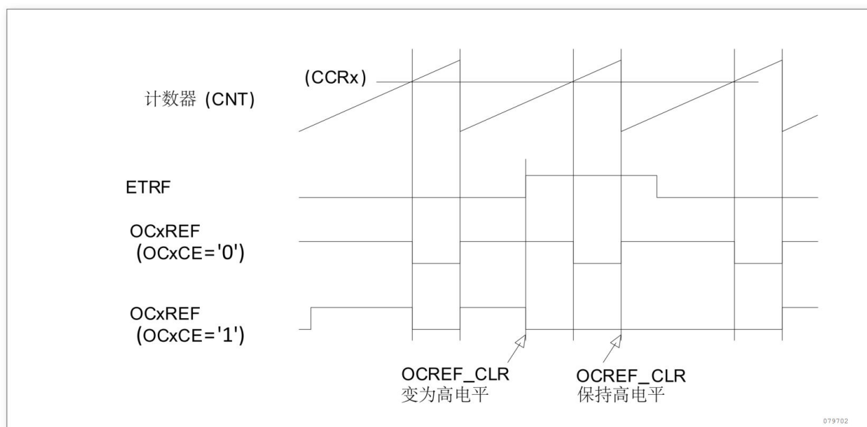
图 13-34 清除 TIMx 的 OCxREF
