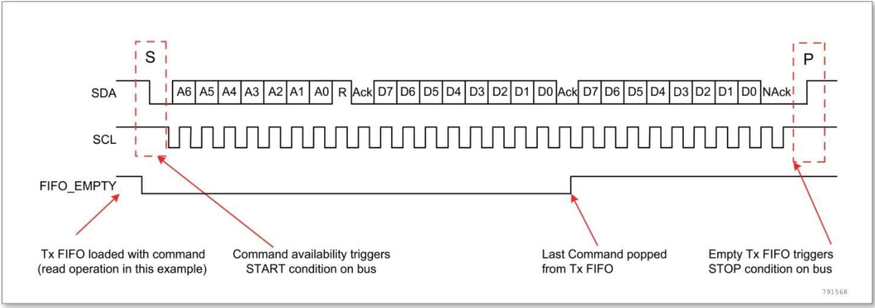
图 19-9 主接收 - Tx FIFO 为空
