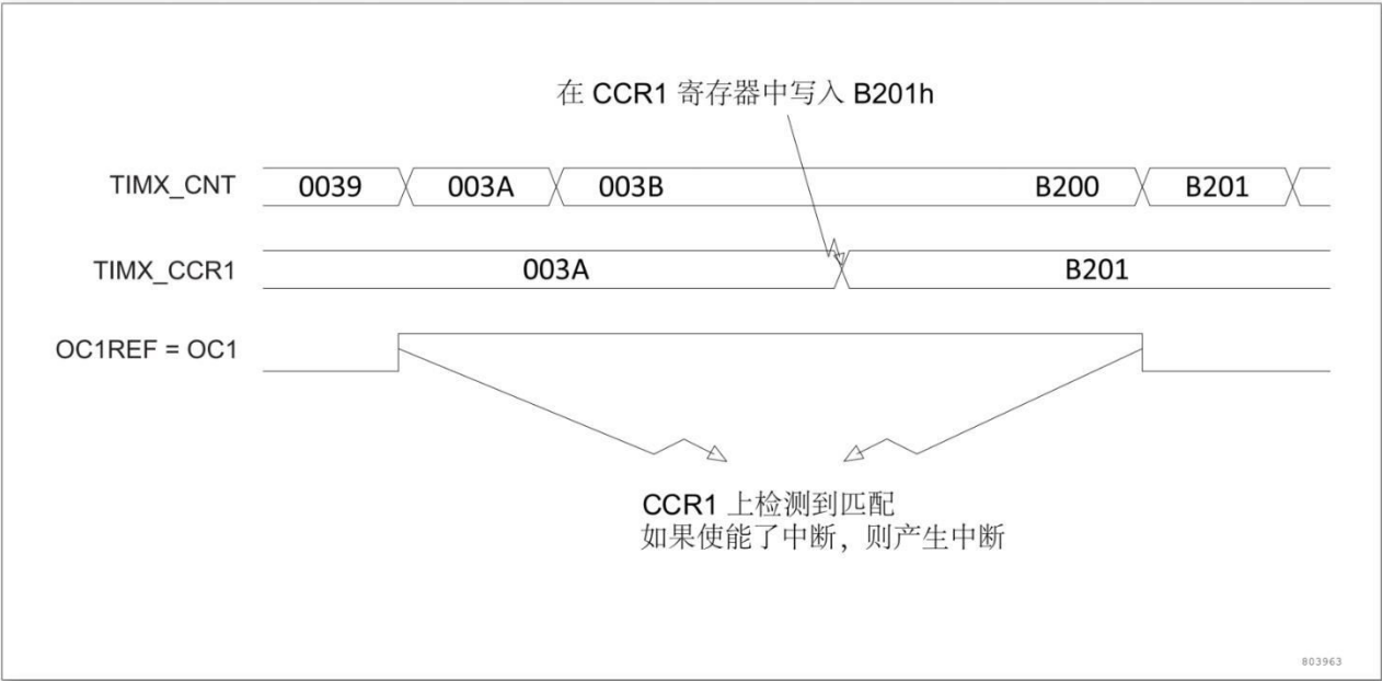
图 12-30 输出比较模式, 翻转 OC1
