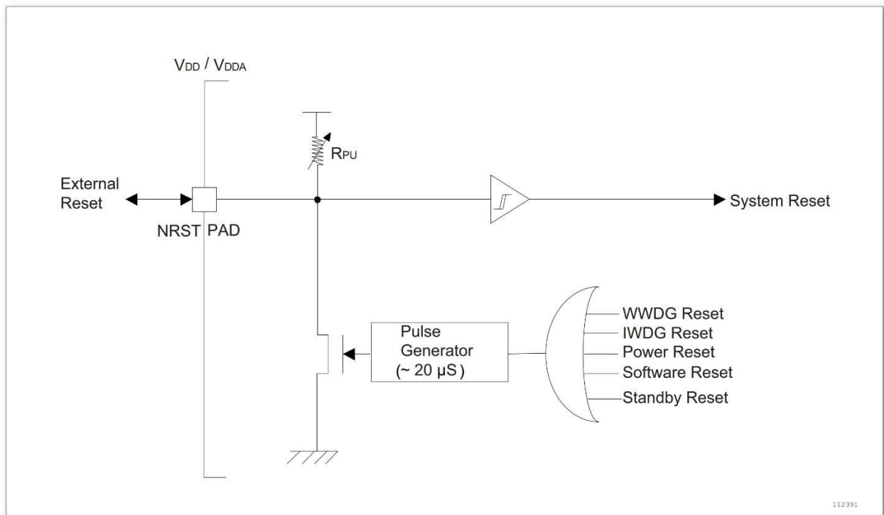
图 5-1 复位电路
