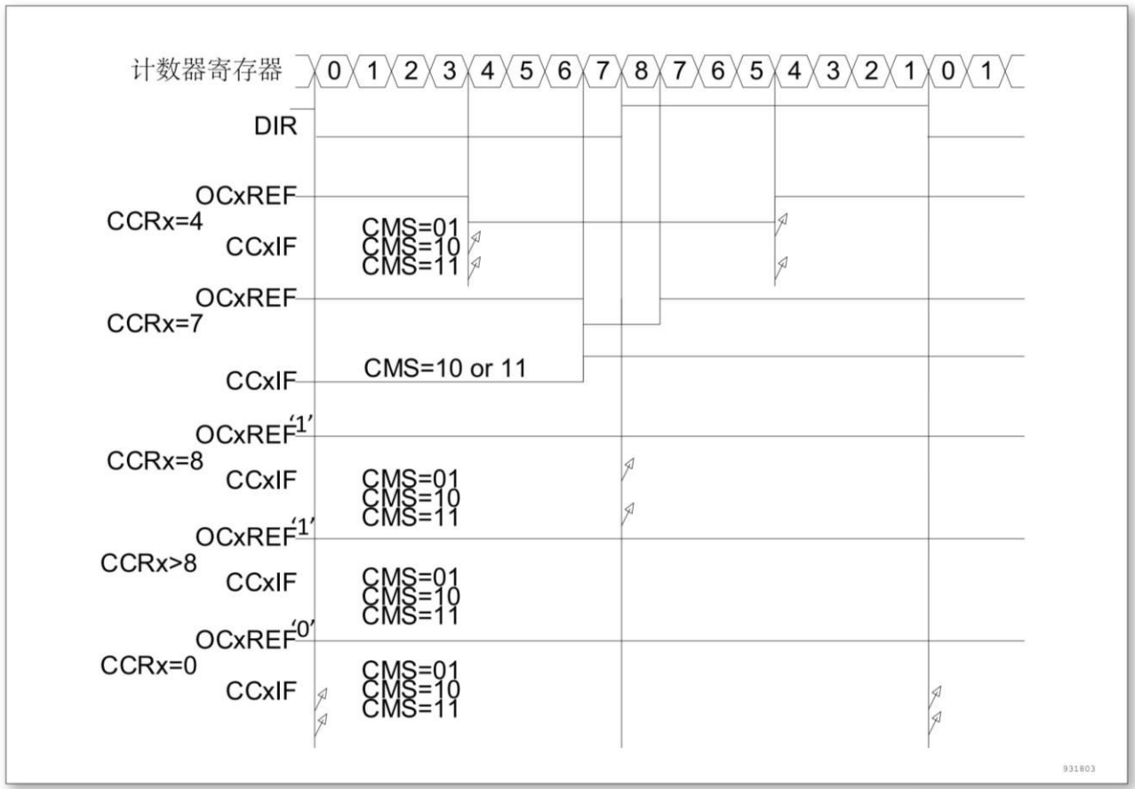
图 13-32 中央对齐的 PWM 波形 (ARR = 8)
