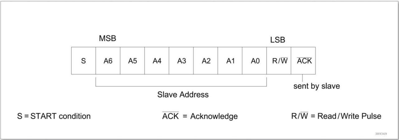
图 19-2 7 位的地址格式
