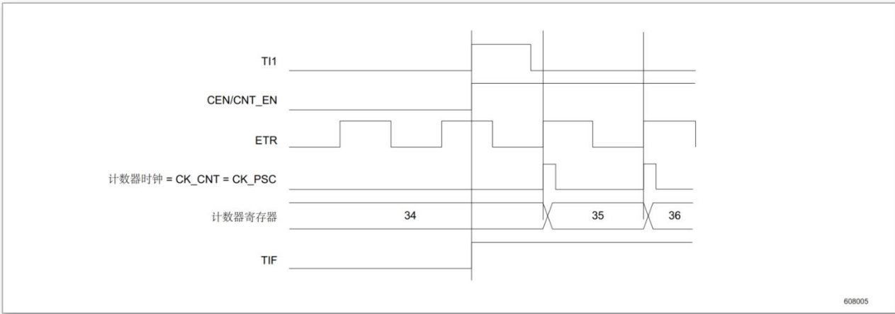
图 11-49 外部时钟模式 2 + 触发模式下的控制电路
