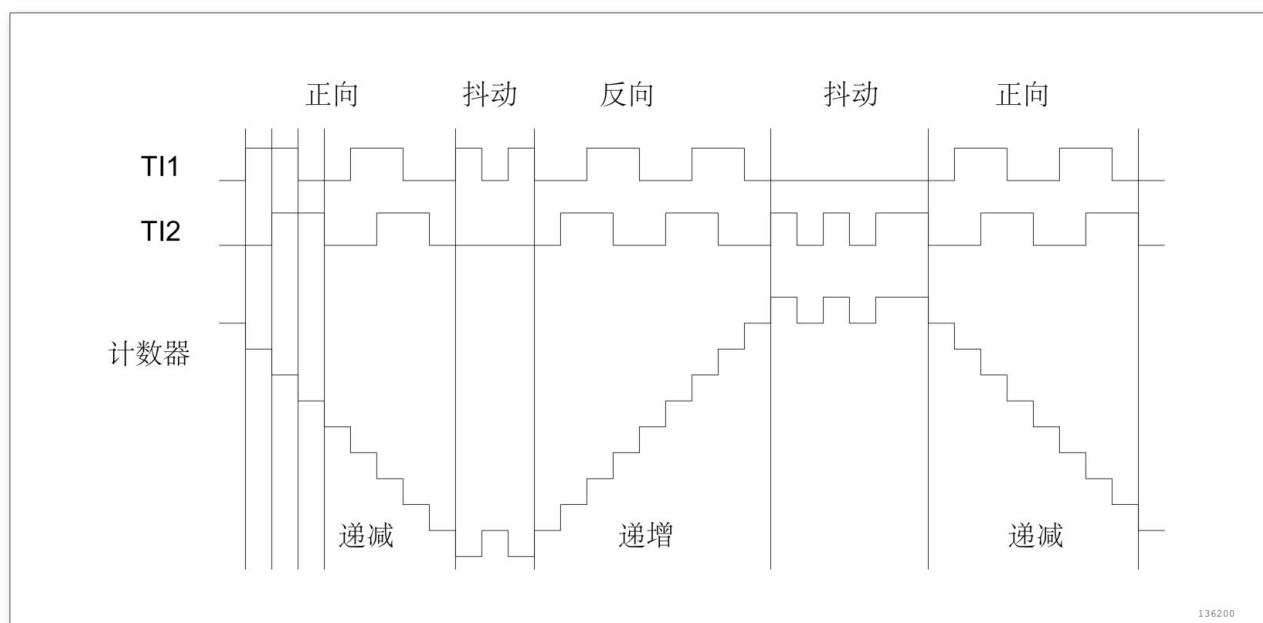
图 11-43 编码器模式下的计数器操作实例
