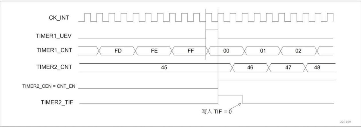
图 12-44 使用定时器 1 的更新触发定时器 2
