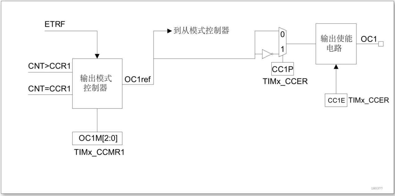
图 11-29 捕获/比较通道的输出部分 (通道 1 至 3)
