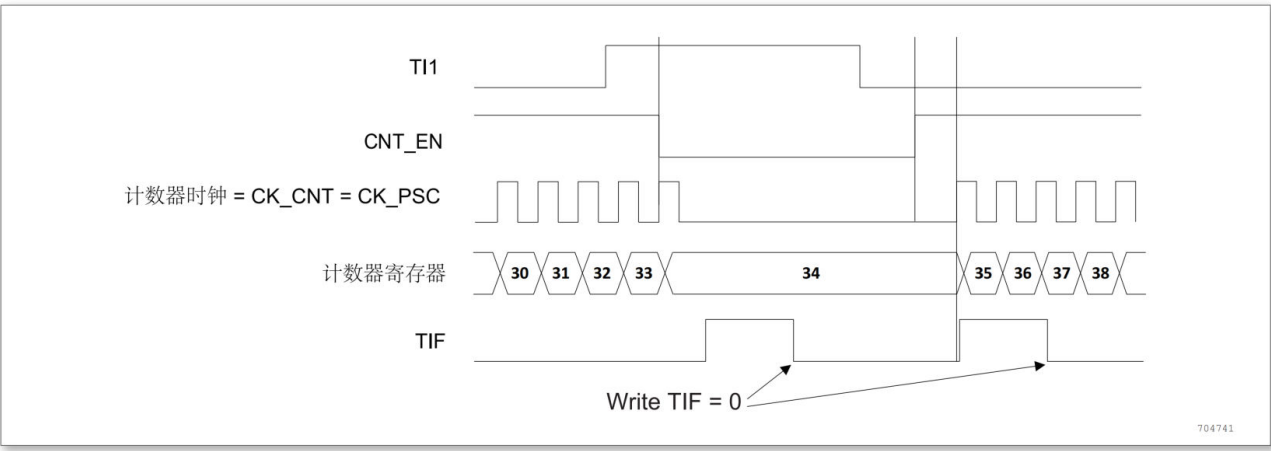
图 13-38 门控模式下的控制电路
