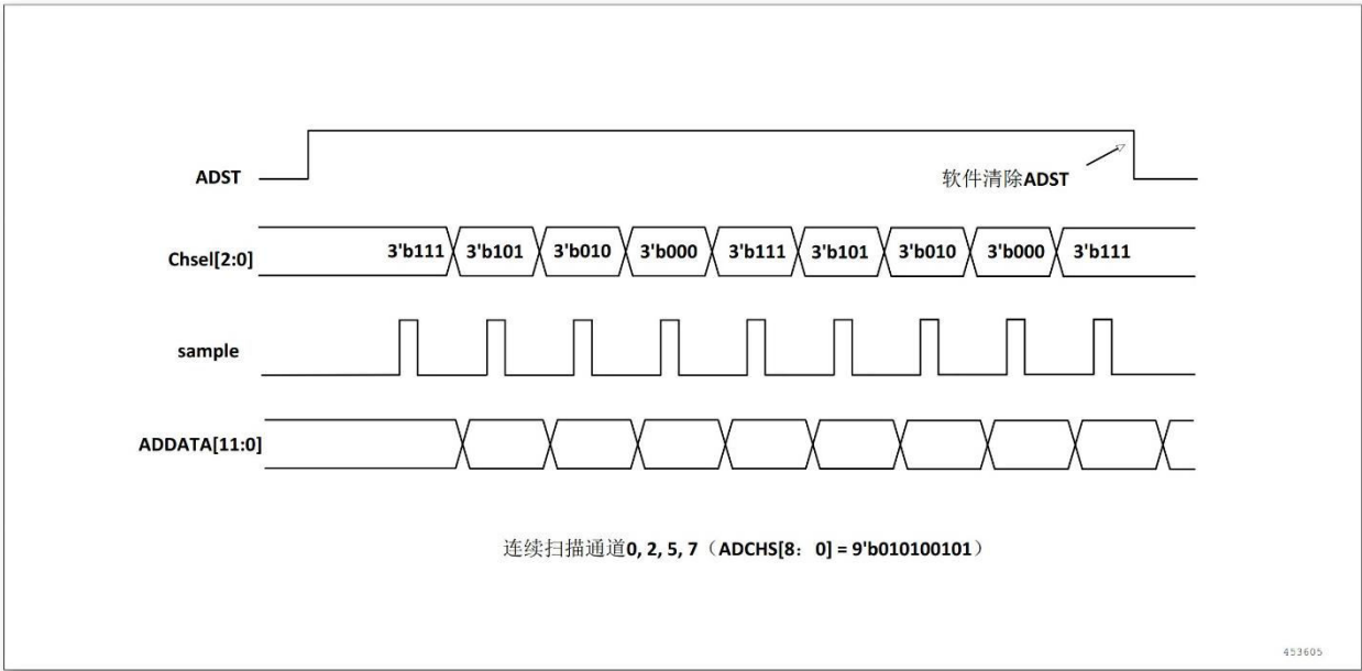
图 9-6 连续扫描模式使能通道转换时序图（通道方向从高到低）
