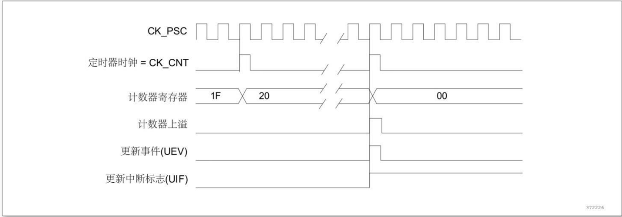
图 12-7 计数器时序图，内部时钟分频因子为 N
