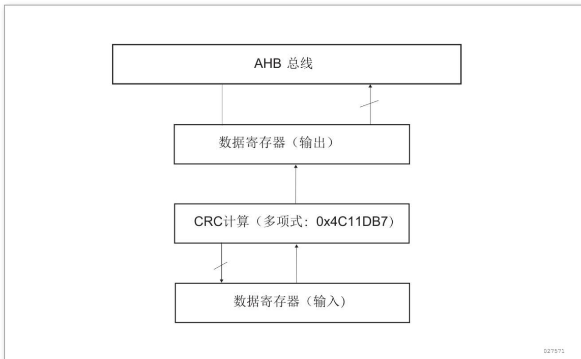
图 3-1 CRC 计算单元框图
