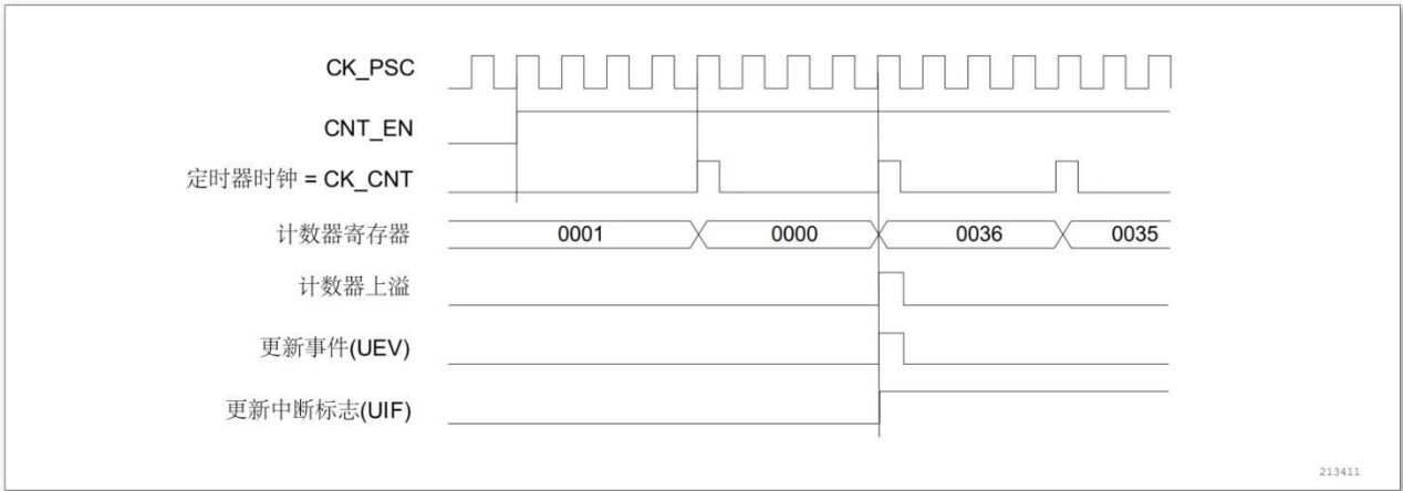
图 12-12 计数器时序图，内部时钟分频因子为 4
