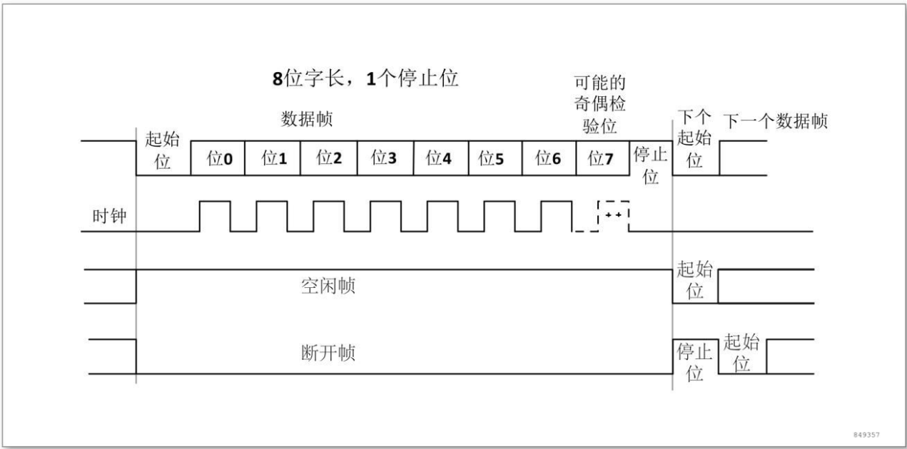
图 20-2 UART 时序
