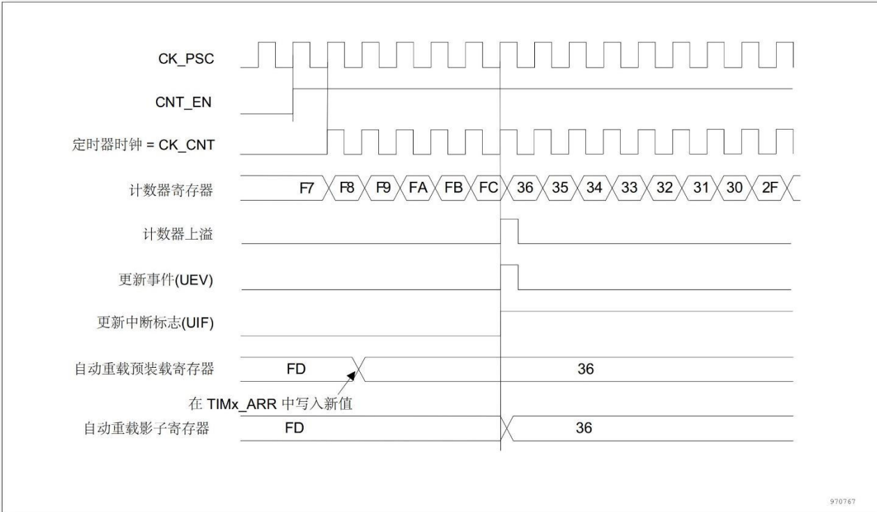
图 12-20 计数器时序图， ARPE = 1 时的更新事件 (计数器溢出)
