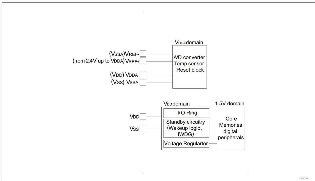
图 4-1 电源框图
