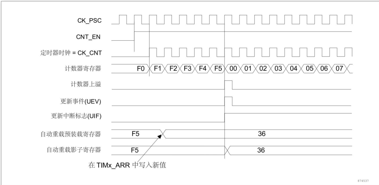
图 13-9 计数器时序图，当 ARPE = 1 时的更新事件 (预装入了 TIMx_ARR)
