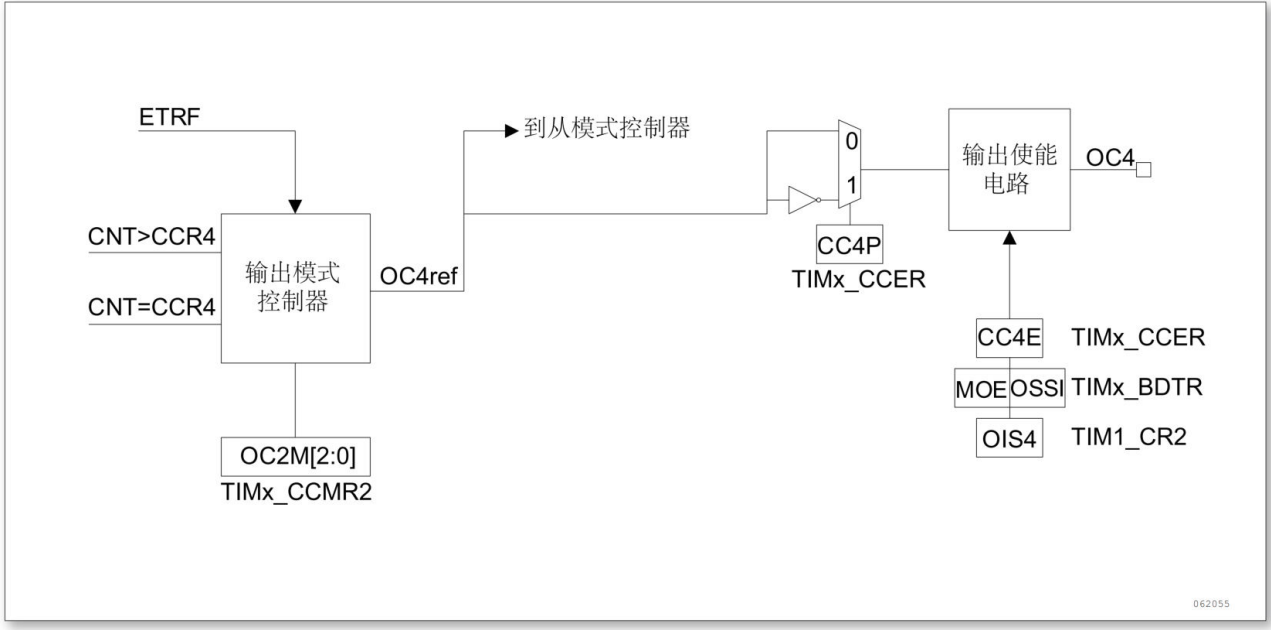
图 11-30 捕获/比较通道的输出部分 (通道 4)
