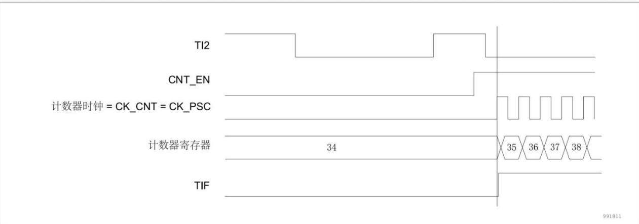
图 12-39 触发器模式下的控制电路
