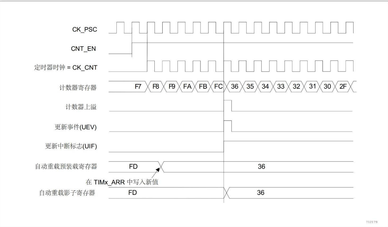
图 11-20 计数器时序图， ARPE = 1 时的更新事件 (计数器溢出)
