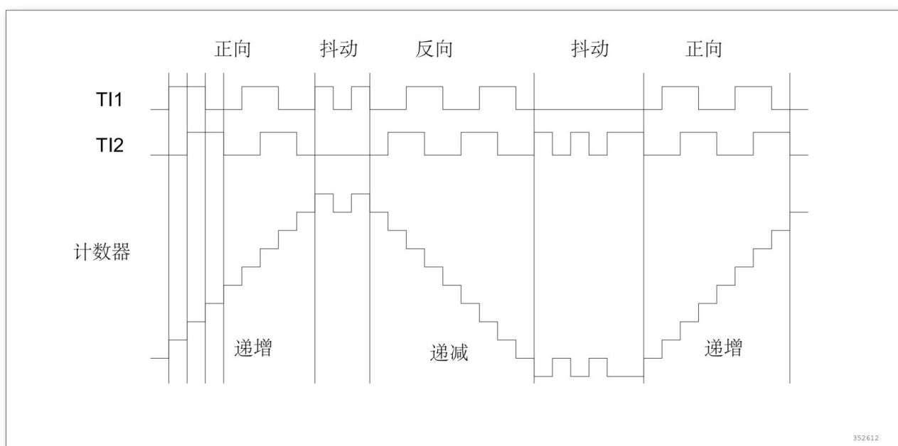
图 11-43 编码器模式下的计数器操作实例
