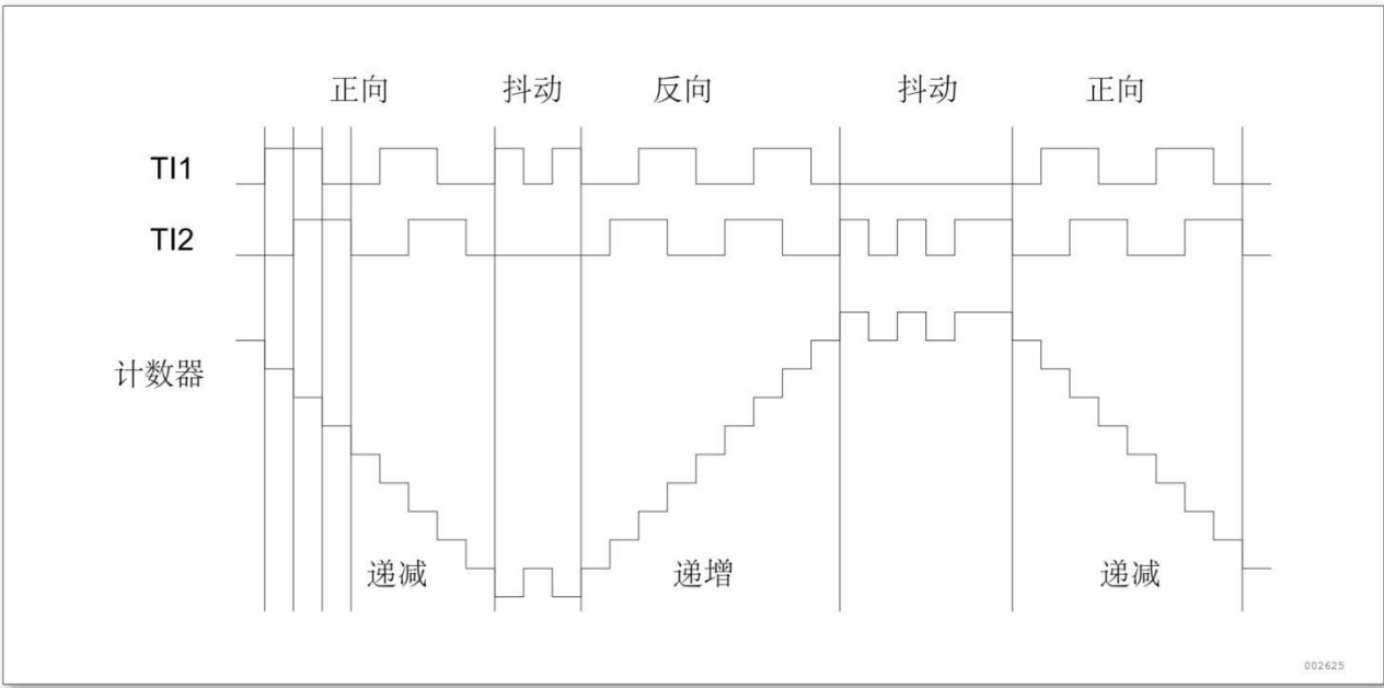
图 12-36 IC1FP1 反相的编码器接口模式实例
