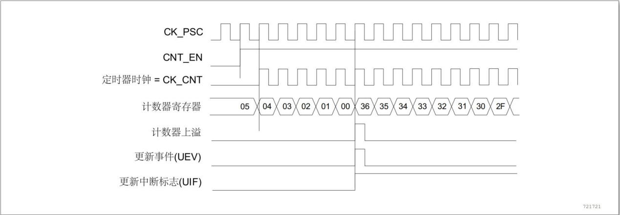
图 13-10 计数器时序图，内部时钟分频因子为 1
