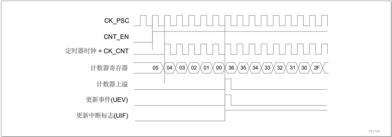
图 12-10 计数器时序图，内部时钟分频因子为 1
