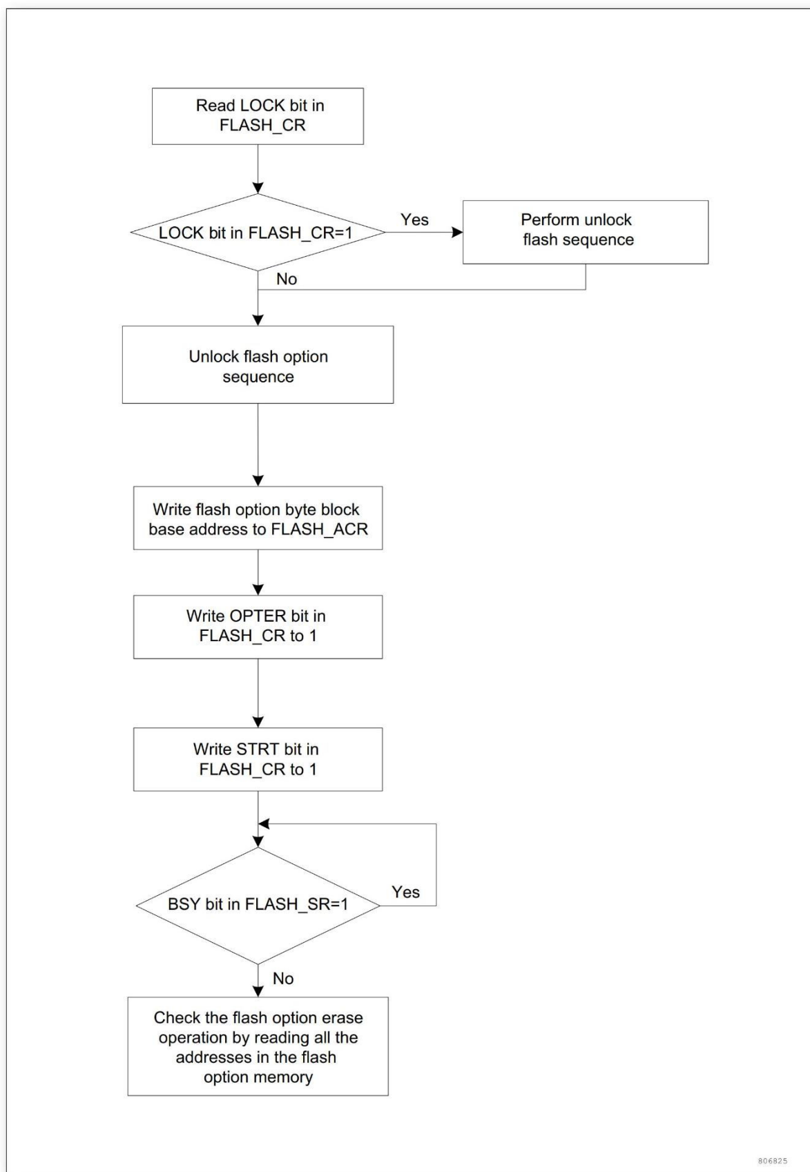
图 2-5 选项字节擦除流程
