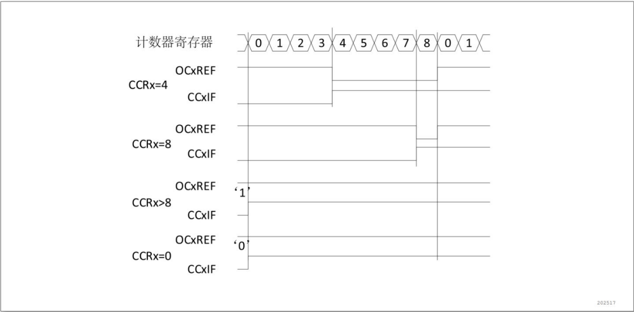
图 15-16 边沿对齐的 PWM 波形 (ARR=8)
