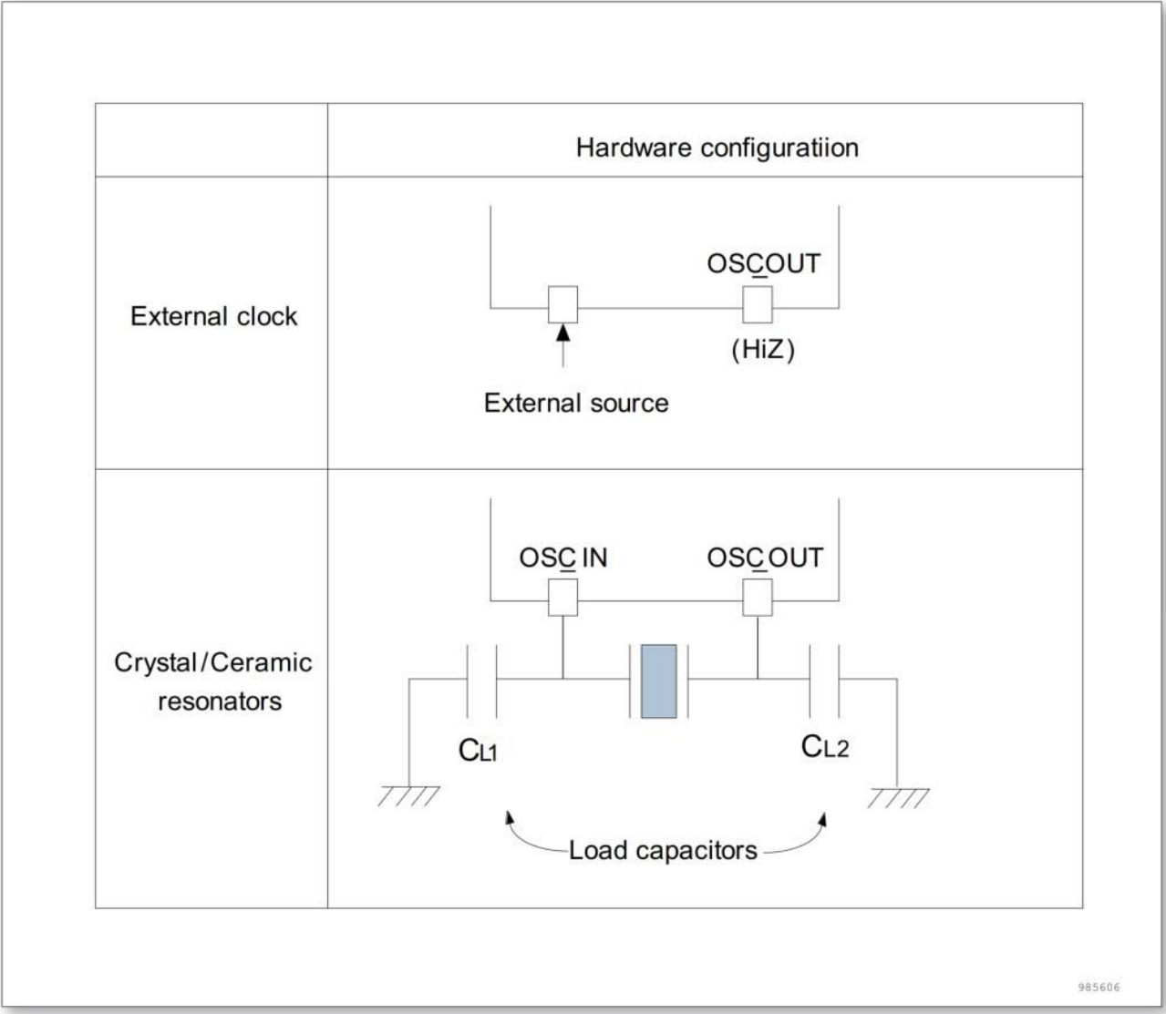
图 5-3 时钟源
