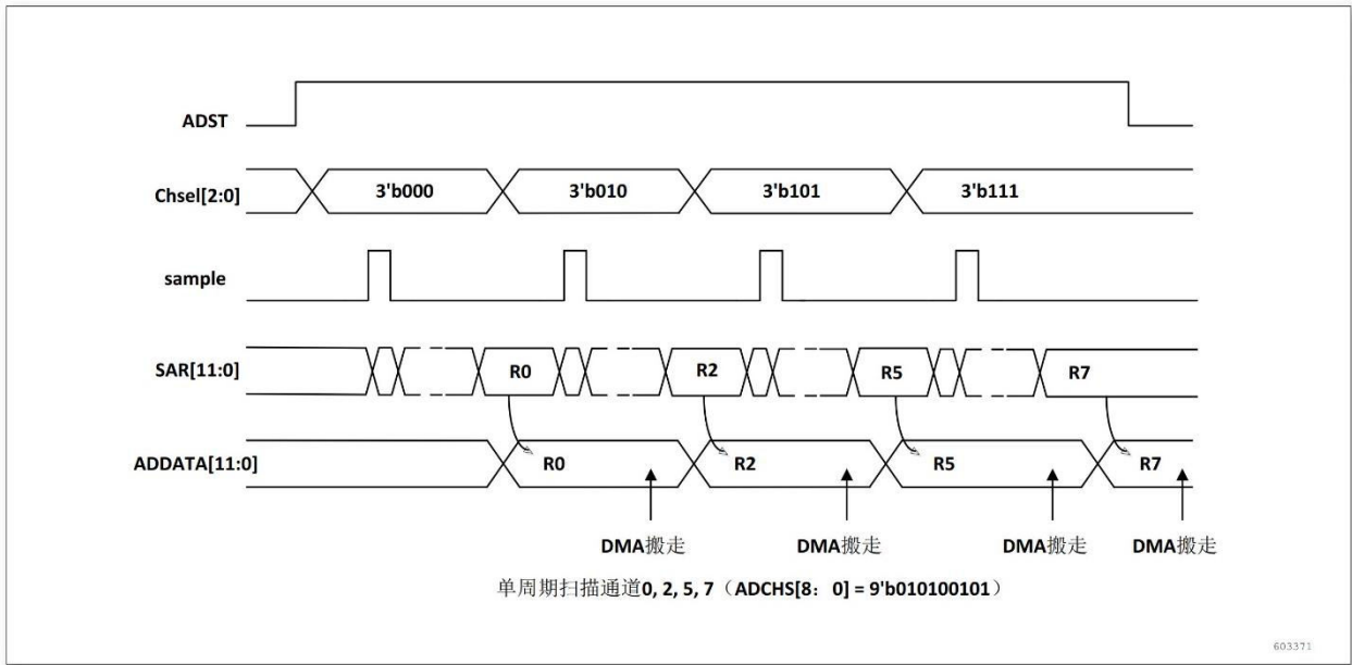
图 9-3 单周期扫描下使能通道转换时序图（通道方向从低到高）
