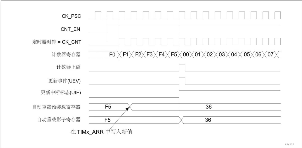
图 14-9 计数器时序图，当 ARPE = 1 时的更新事件 (预装载了 TIM14_ARR)
