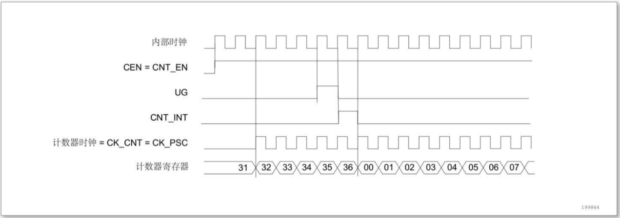
图 12-21 一般模式下的控制电路，内部时钟分频因子为 1
