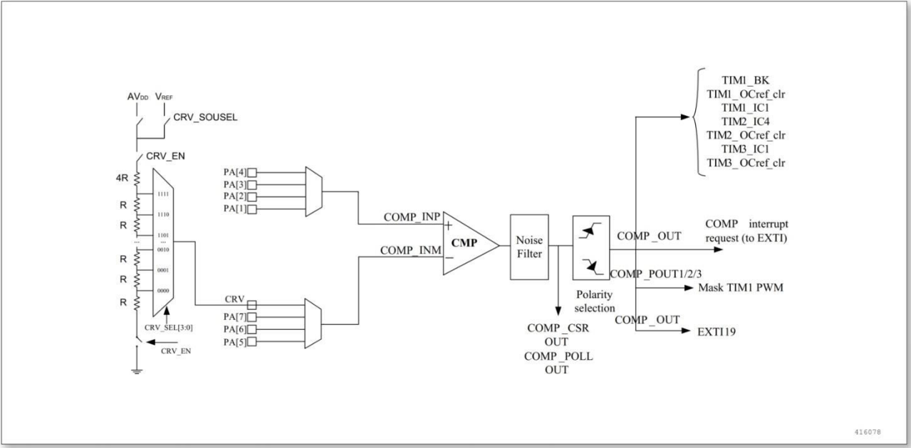
图 10-1 比较器框图
