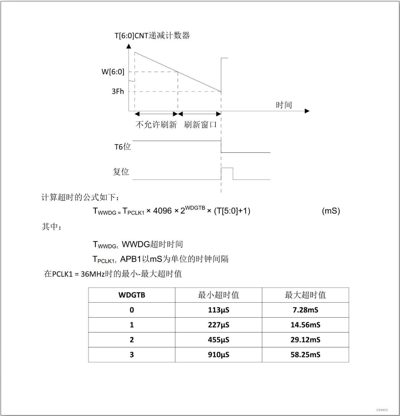
图 17-2 窗口看门狗时序图
