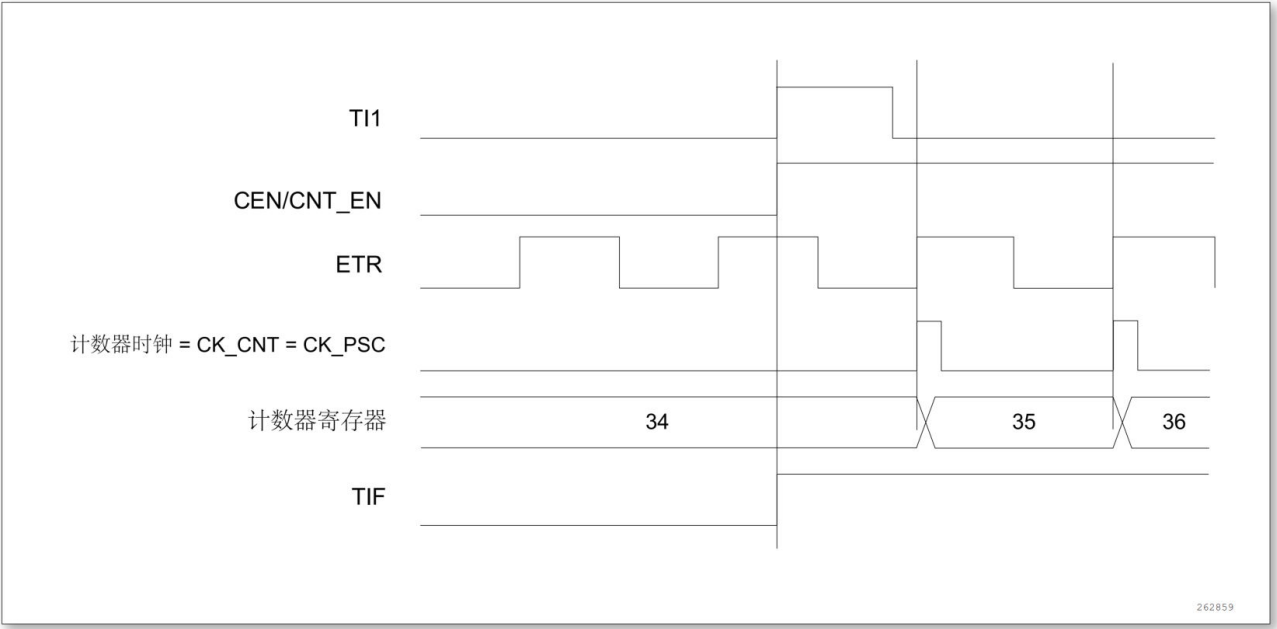
图 13-40 外部时钟模式 2+ 触发模式下的控制电路
