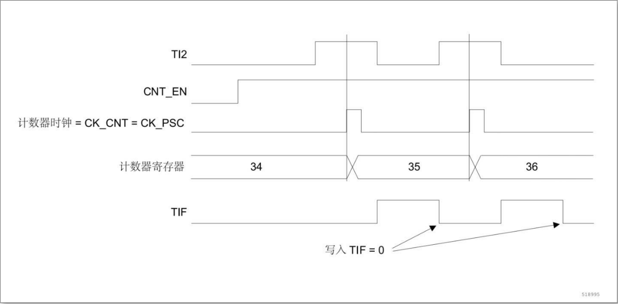
图 12-23 外部时钟模式 1 下的控制电路
