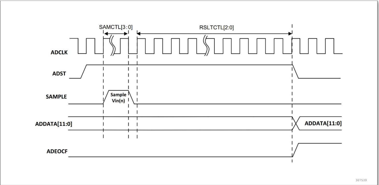
图 9-2 单次转换模式时序图
