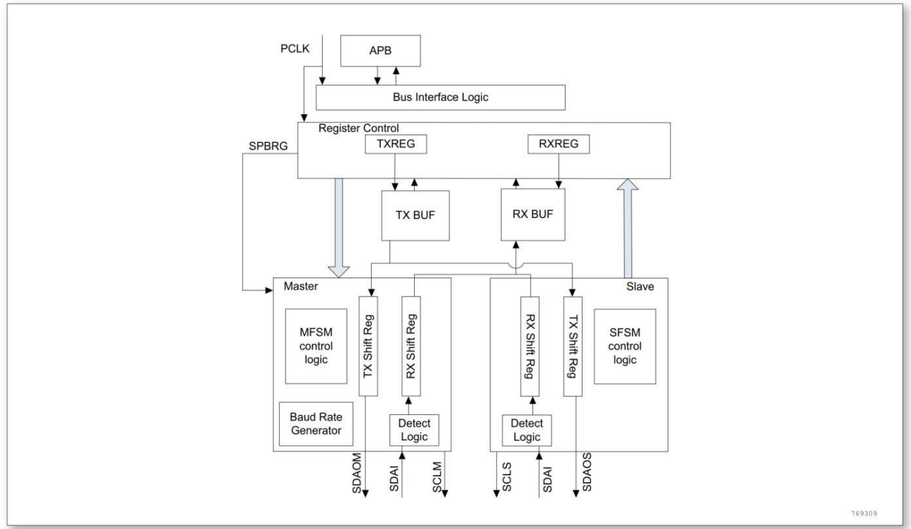
图 19-12 I2C 功能框图
