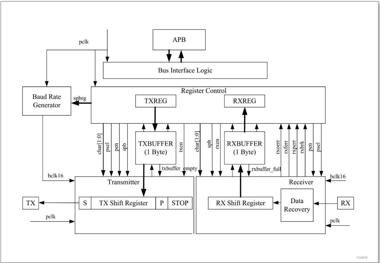
图 20-1 UART 方框图
