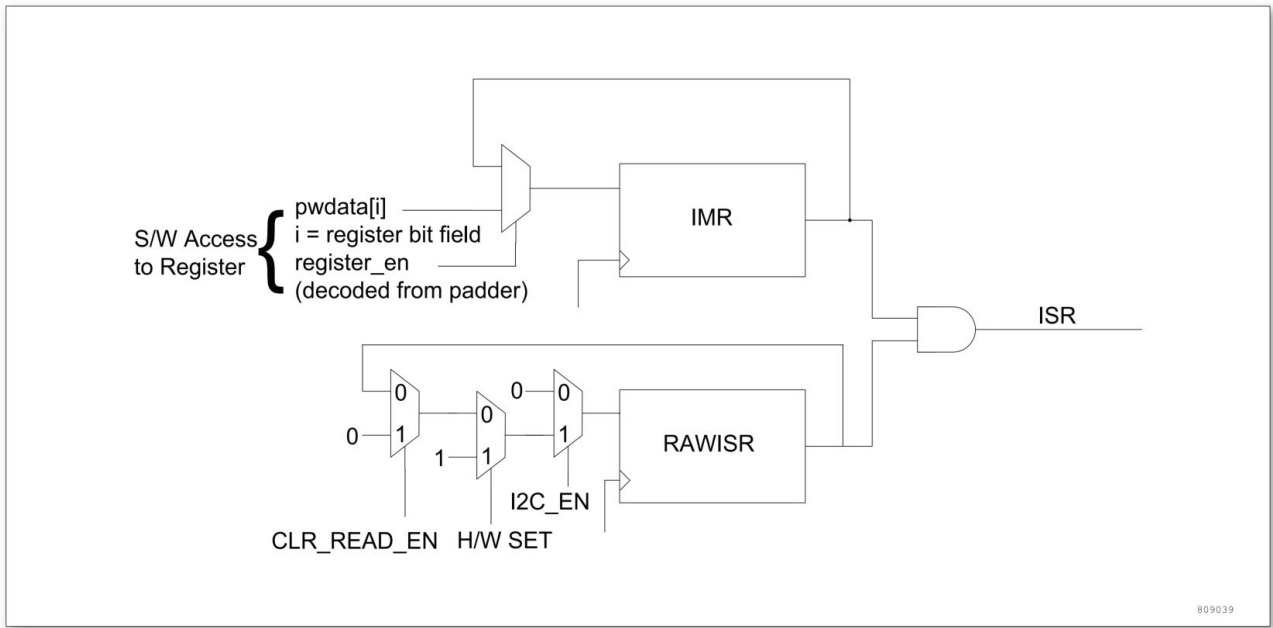
图 19-14 I2C 中断机制
