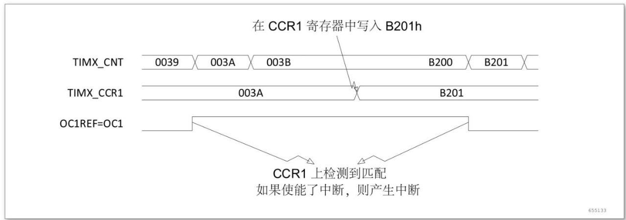
图 15-15 输出比较模式, 翻转 OC1
