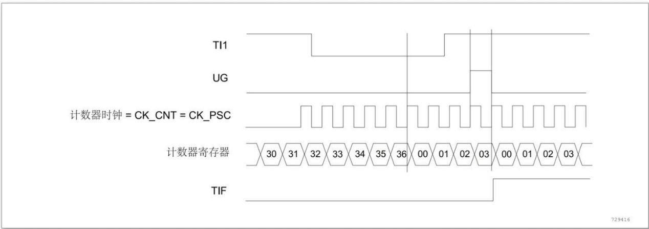
图 12-37 复位模式下的控制电路
