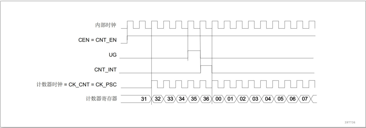
图 11-22 一般模式下的控制电路，内部时钟分频因子为 1
