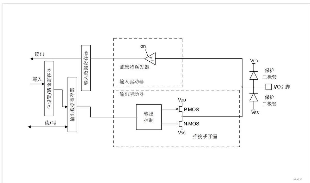
图 6-3 输出配置
