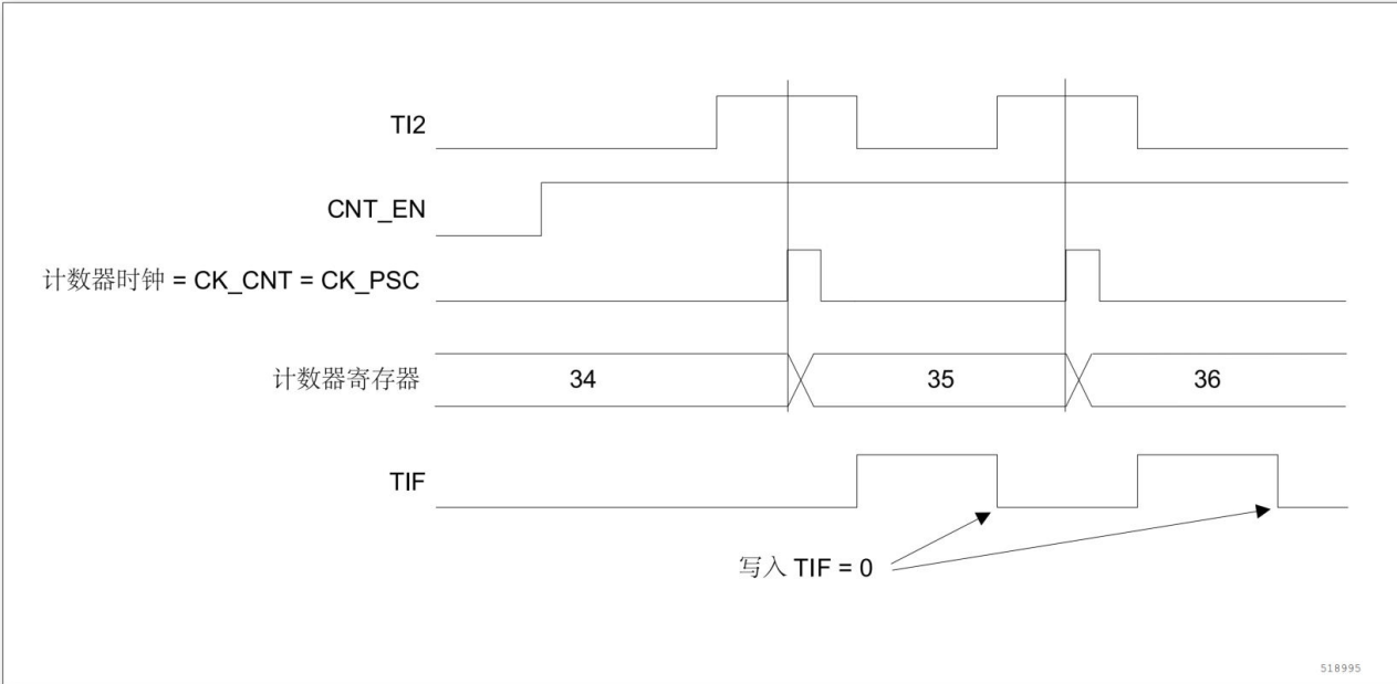
图 13-23 外部时钟模式 1 下的控制电路
