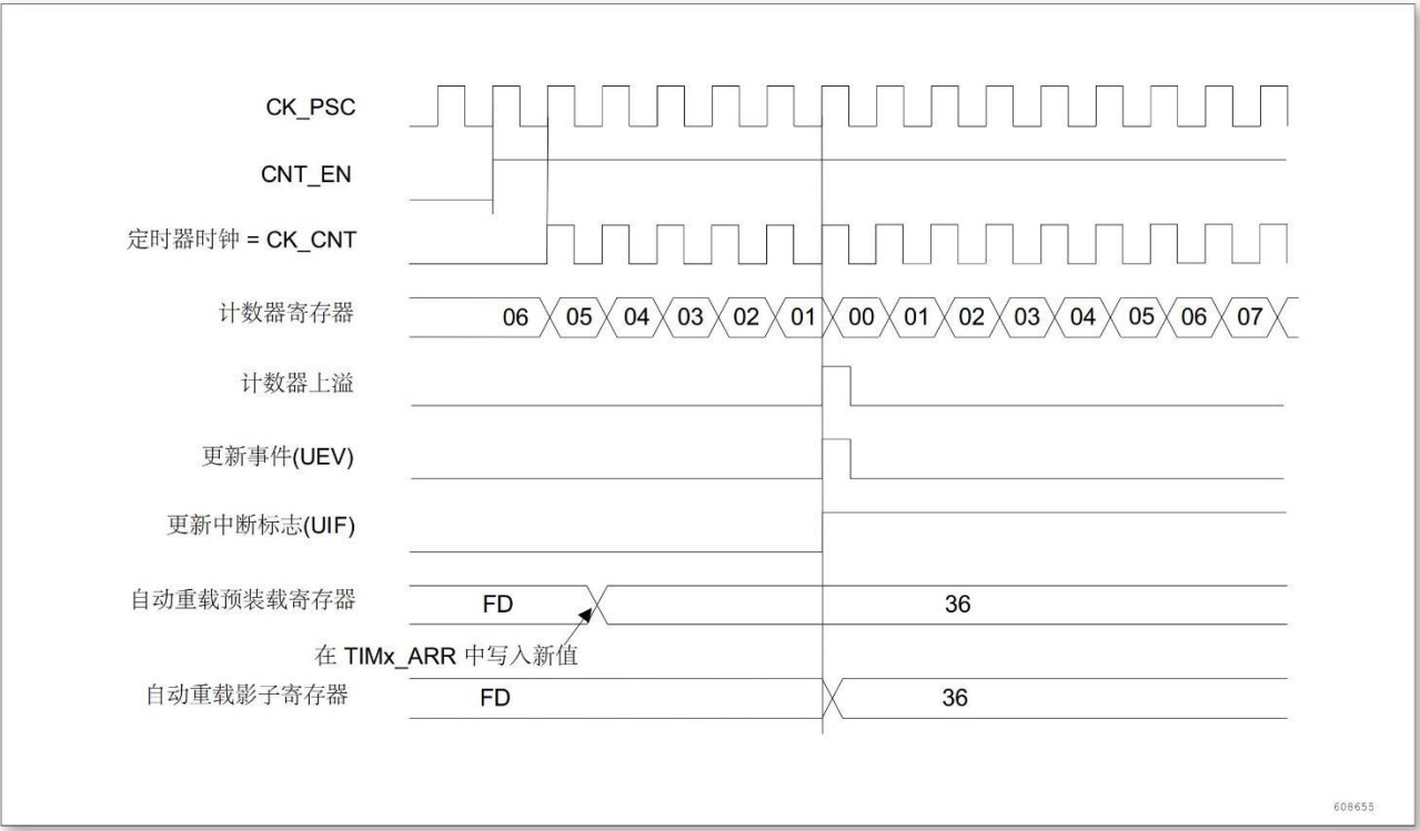
图 11-19 计数器时序图， ARPE = 1 时的更新事件 (计数器下溢)
