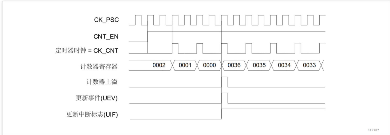
图 13-11 计数器时序图，内部时钟分频因子为 2
