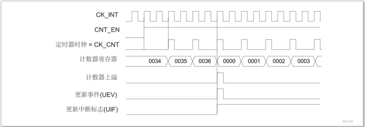
图 15-5 计数器时序图，内部时钟分频因子为 2
