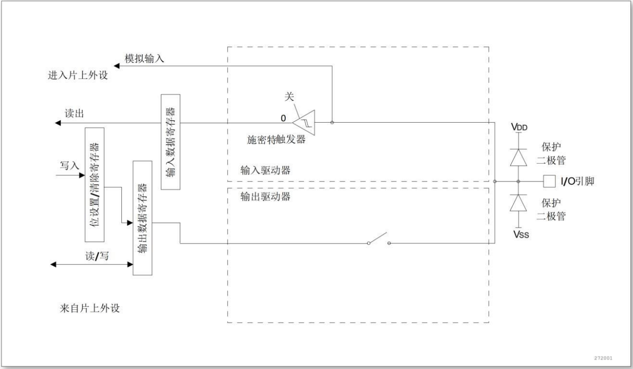
图 6-5 高阻抗的模拟输入配置
