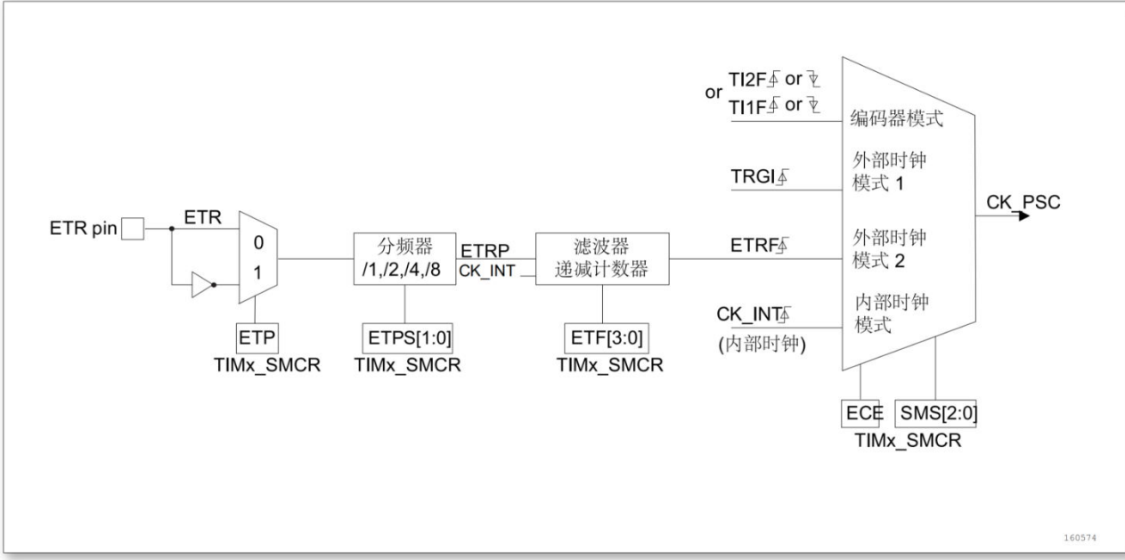
图 11-25 外部触发输入框图
