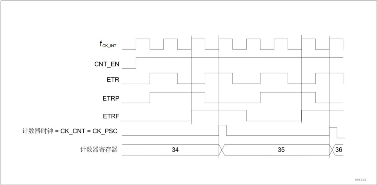
图 11-26 外部时钟模式 2 下的控制电路
