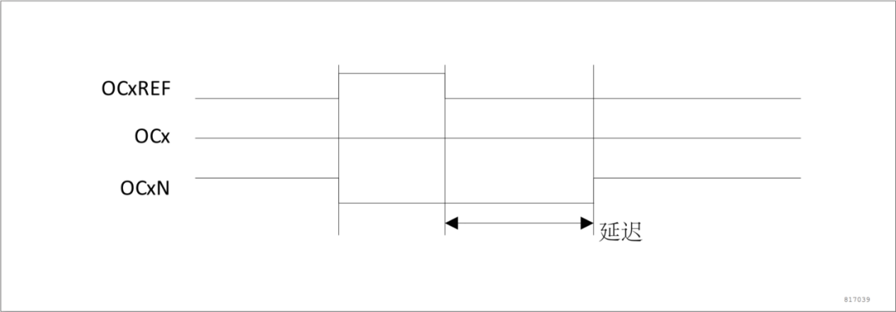
图 15-19 死区波形延迟大于正脉冲
