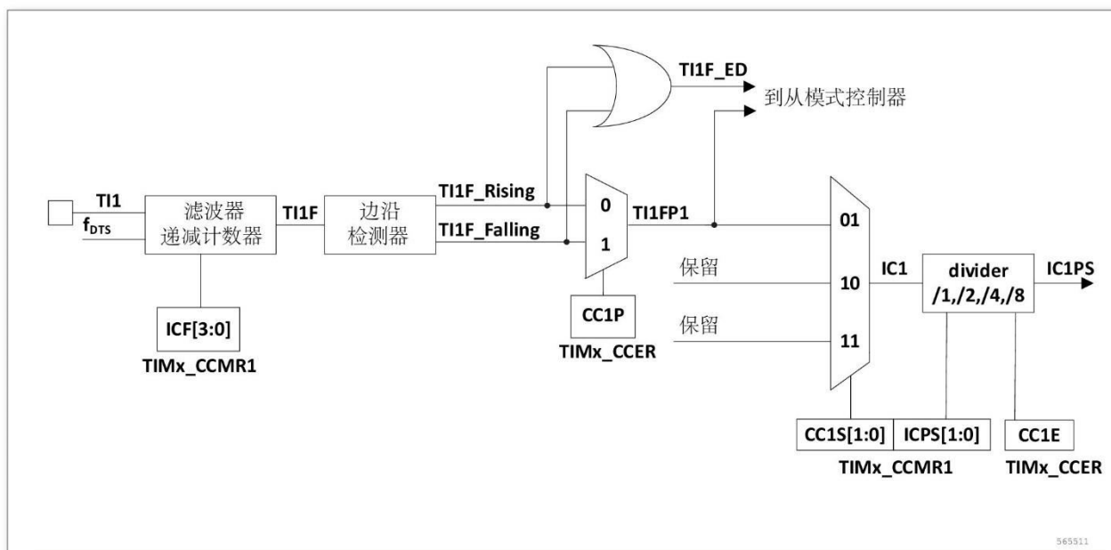
图 14-12 捕获/比较通道 (如: 通道 1 输入部分)
