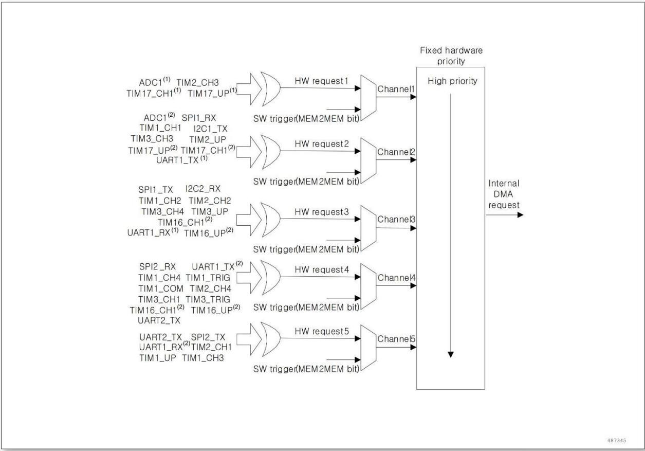
图 8-2 外设 DMA 请求映射
