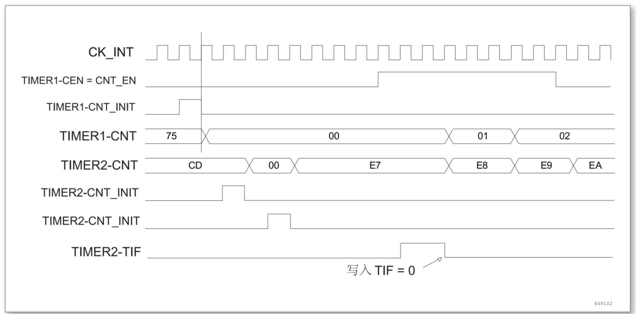
图 13-45 利用定时器 1 的使能触发定时器 2
