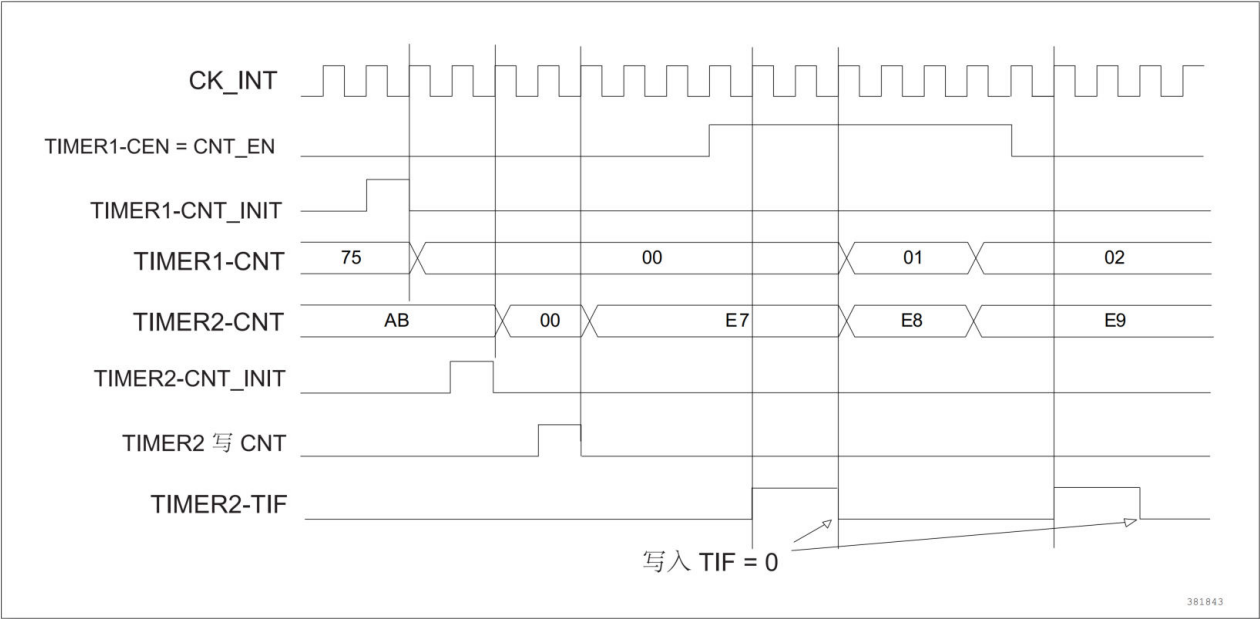
图 13-43 通过使能定时器 1 可以控制定时器 2
