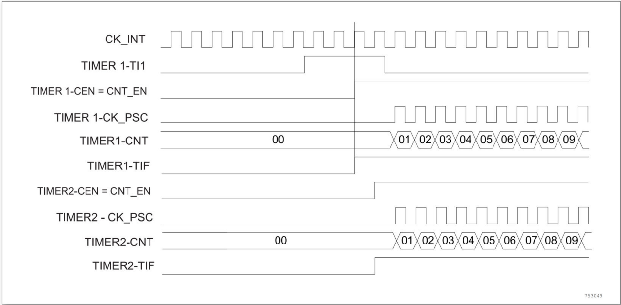
图 13-46 使用定时器 1 的 T1 输入触发定时器 1 和定时器 2
