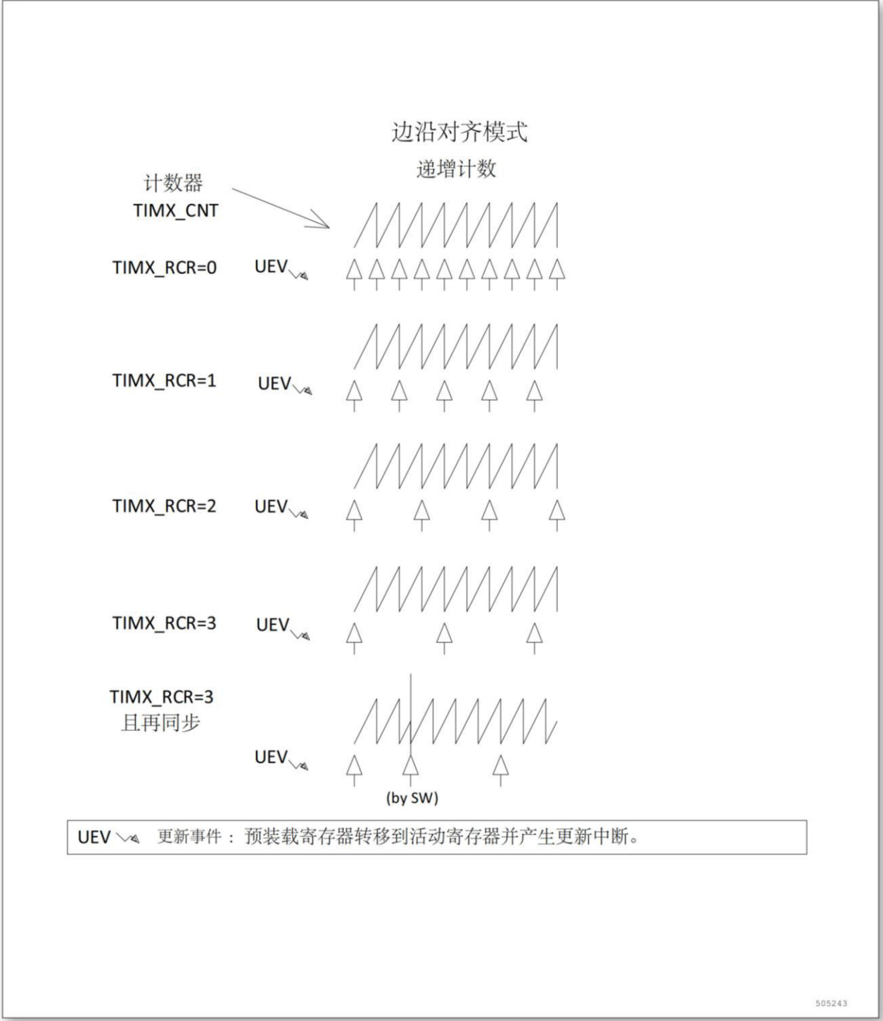
图 14-10 不同模式及不同 TIMx_RCR 寄存器设置下更新速率的例子
