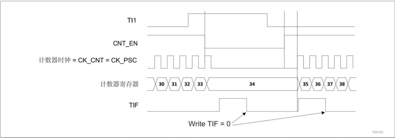
图 12-38 门控模式下的控制电路
