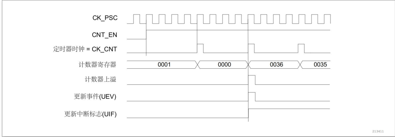
图 13-12 计数器时序图，内部时钟分频因子为 4
