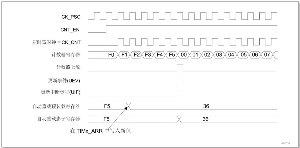
图 12-9 计数器时序图，当 ARPE = 1 时的更新事件 (预装入了 TIMx_ARR)
