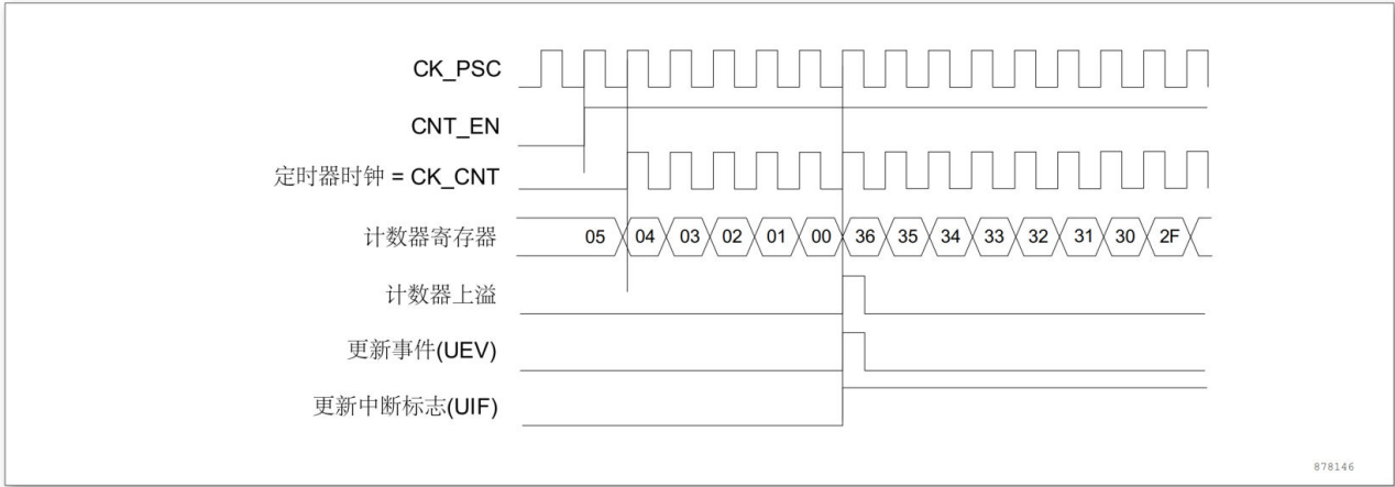
图 11-10 计数器时序图，内部时钟分频因子为 1
