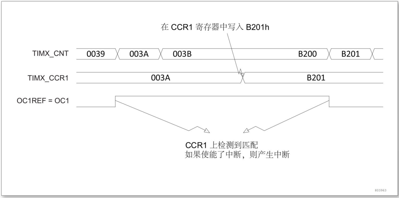
图 14-15 输出比较模式，翻转 OC1
