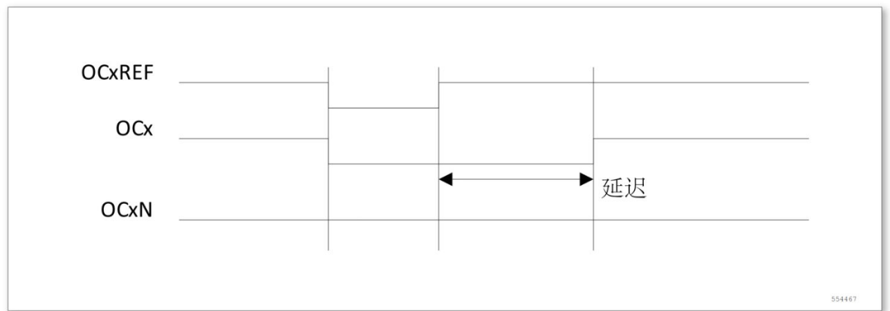
图 15-18 死区波形延迟大于负脉冲
