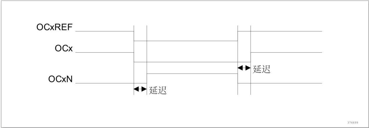
图 11-36 带死区插入的互补输出
