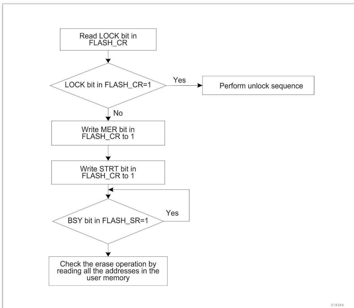
图 2-3 Flash 寄存器整片擦除流程
