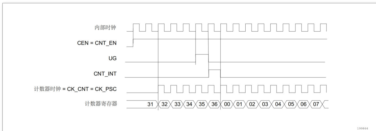
图 14-11 一般模式下的控制电路，内部时钟分频因子为 1
