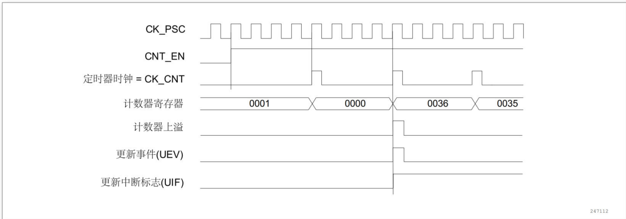
图 11-12 计数器时序图，内部时钟分频因子为 4
