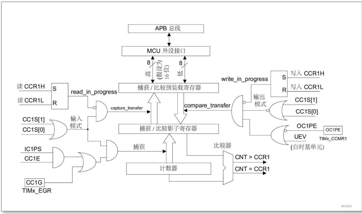
图 14-13 捕获/比较通道 1 的主电路
