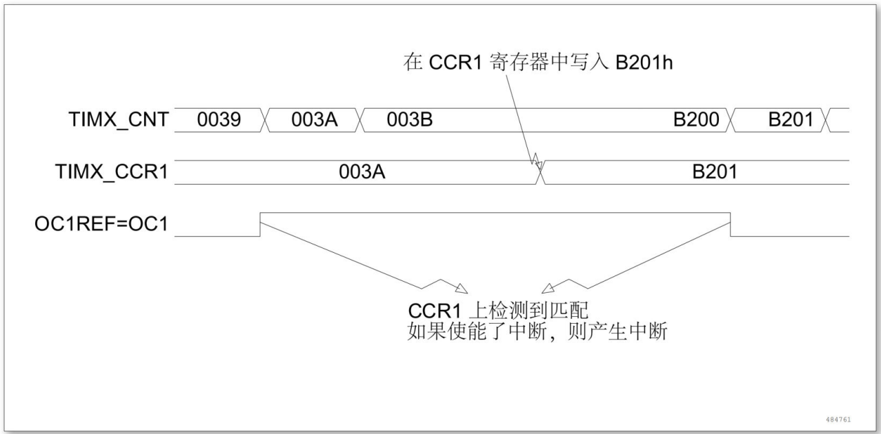
图 11-32 输出比较模式，翻转 OC1
