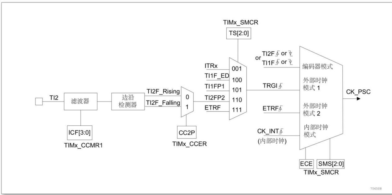
图 11-23 TI2 外部时钟连接例子
