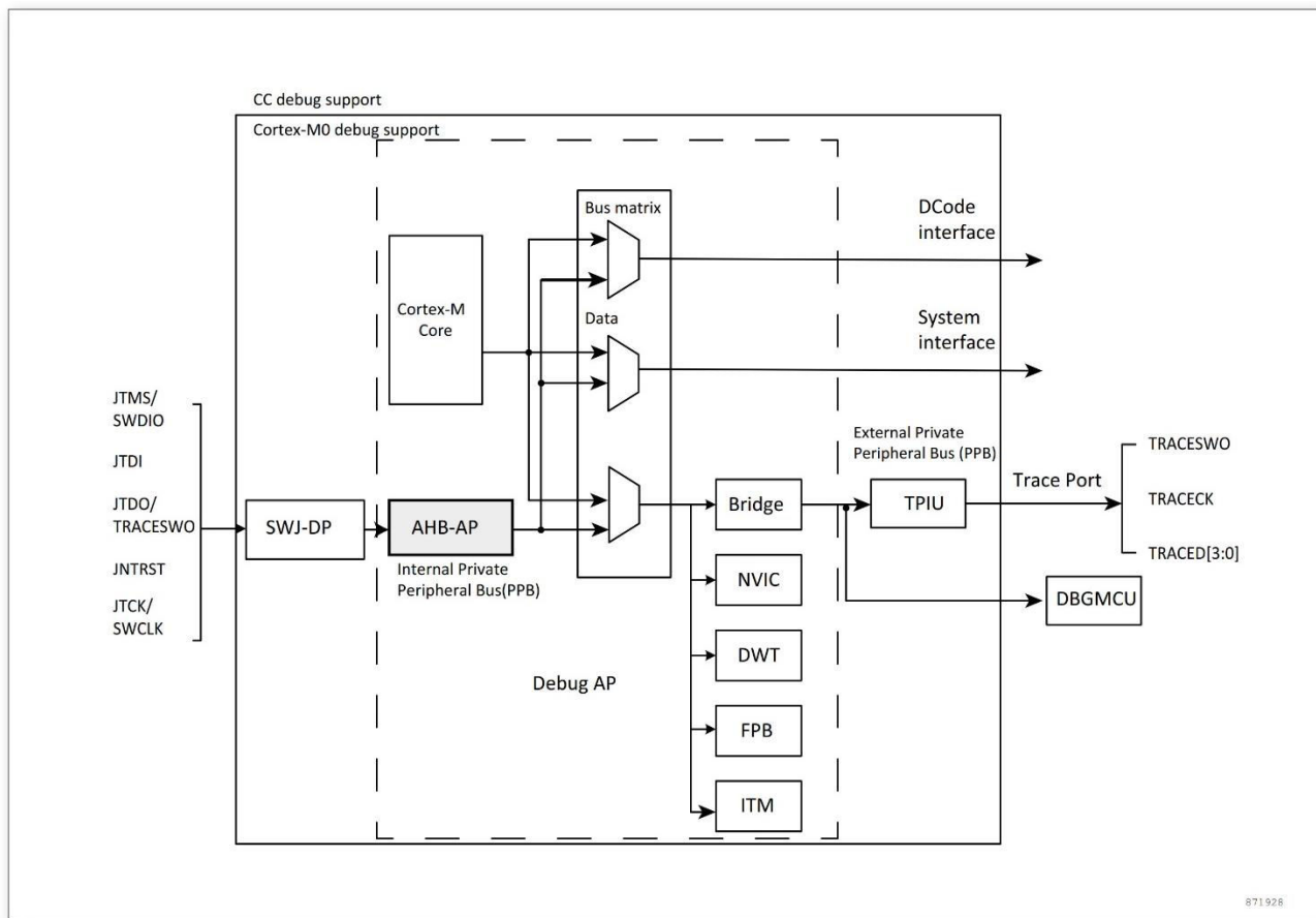
图 24-1 MM32 系列级别和 CPU 级别的调试框
