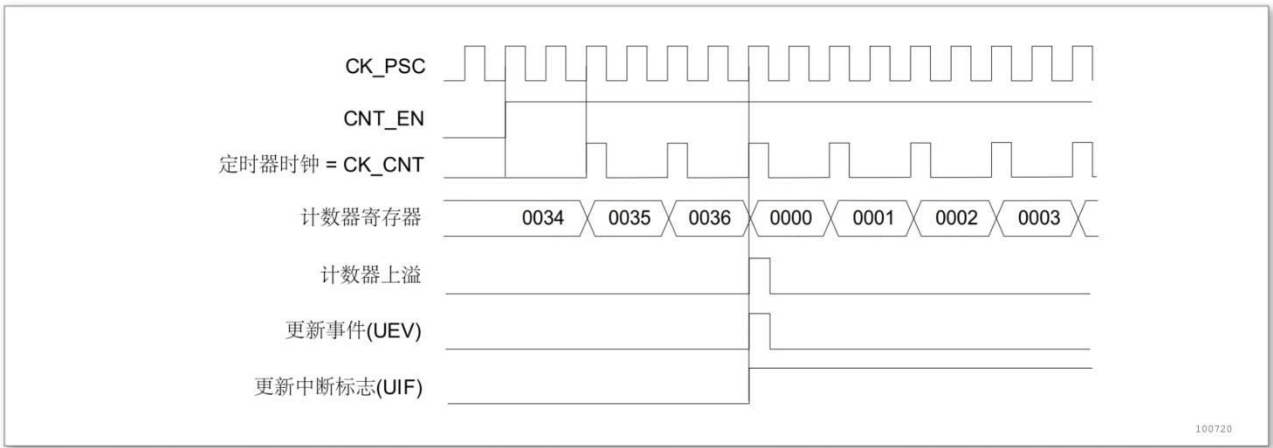
图 12-5 计数器时序图，内部时钟分频因子为 2
