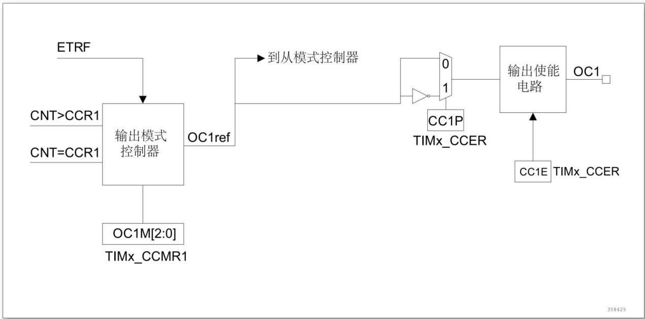
图 13-28 捕获/比较通道的输出部分 (通道 1)
