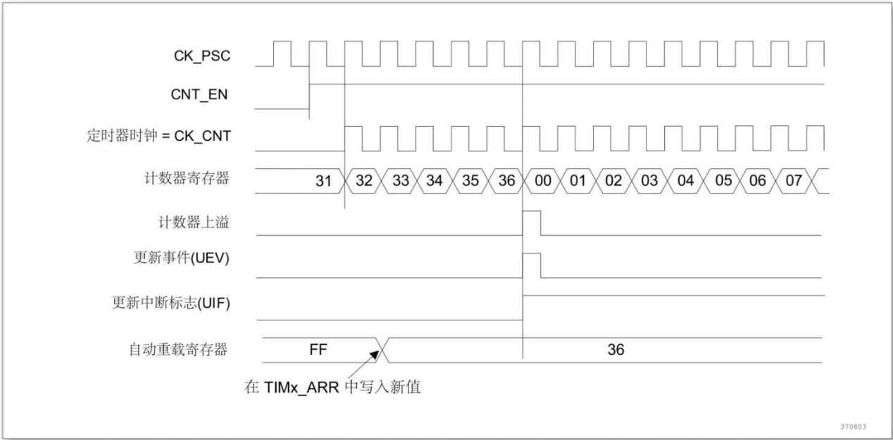
图 12-8 计数器时序图，当 ARPE = 0 时的更新事件 (TIMx_ARR 没有预装入)
