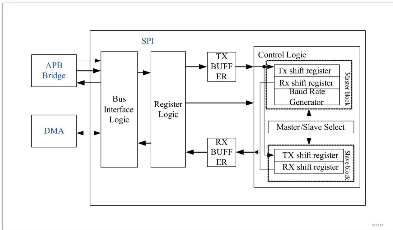
图 18-1 SPI 框图
