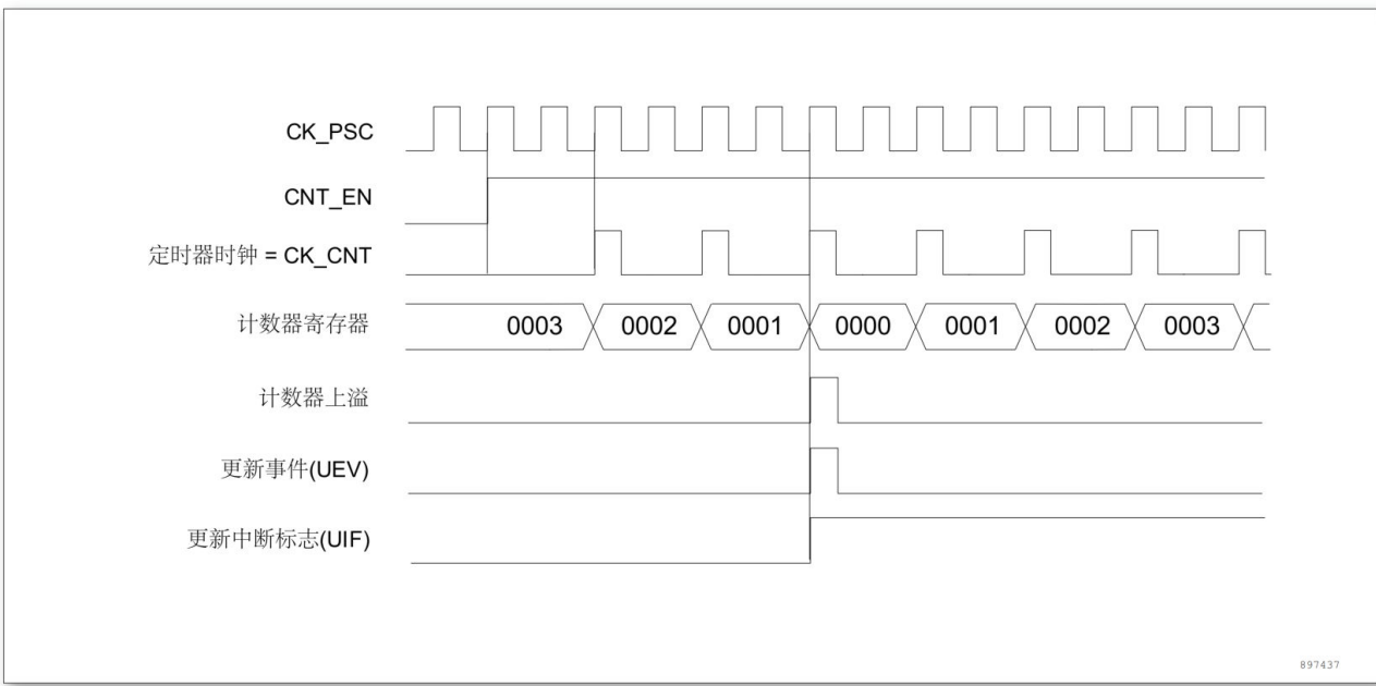
图 11-16 计数器时序图，内部时钟分频因子为 2
