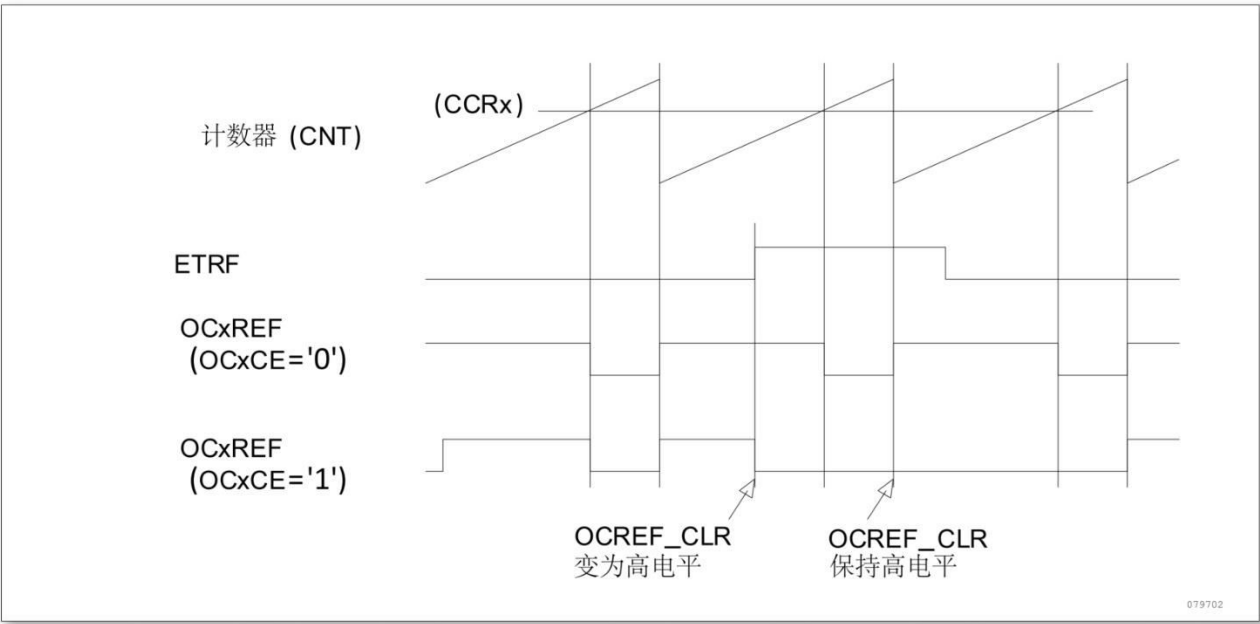
图 12-34 清除 TIMx 的 OCxREF
