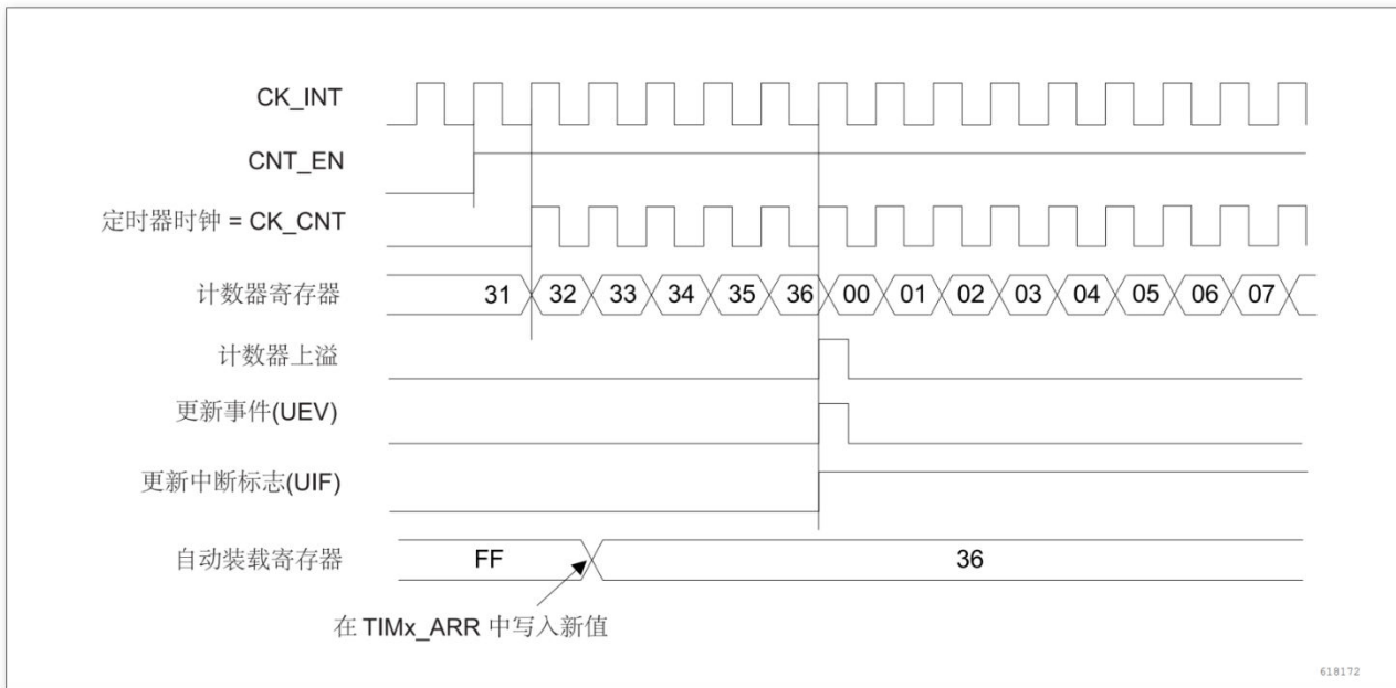
图 15-8 计数器时序图，当 ARPE=0 时的更新事件(TIMX ARR 没有预装载)
