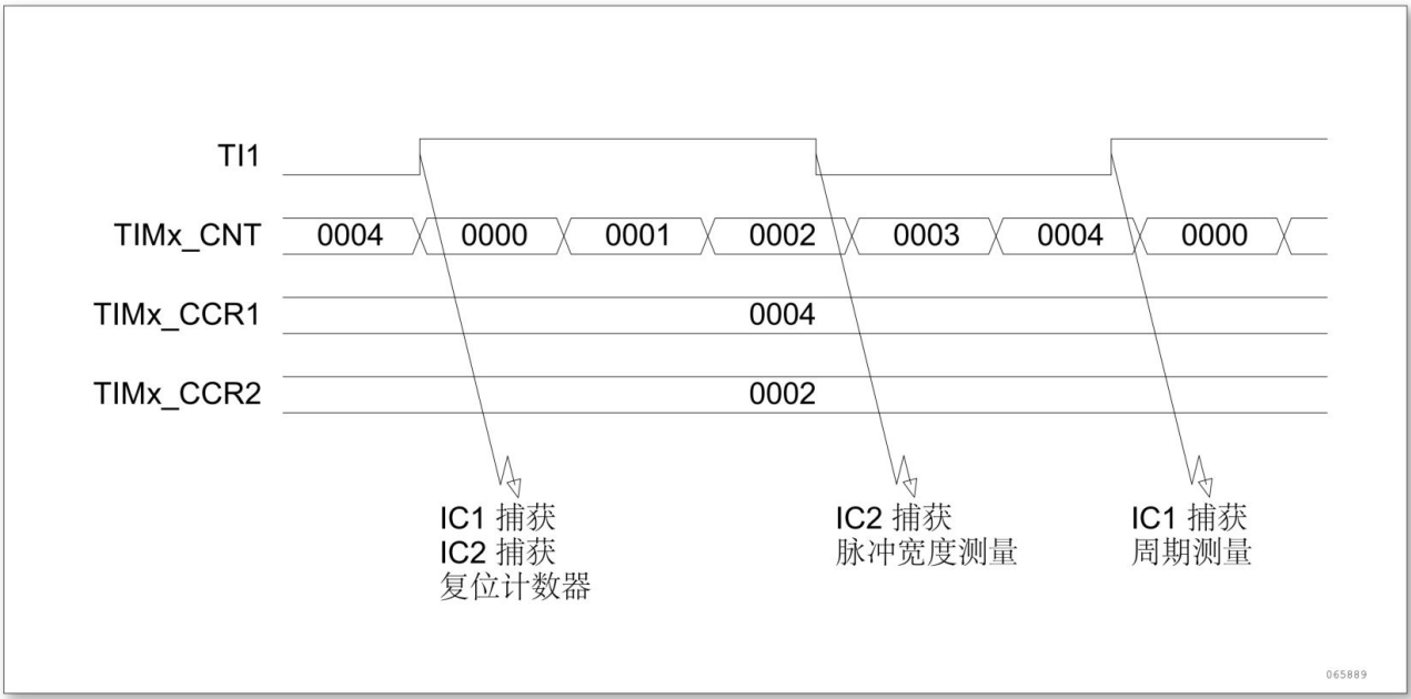
图 11-31 PWM 输入模式时序
