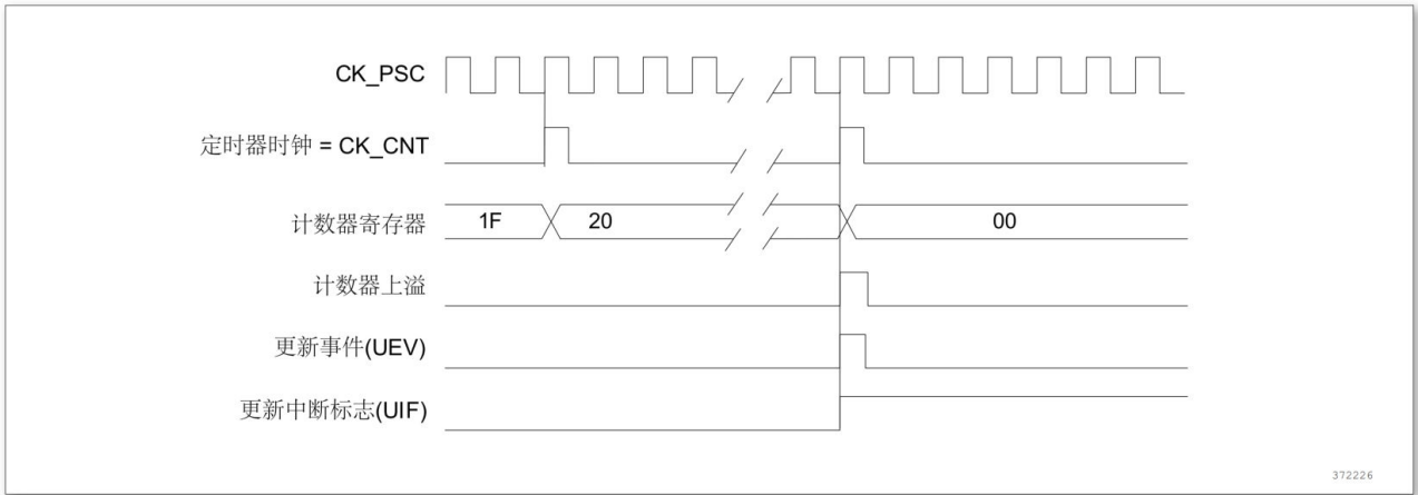
图 14-7 计数器时序图，内部时钟分频因子为 N
