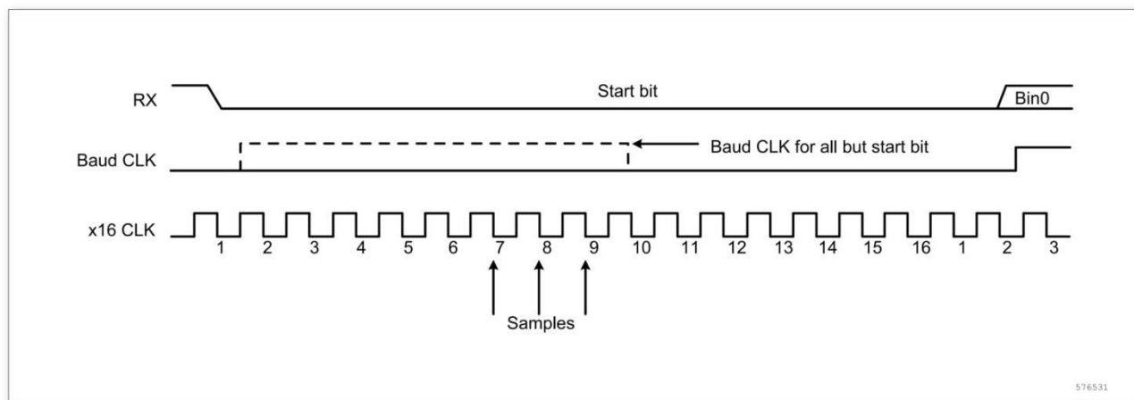
图 20-6 RX 引脚采样方案
