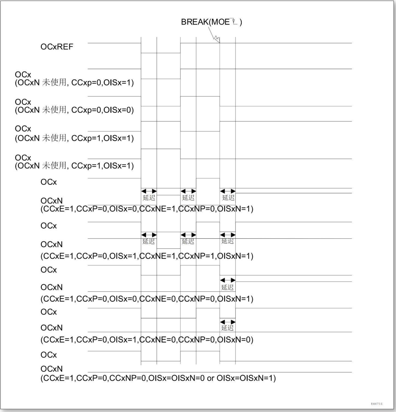
图 11-39 响应刹车的输出
