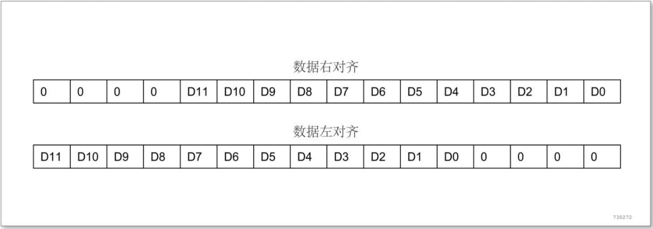
图 9-7 数据对齐方式
