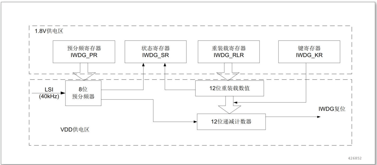
图 16-1 独立看门狗框图
