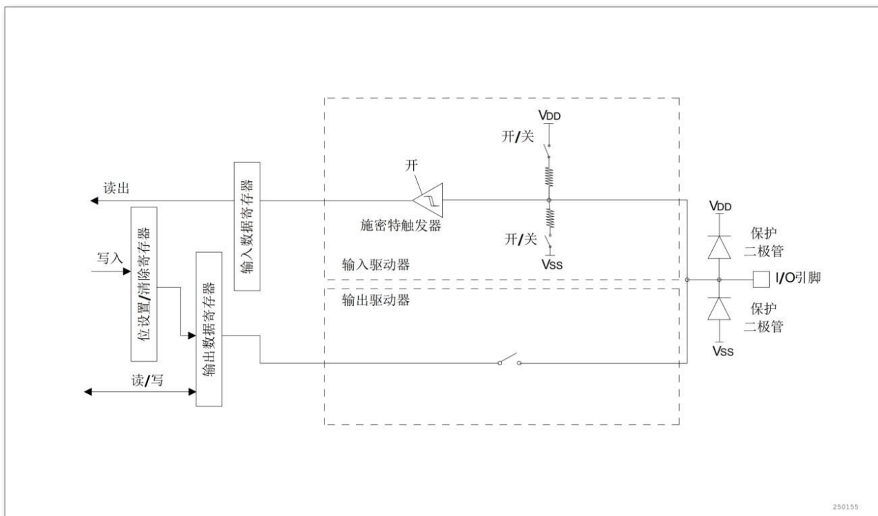
图 6-2 输入浮空/上拉/下拉配置
