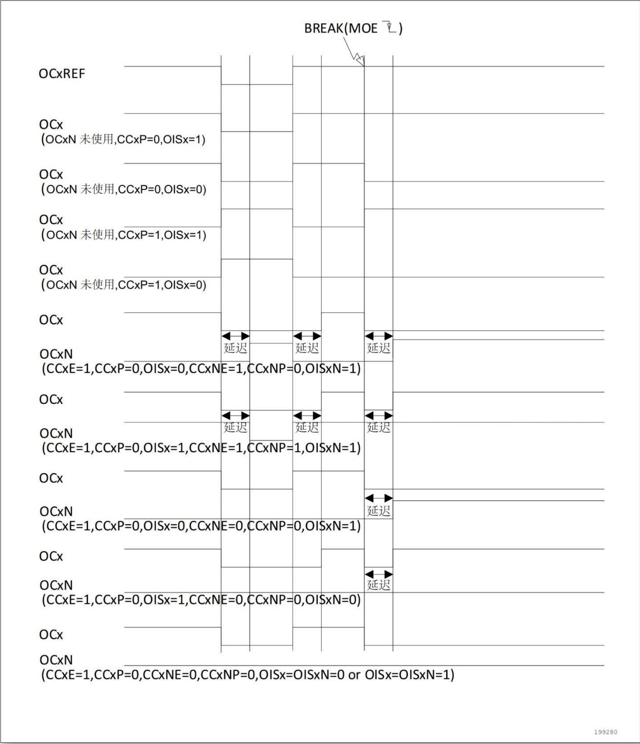
图 15-20 响应刹车的输出
