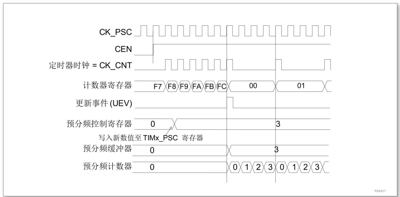
图 15-3 当预分频器的参数从 1 变到 4 时，计数器的时序图
