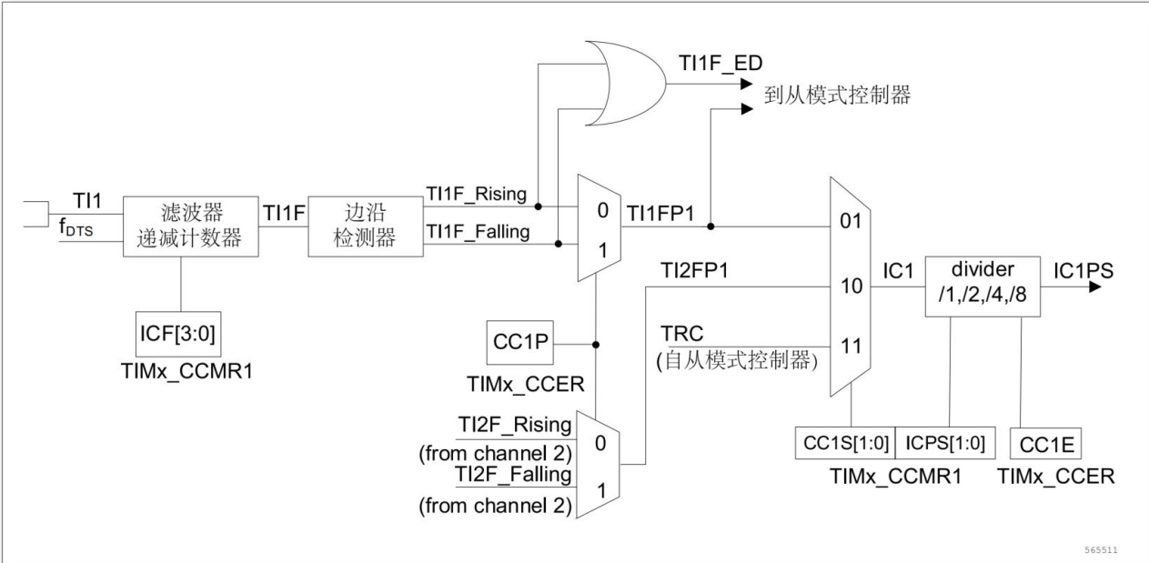
图 13-26 捕获/比较通道 (如: 通道 1 输入部分)
