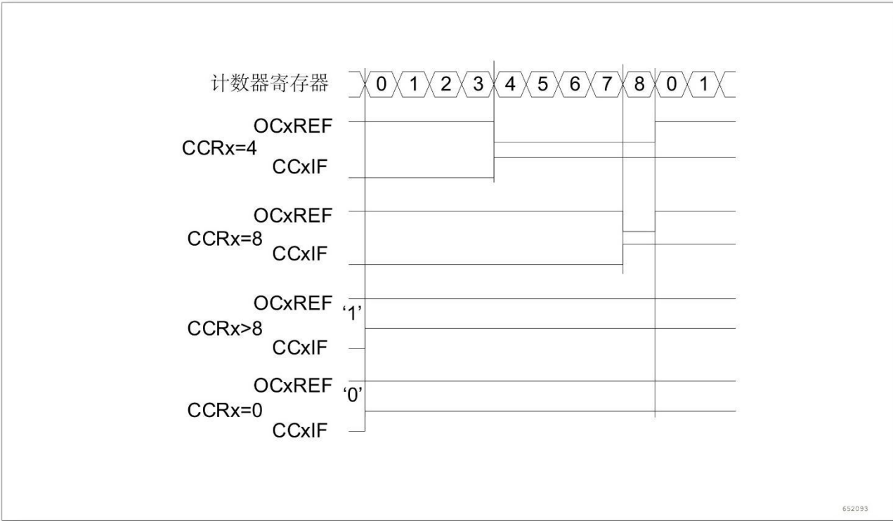
图 11-33 边沿对齐的 PWM 波形 (ARR = 8)
