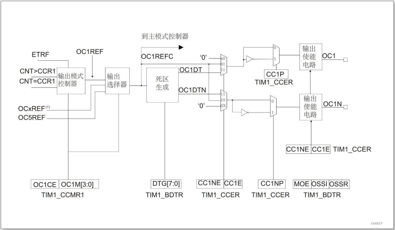
图 15-14 捕获/比较通道的输出部分（通道 1）
