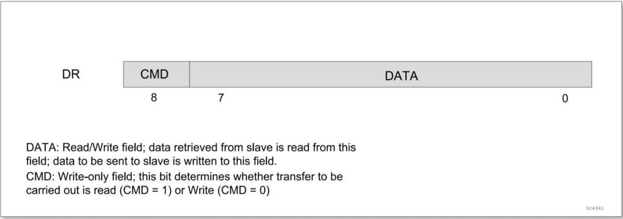
图 19-7 DR 寄存器
