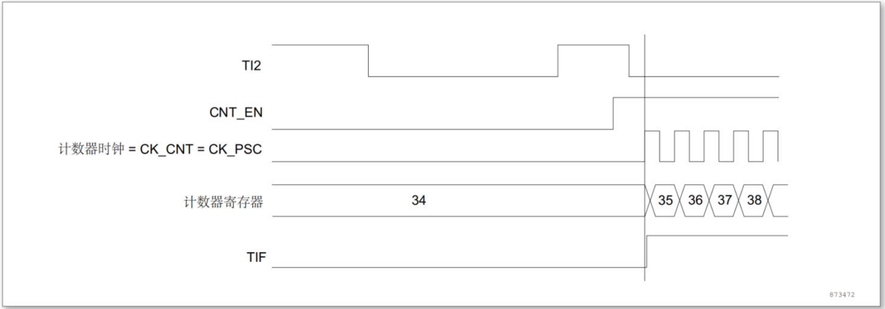
图 11-48 触发器模式下的控制电路
