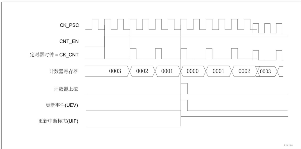
图 13-16 计数器时序图，内部时钟分频因子为 2
