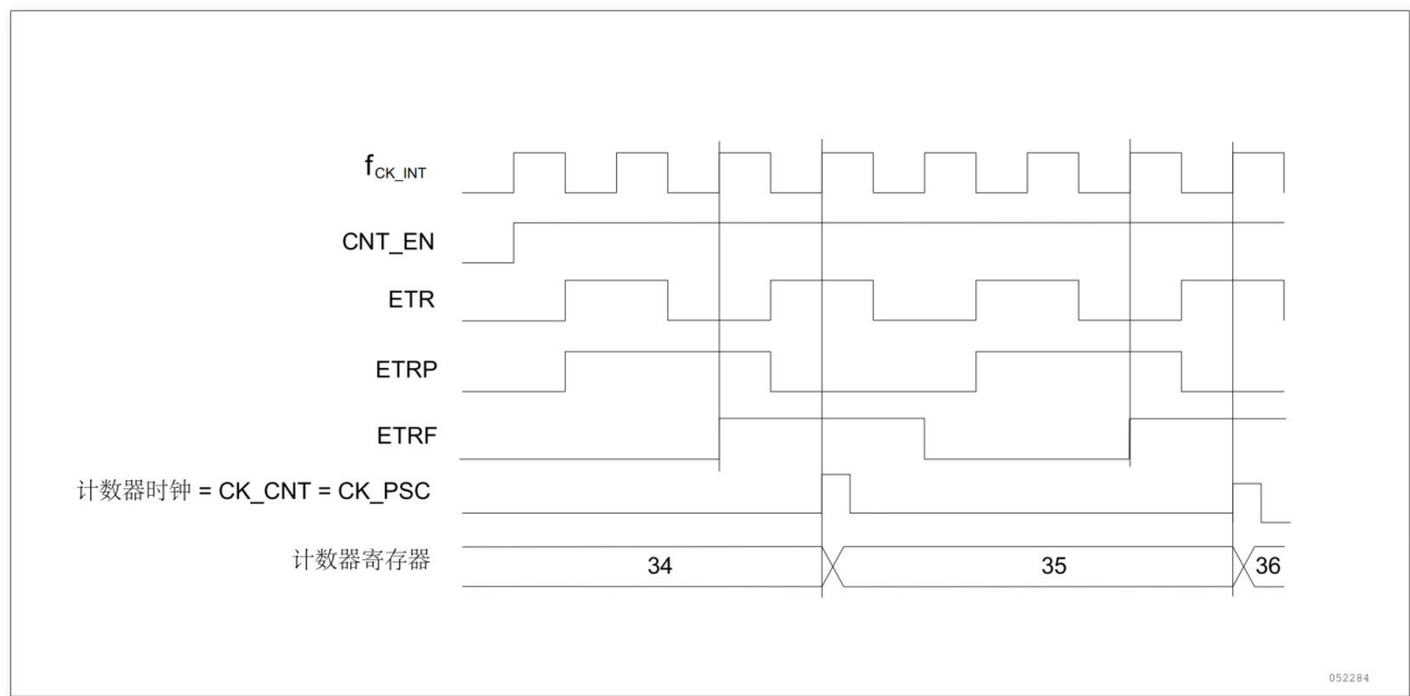
图 13-25 外部时钟模式 2 下的控制电路
