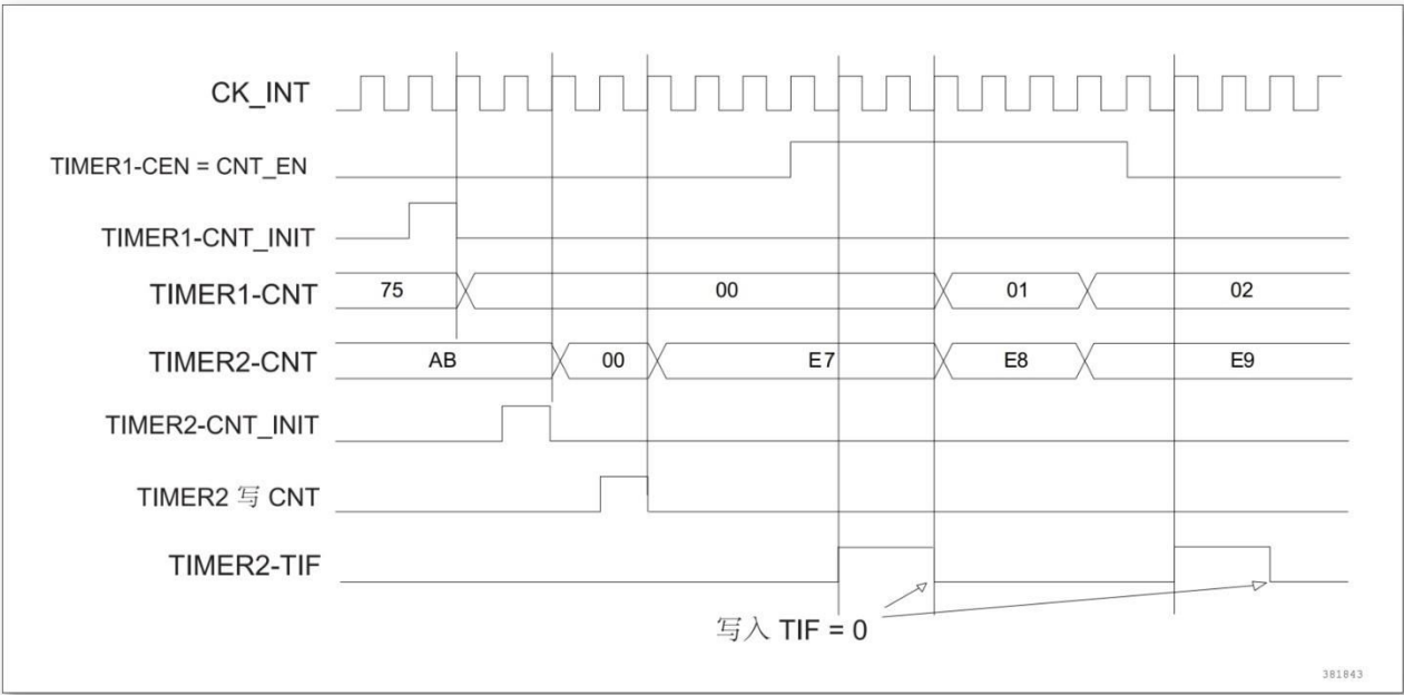
图 12-43 通过使能定时器 1 可以控制定时器 2
