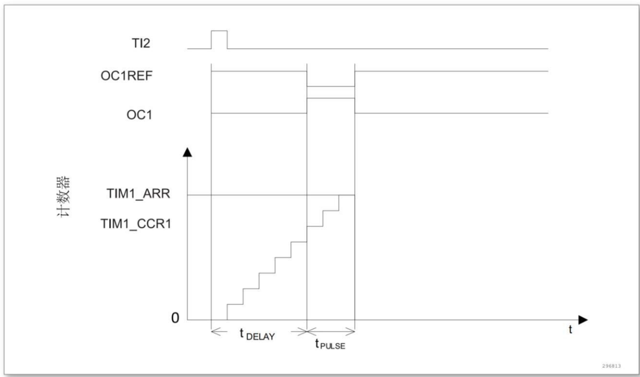
图 13-33 单脉冲模式的例子
