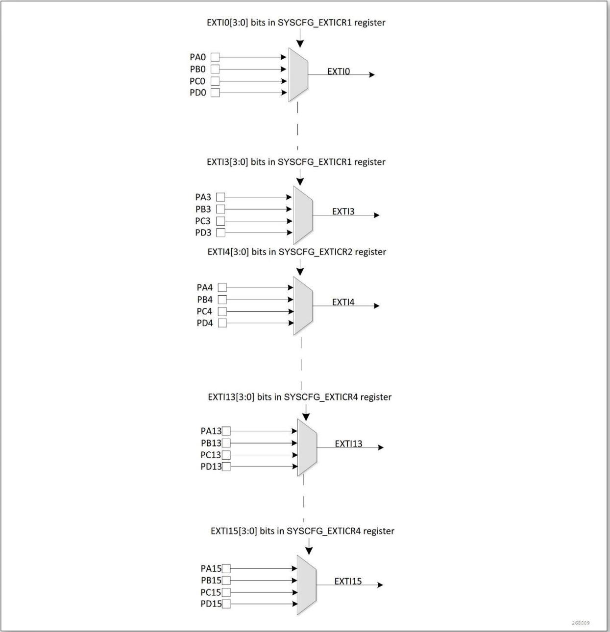
图 7-2 外部中断通用 I/O 映像
