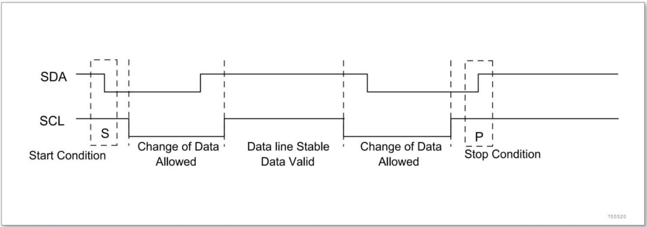
图 19-1 起始和停止条件
