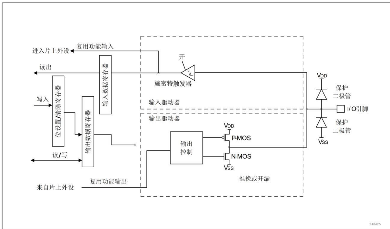
图 6-4 复用功能配置
