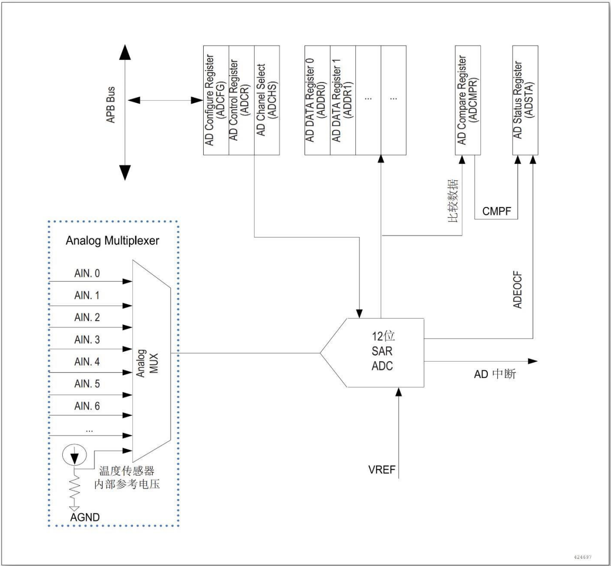
图 9-1 ADC 框图
