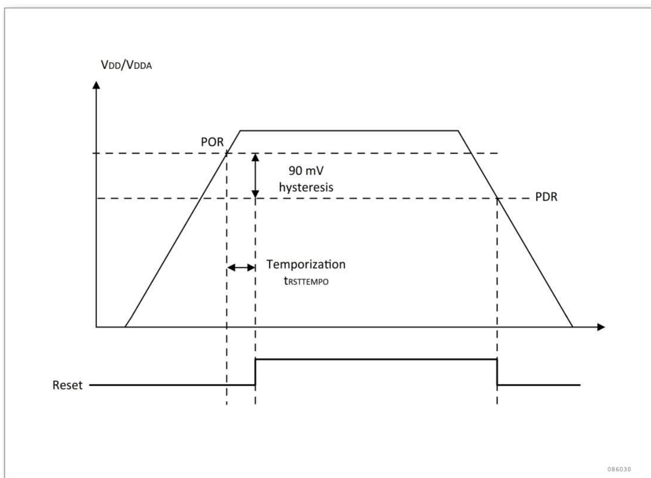
图 4-2 上电复位和掉电复位波形图
