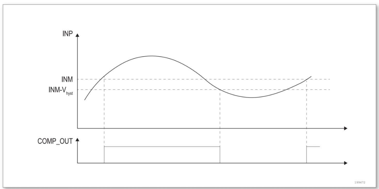
图 10-2 比较器的迟滞现象
