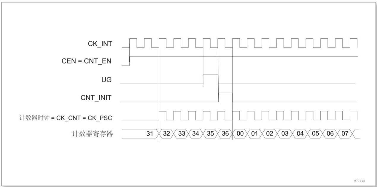
图 15-11 一般模式下的控制电路，内部时钟分频因子为 1
