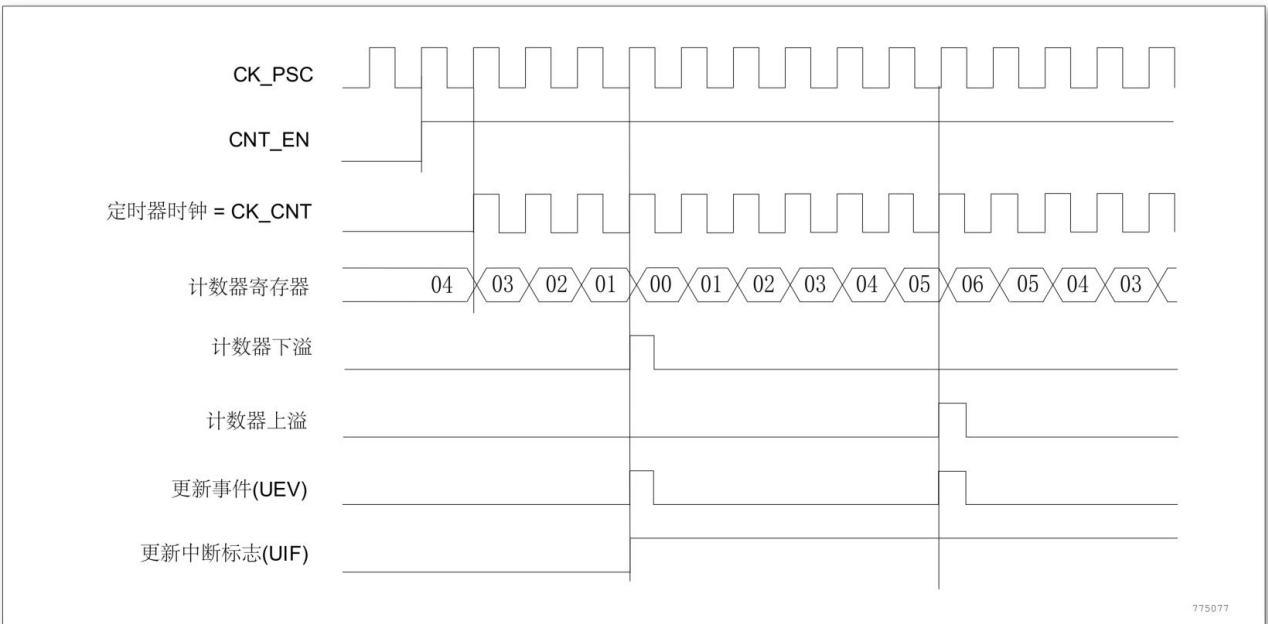
图 13-15 计数器时序图，内部时钟分频因子为 1，TIMx_ARR = 0x6
