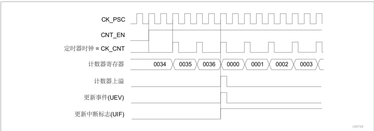
图 13-5 计数器时序图，内部时钟分频因子为 2
