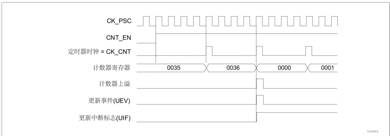
图 13-6 计数器时序图，内部时钟分频因子为 4
