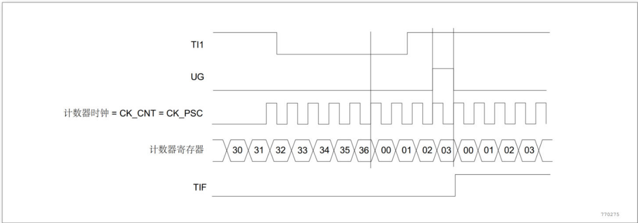
图 11-46 复位模式下的控制电路
