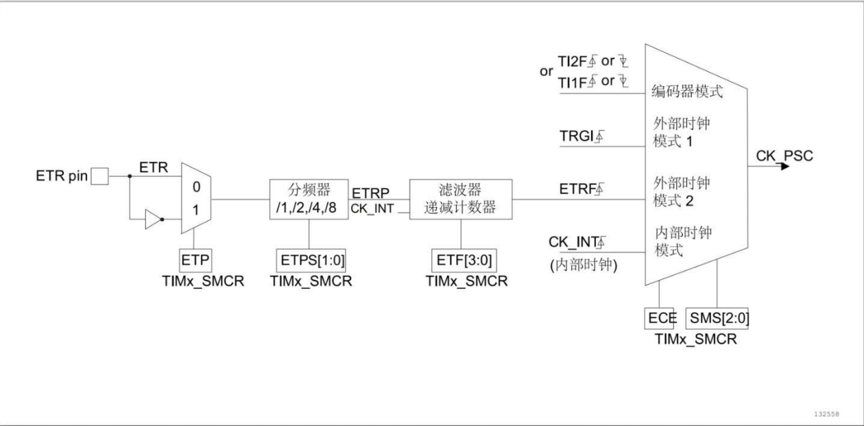
图 12-24 外部触发输入框图
