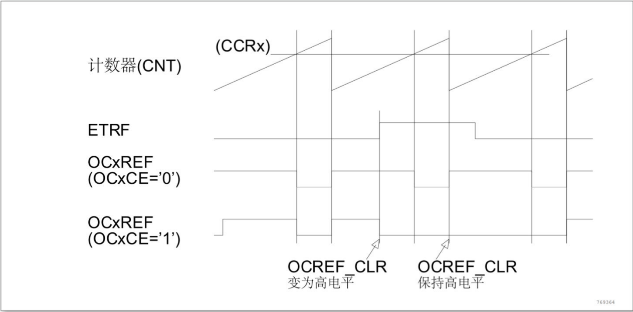
图 11-40 清除 TIMx 的 OCxREF
