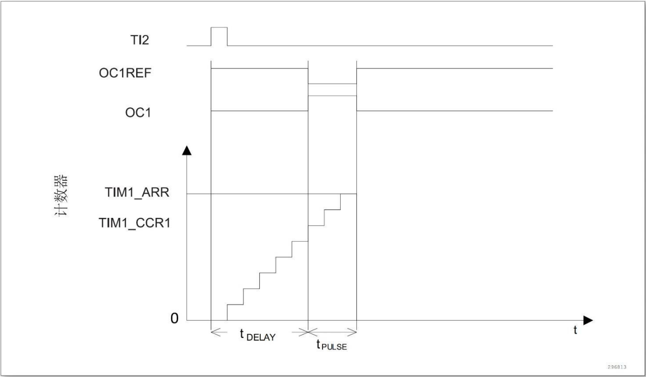
图 12-33 单脉冲模式的例子
