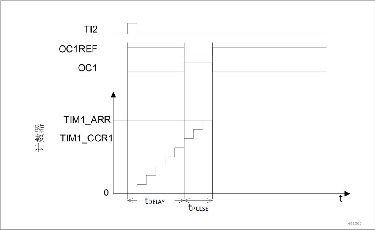
图 15-21 单脉冲模式的例子
