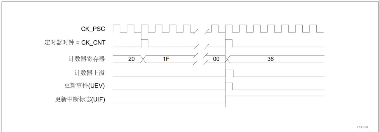
图 13-13 计数器时序图，内部时钟分频因子为 N
