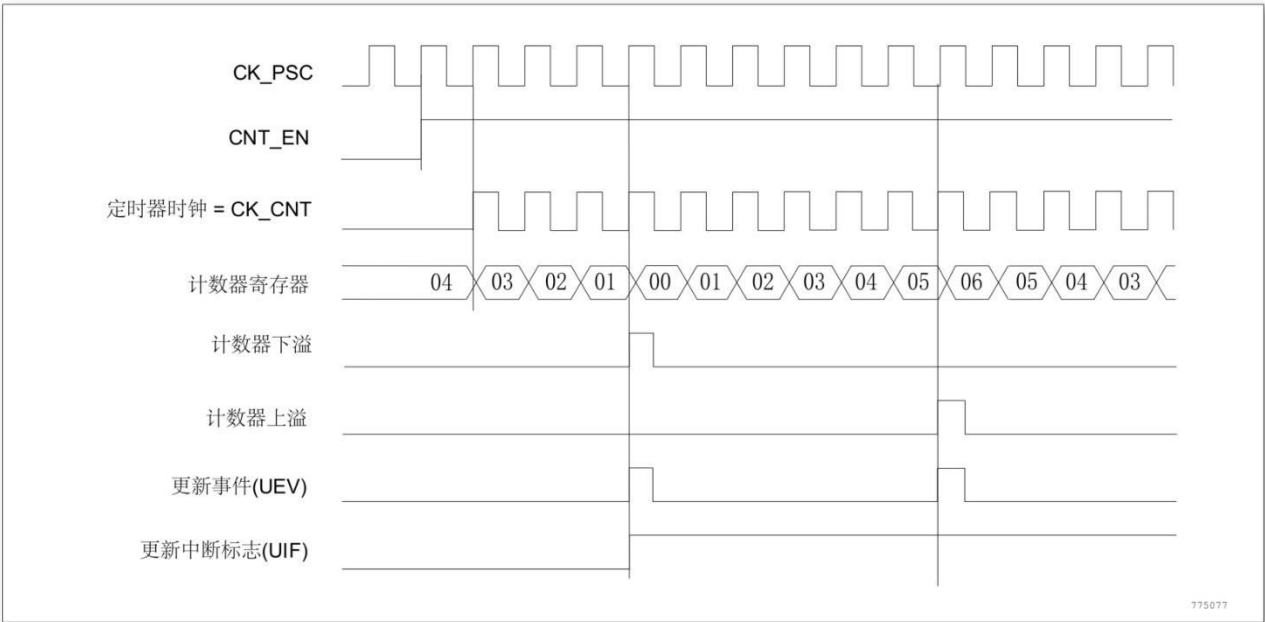
图 12-15 计数器时序图，内部时钟分频因子为 1，TIMx_ARR = 0x06
