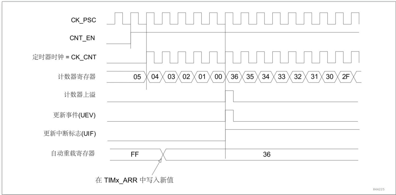
图 11-14 计数器时序图，当没有使用重复计数器时的更新事件
