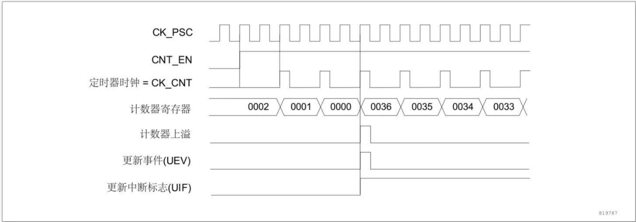
图 12-11 计数器时序图，内部时钟分频因子为 2
