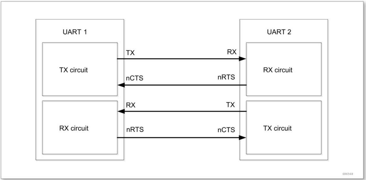
图 20-7 两个 UART 间的硬件流控制
