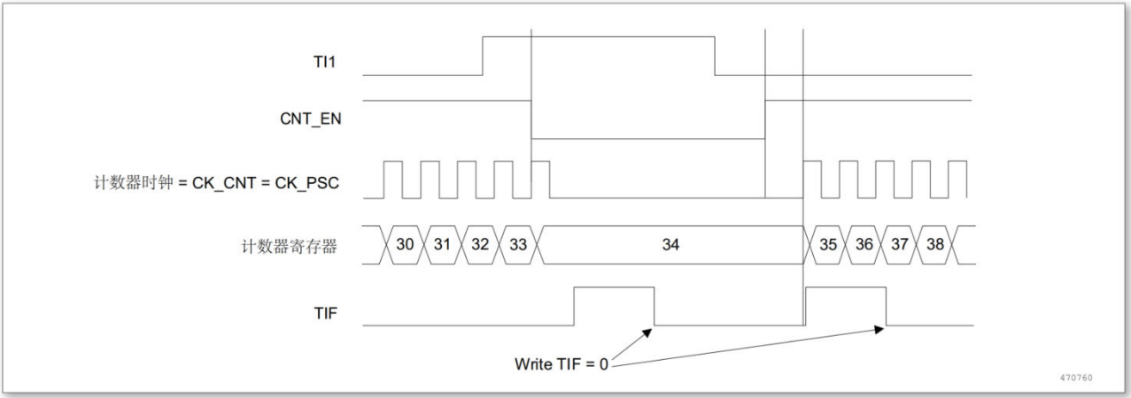
图 11-47 门控模式下的控制电路
