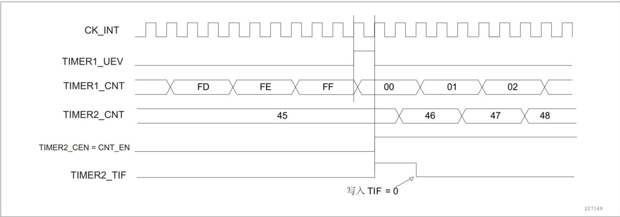
图 13-44 使用定时器 1 的更新触发定时器 2
