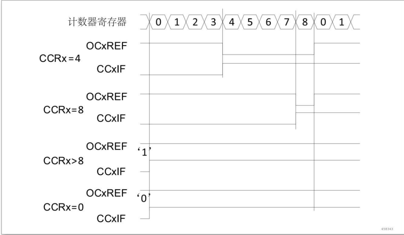
图 14-16 边沿对齐的 PWM 波形 (ARR = 8)
