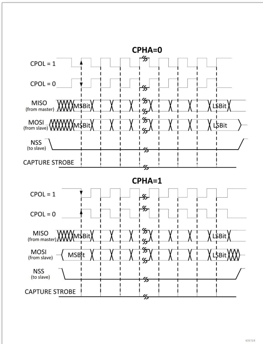
图 18-3 数据时钟时序图
