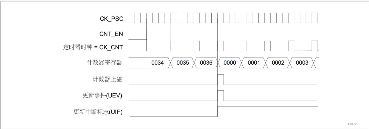
图 14-5 计数器时序图，内部时钟分频因子为 2
