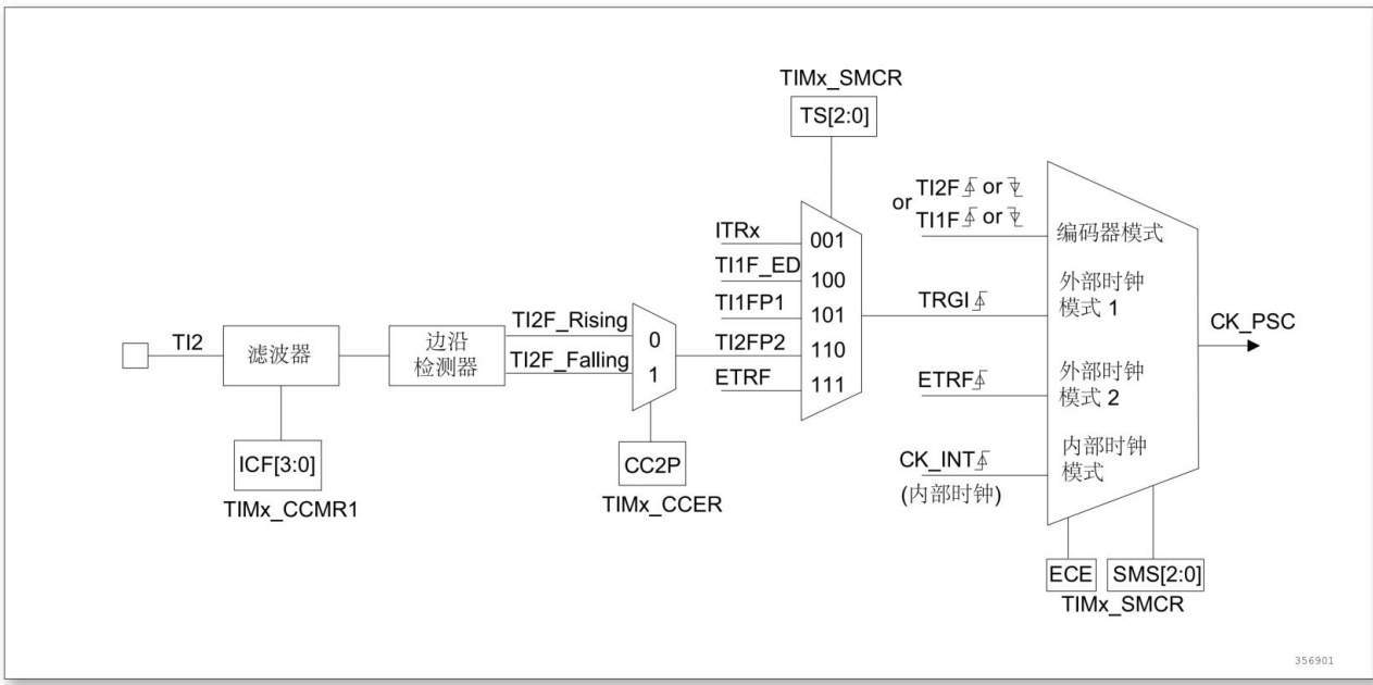
图 13-22 TI2 外部时钟连接例子
