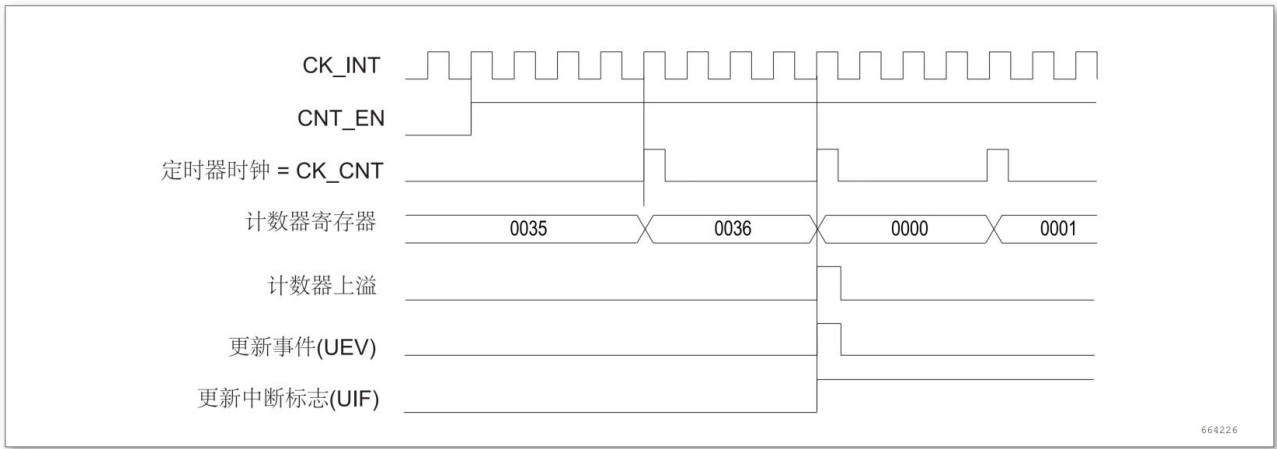
图 15-6 计数器时序图，内部时钟分频因子为 4
