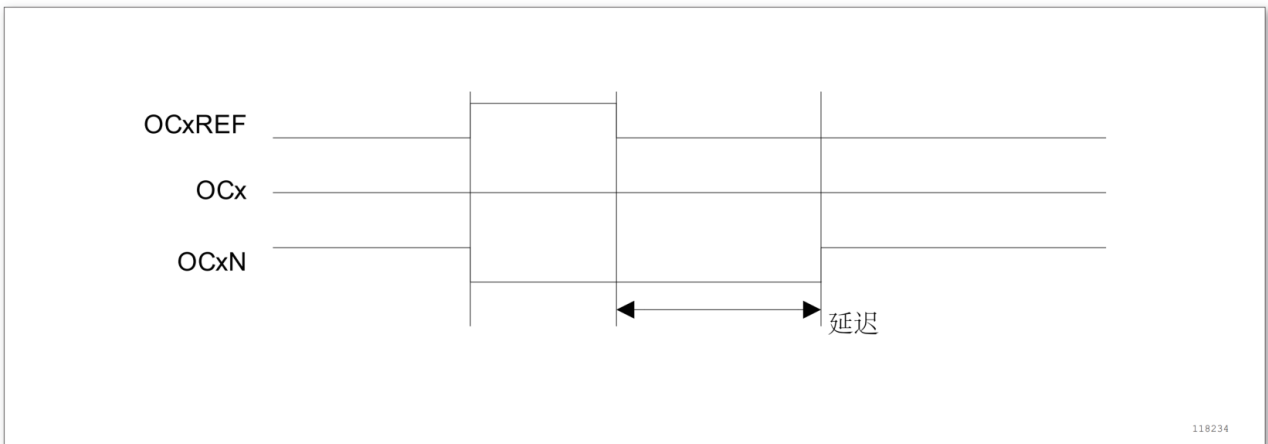
图 11-38 死区波形延迟大于正脉冲
