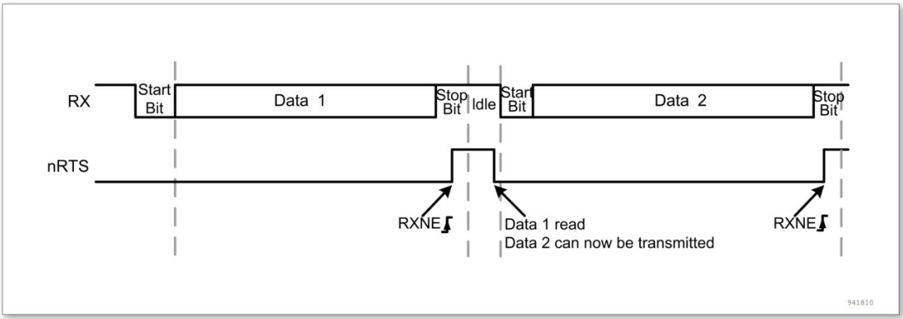
图 20-8 RTS 流控制
