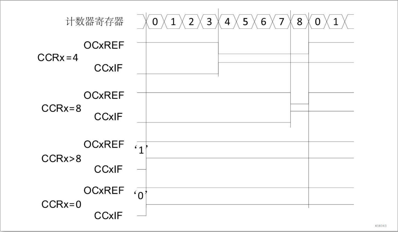
图 12-31 边沿对齐的 PWM 波形 (ARR = 8)
