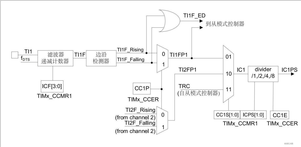
图 11-27 捕获/比较通道 (如: 通道 1 输入部分)
