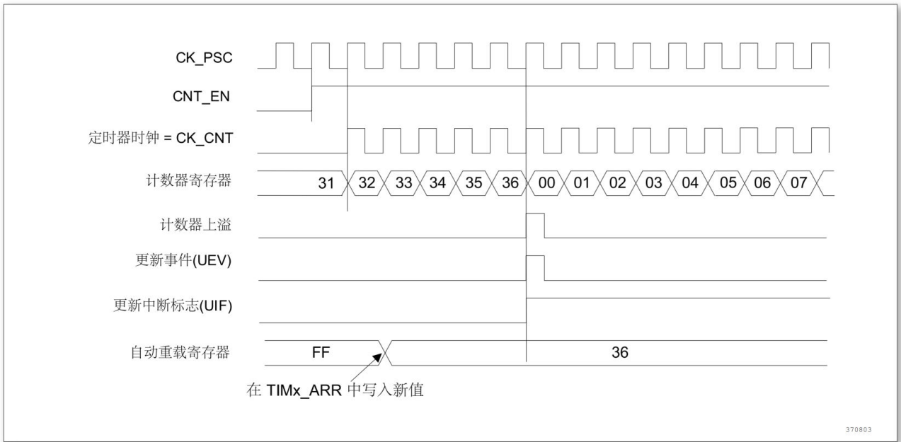
图 14-8 计数器时序图，当 ARPE = 0 时的更新事件 (TIM14_ARR 没有预装载)
