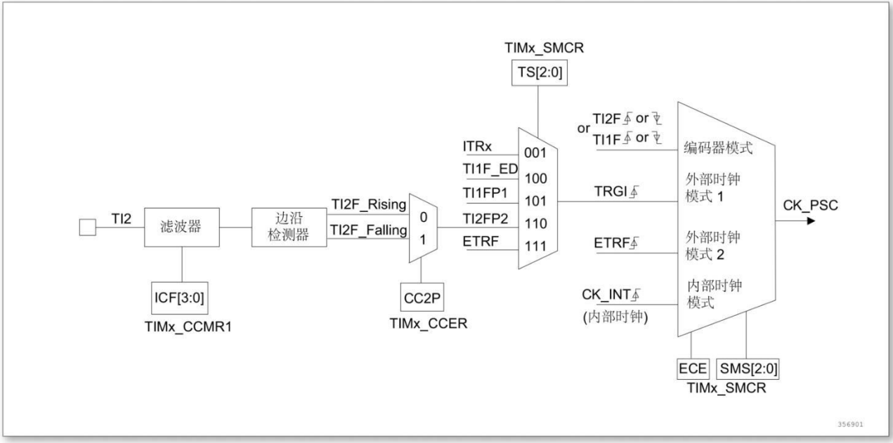
图 12-22 TI2 外部时钟连接例子
