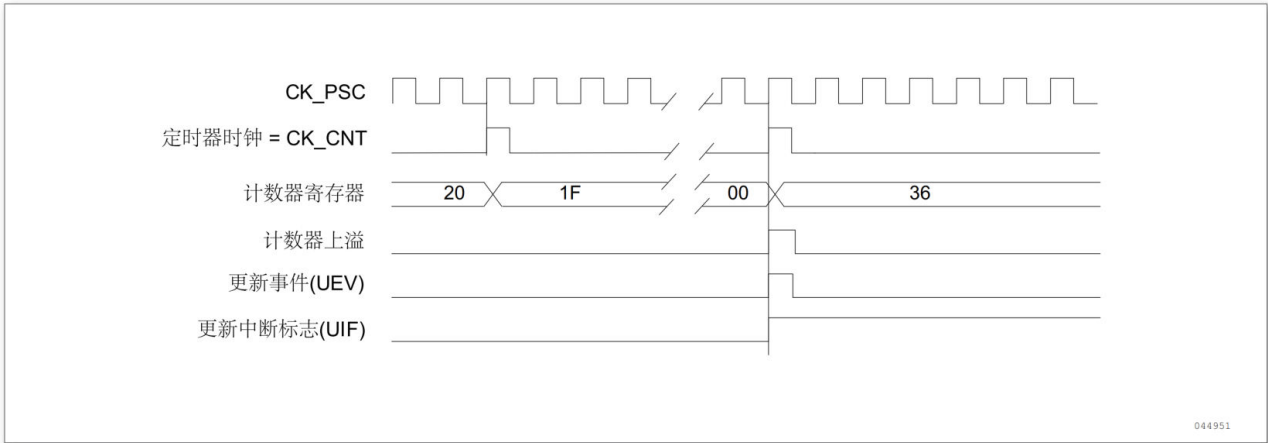
图 11-13 计数器时序图，内部时钟分频因子为 N
