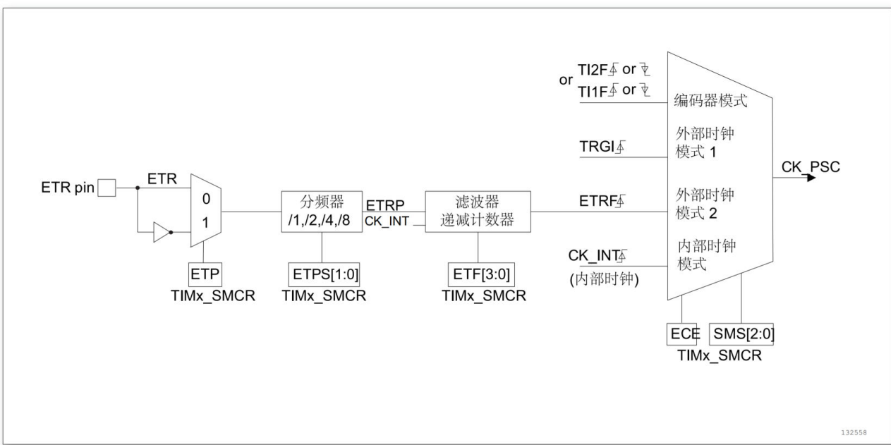
图 13-24 外部触发输入框图
