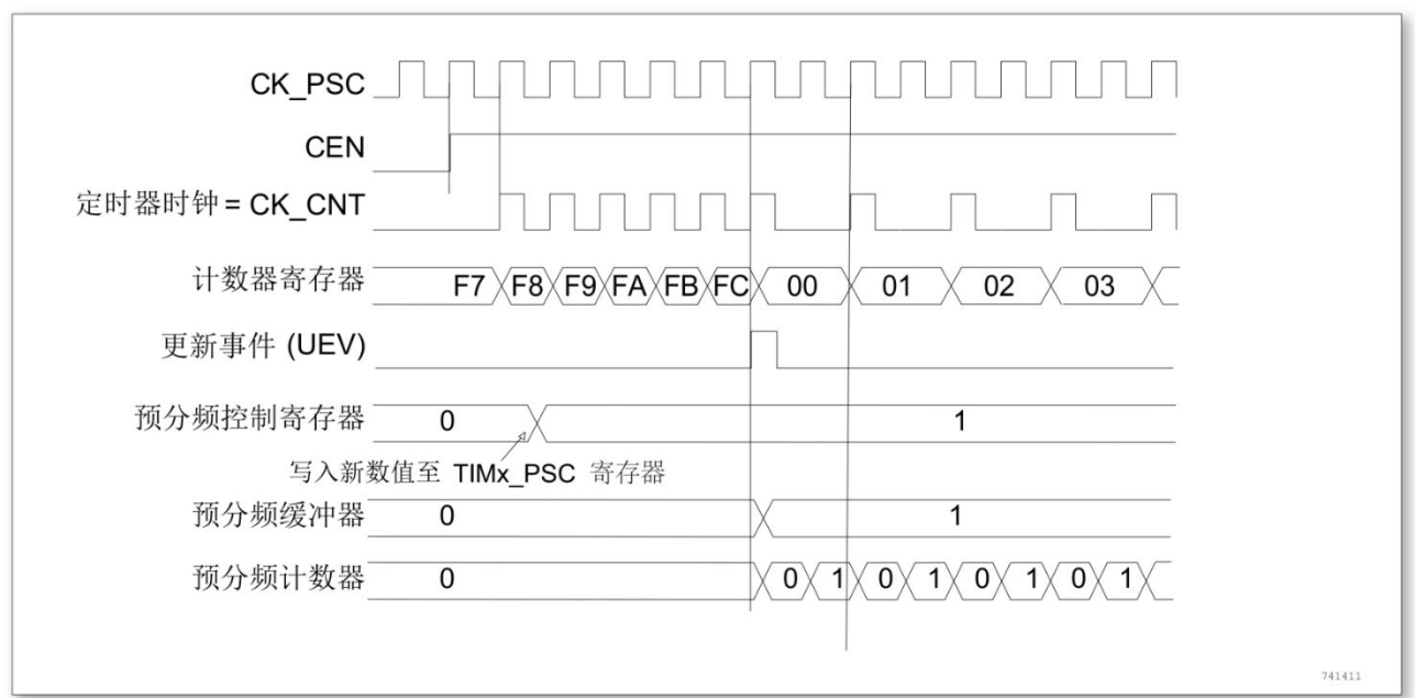
图 15-2 当预分频器的参数从 1 变到 2 时，计数器的时序图
