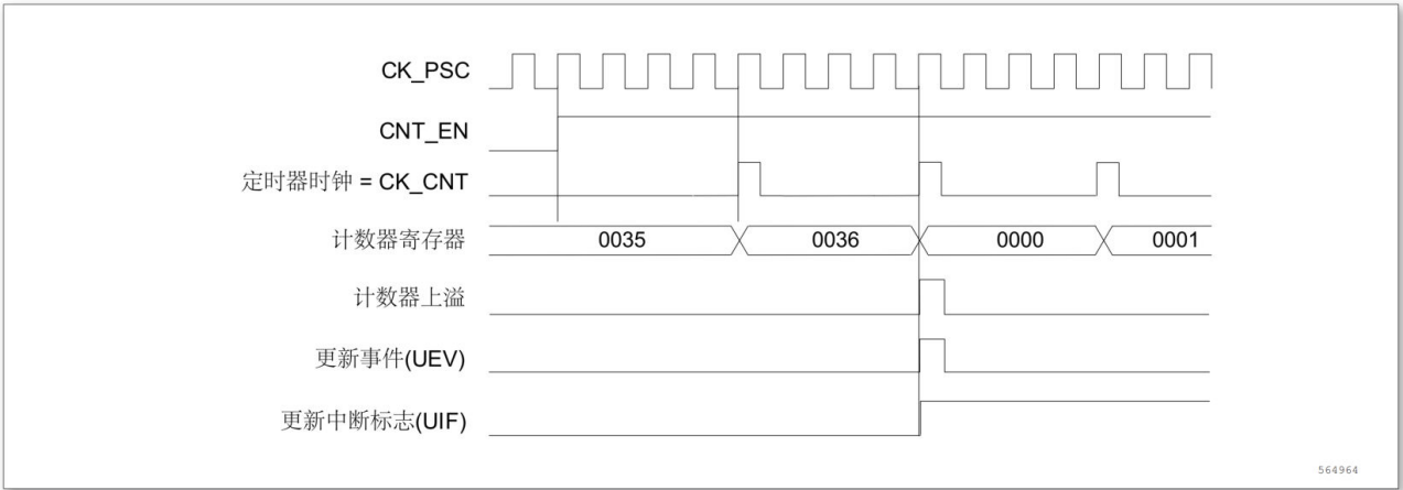
图 14-6 计数器时序图，内部时钟分频因子为 4
