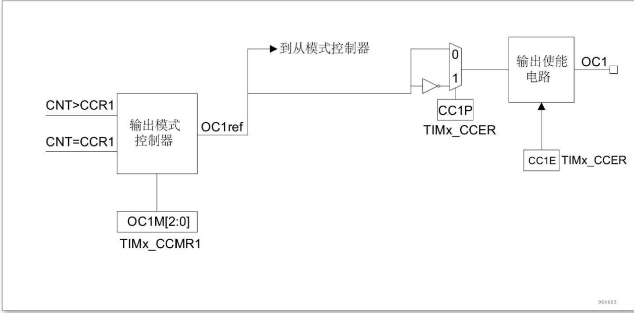
图 12-28 捕获/比较通道的输出部分 (通道 1)
