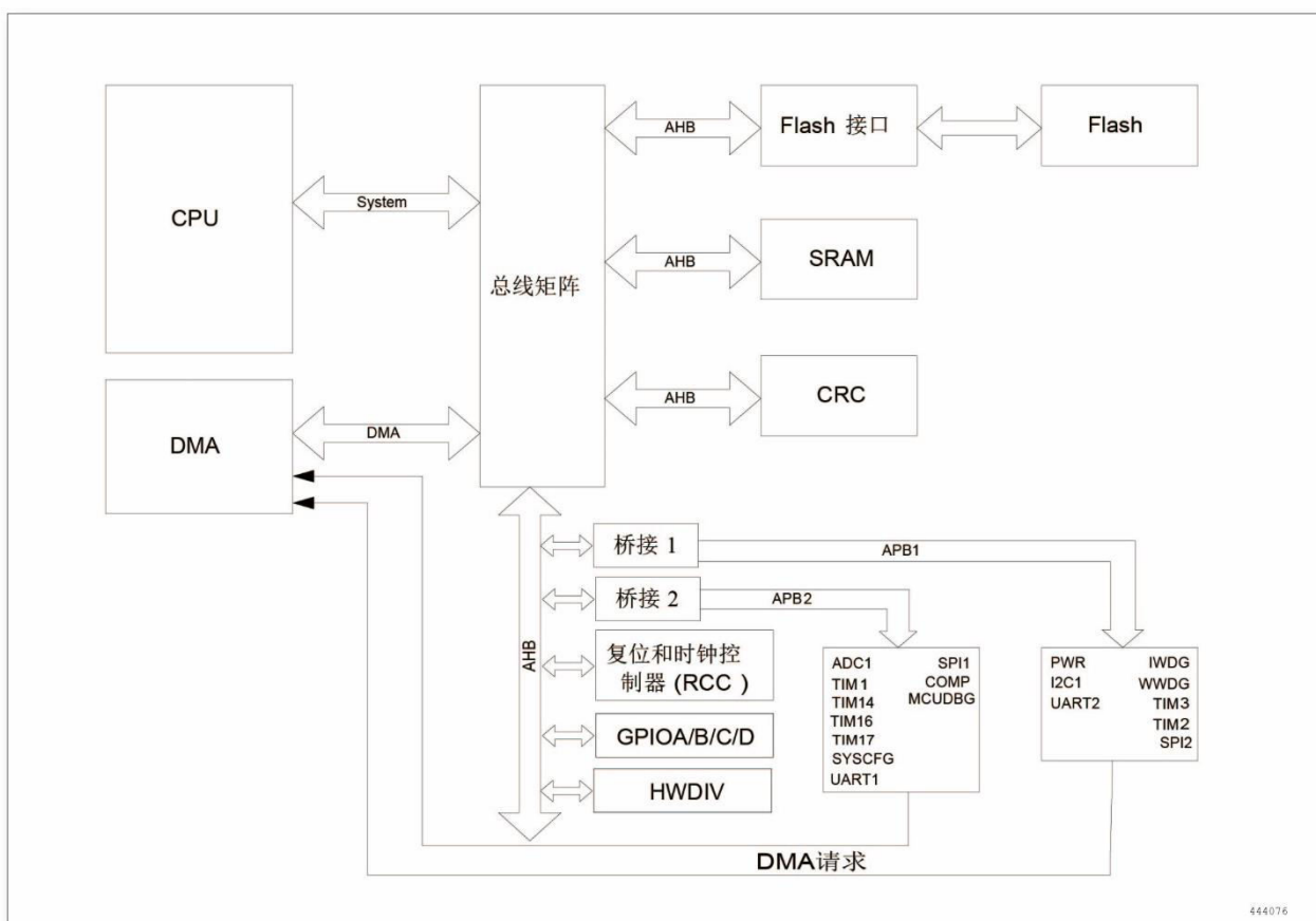
图 1-1 系统架构框图
