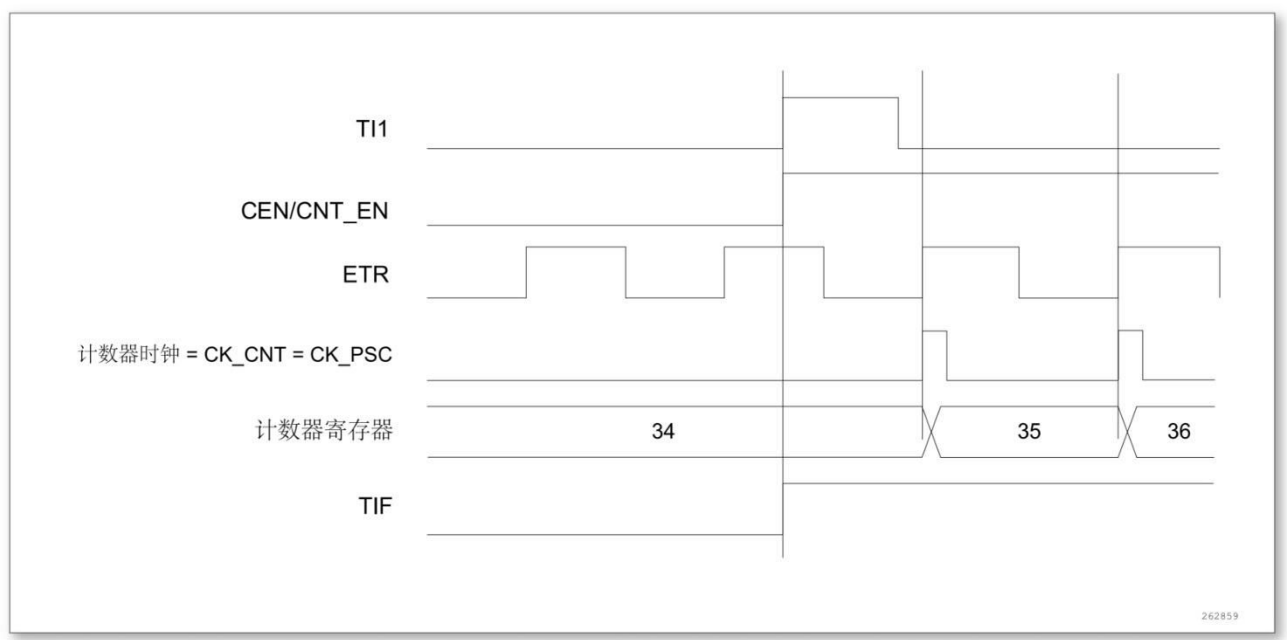
图 12-40 外部时钟模式 2 + 触发模式下的控制电路
