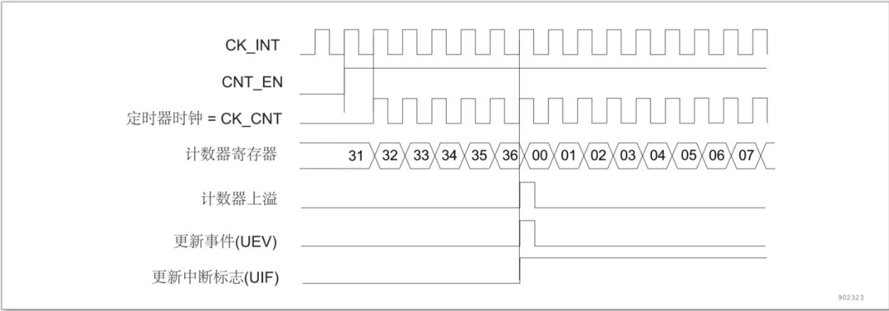
图 15-4 计数器时序图，内部时钟分频因子为 1
