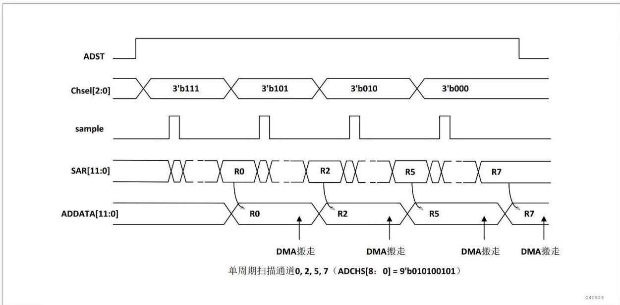
图 9-4 单周期扫描下使能通道转换时序图（通道方向从高到低）
