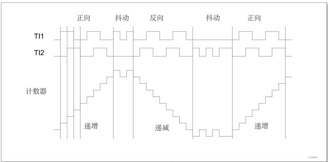
图 12-35 编码器模式下的计数器操作实例
