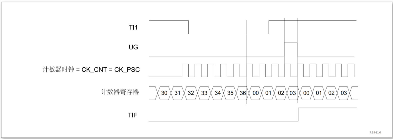
图 13-37 复位模式下的控制电路
