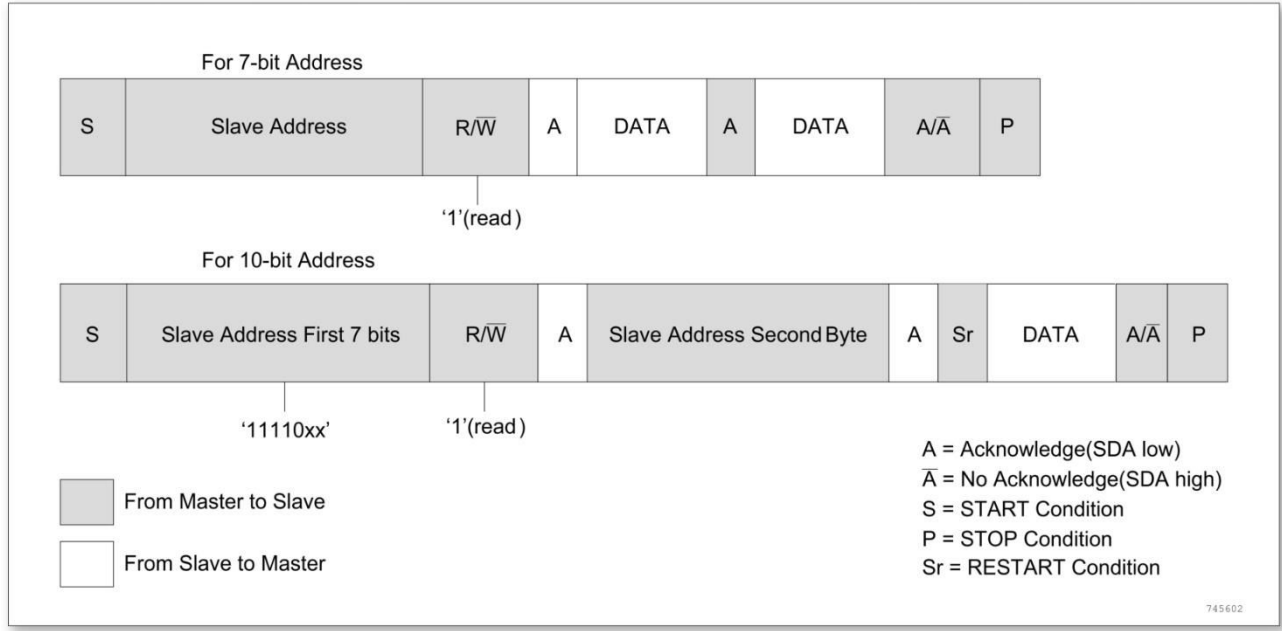
图 19-5 主接收协议
