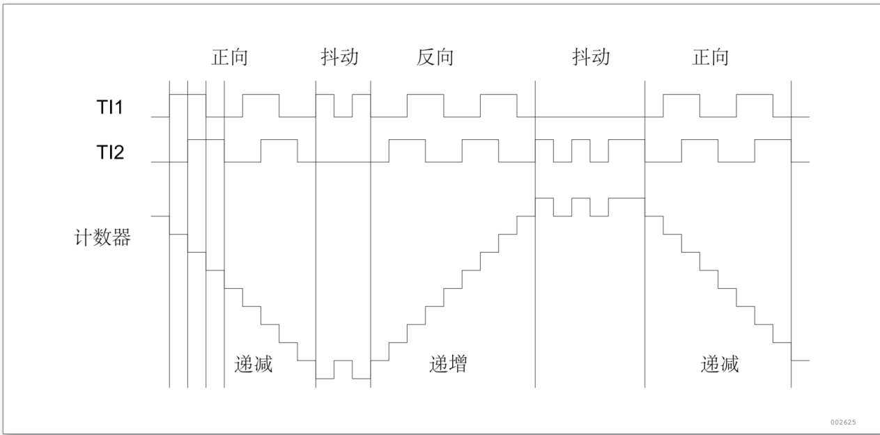
图 13-36 IC1FP1 反相的编码器接口模式示例
