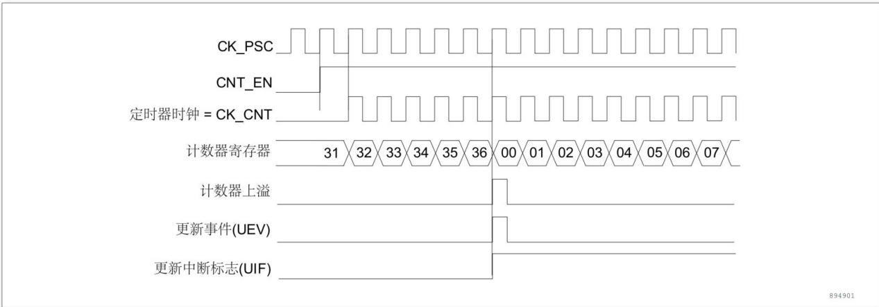
图 13-4 计数器时序图，内部时钟分频因子为 1
