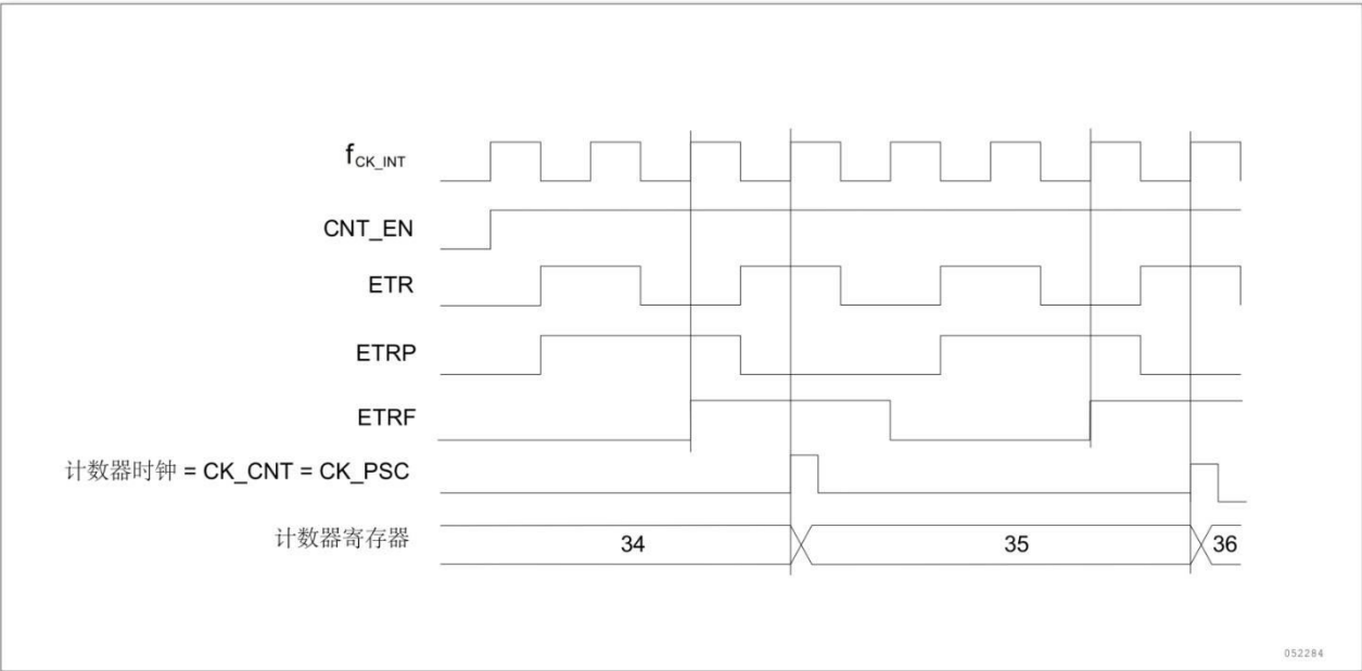
图 12-25 外部时钟模式 2 下的控制电路
