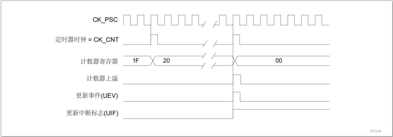
图 13-7 计数器时序图，内部时钟分频因子为 N
