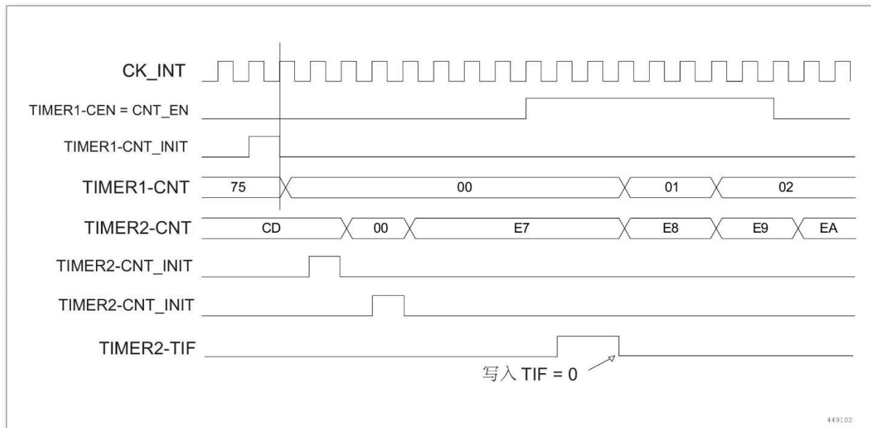
图 12-45 利用定时器 1 的使能触发定时器 2
