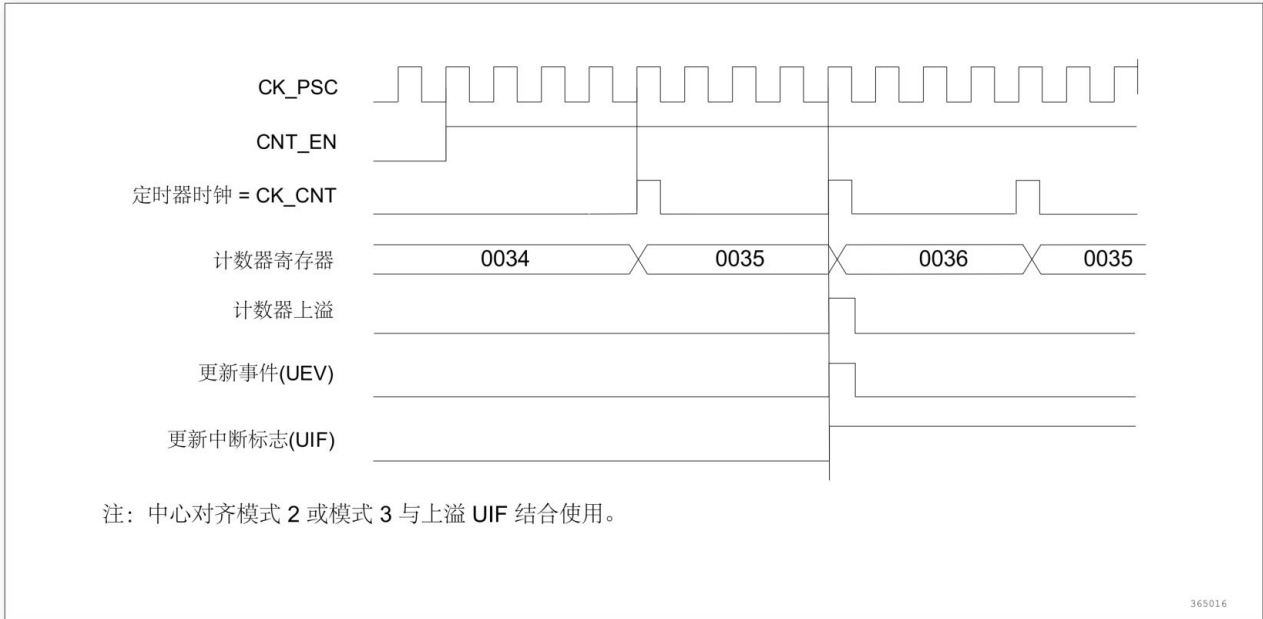
图 11-17 计数器时序图，内部时钟分频因子为 4，TIMx_ARR = 0x36
