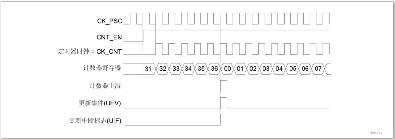
图 12-4 计数器时序图，内部时钟分频因子为 1
