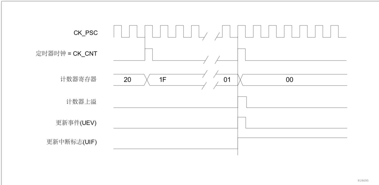
图 11-18 计数器时序图，内部时钟分频因子为 N
