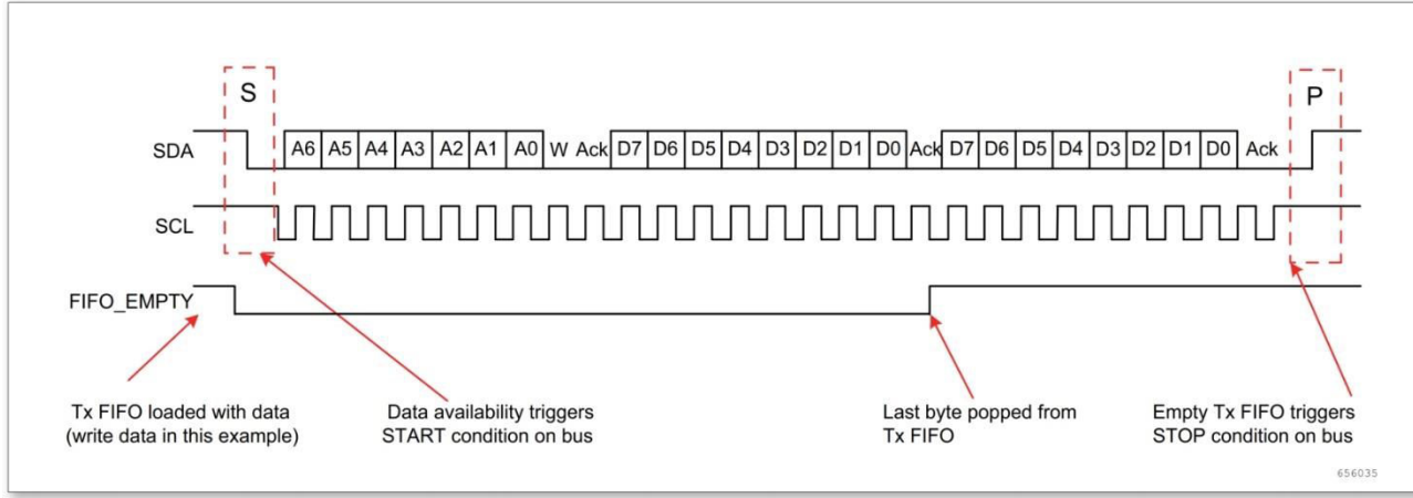
图 19-8 主发送 - Tx FIFO 为空
