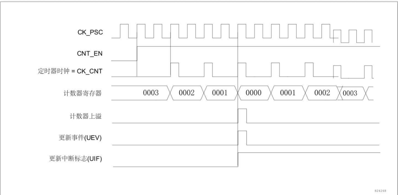
图 12-16 计数器时序图，内部时钟分频因子为 2
