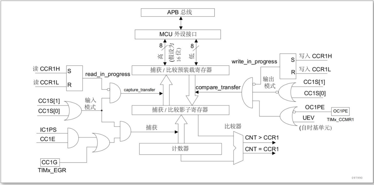
图 15-13 捕获/比较通道 1 的主电路
