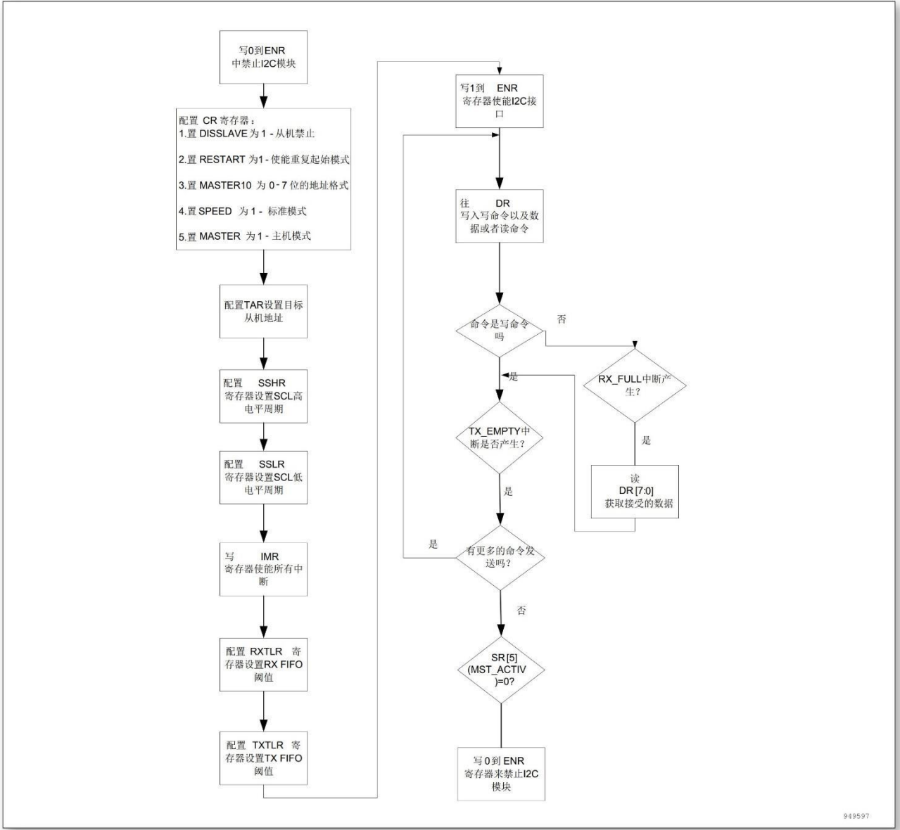
图 19-13 I2C 接口主机流程图
