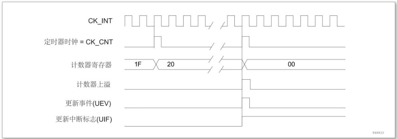
图 15-7 计数器时序图，内部时钟分频因子为 N
